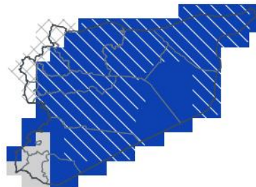
SON 2026 — échéance 1 mois 1-sur-46 humide · 100e centile
