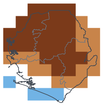
JJA 2026 — en saison 1-sur-15 sec · 4e centile
