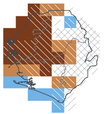
JAS 2026 — en saison 1-sur-8 sec · 11e centile
