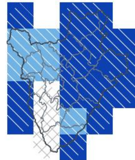
DJF 2026/27 — échéance 4 mois 1-sur-9 humide · 91e centile
