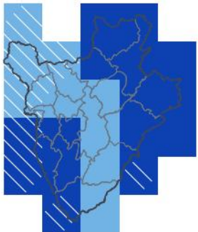
OND 2026 — échéance 2 mois 1-sur-12 humide · 93e centile
