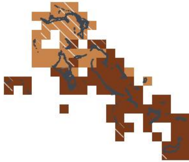
JAS 2026 — en saison 1-sur-12 sec · 7e centile
