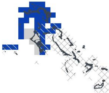
NDJ 2026/27 — échéance 3 mois 1-sur-46 humide · 100e centile
