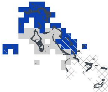
DJF 2026/27 — échéance 4 mois hors saison
