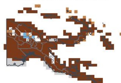
SON 2026 — échéance 1 mois 1-sur-46 sec · 0e centile
