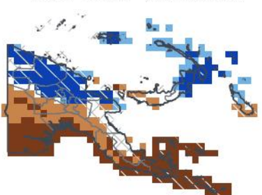
NDJ 2026/27 — échéance 3 mois 1-sur-4 sec · 24e centile
