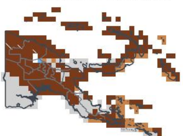
JAS 2026 — en saison 1-sur-46 sec · 0e centile
