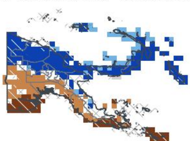
DJF 2026/27 — échéance 4 mois 1-sur-46 humide · 100e centile
