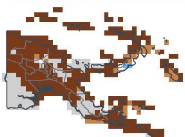
JJA 2026 — en saison 1-sur-46 sec · 0e centile
