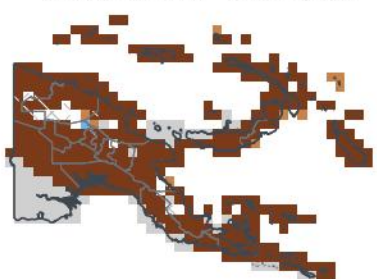
ASO 2026 — en saison 1-sur-46 sec · 0e centile
