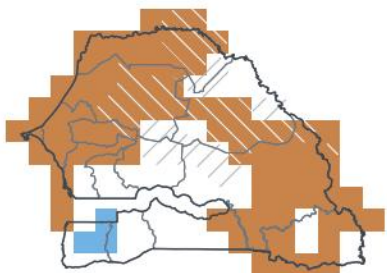
JJA 2026 — en saison 1-sur-3 sec · 33e centile
