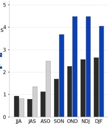
Précipitations moyennes du pays (mm/jour) noir = normale · couleur = prévision
