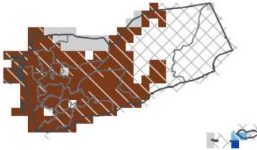
ASO 2026 — en saison 1-sur-46 sec · 0e centile
