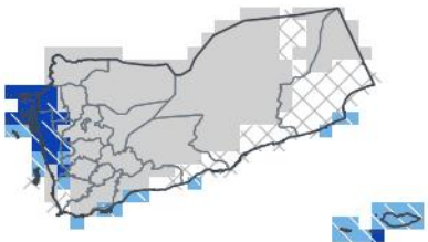
OND 2026 — échéance 2 mois hors saison
