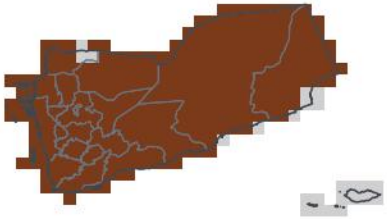
JJA 2026 — en saison 1-sur-46 sec · 0e centile
