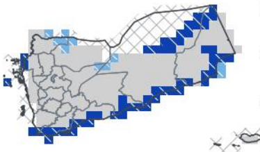
DJF 2026/27 — échéance 4 mois hors saison
