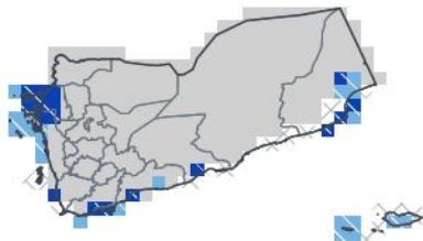
NDJ 2026/27 — échéance 3 mois hors saison
