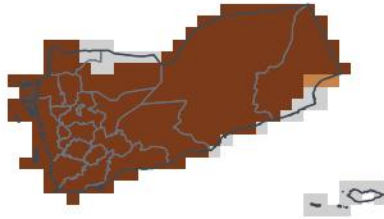
JAS 2026 — en saison 1-sur-46 sec · 0e centile
