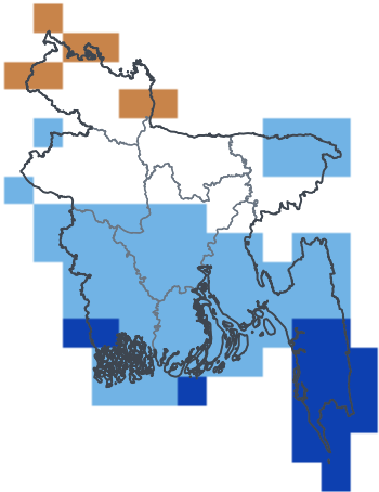
JJA 2026 — en saison 1-sur-4 humide · 73e centile
