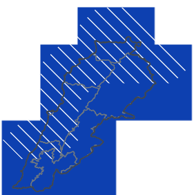
OND 2026 — échéance 2 mois 1-sur-46 humide · 100e centile
