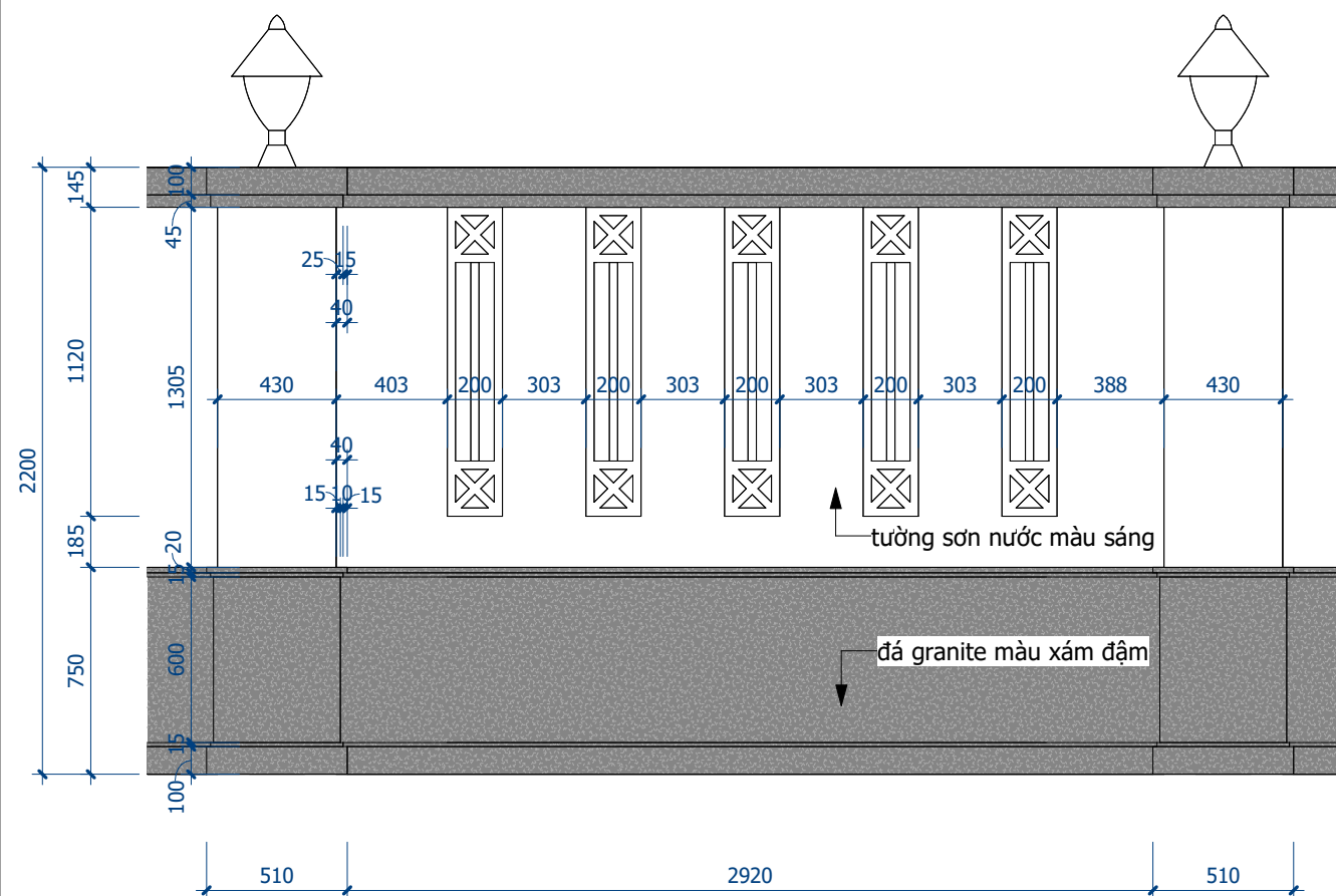
3 MẶT ĐỨNG TƯỜNG RÀO CHÍNH 1 : 25
