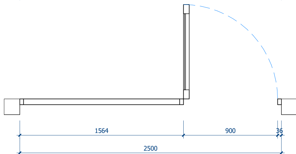
CỬA D8 1 : 20
