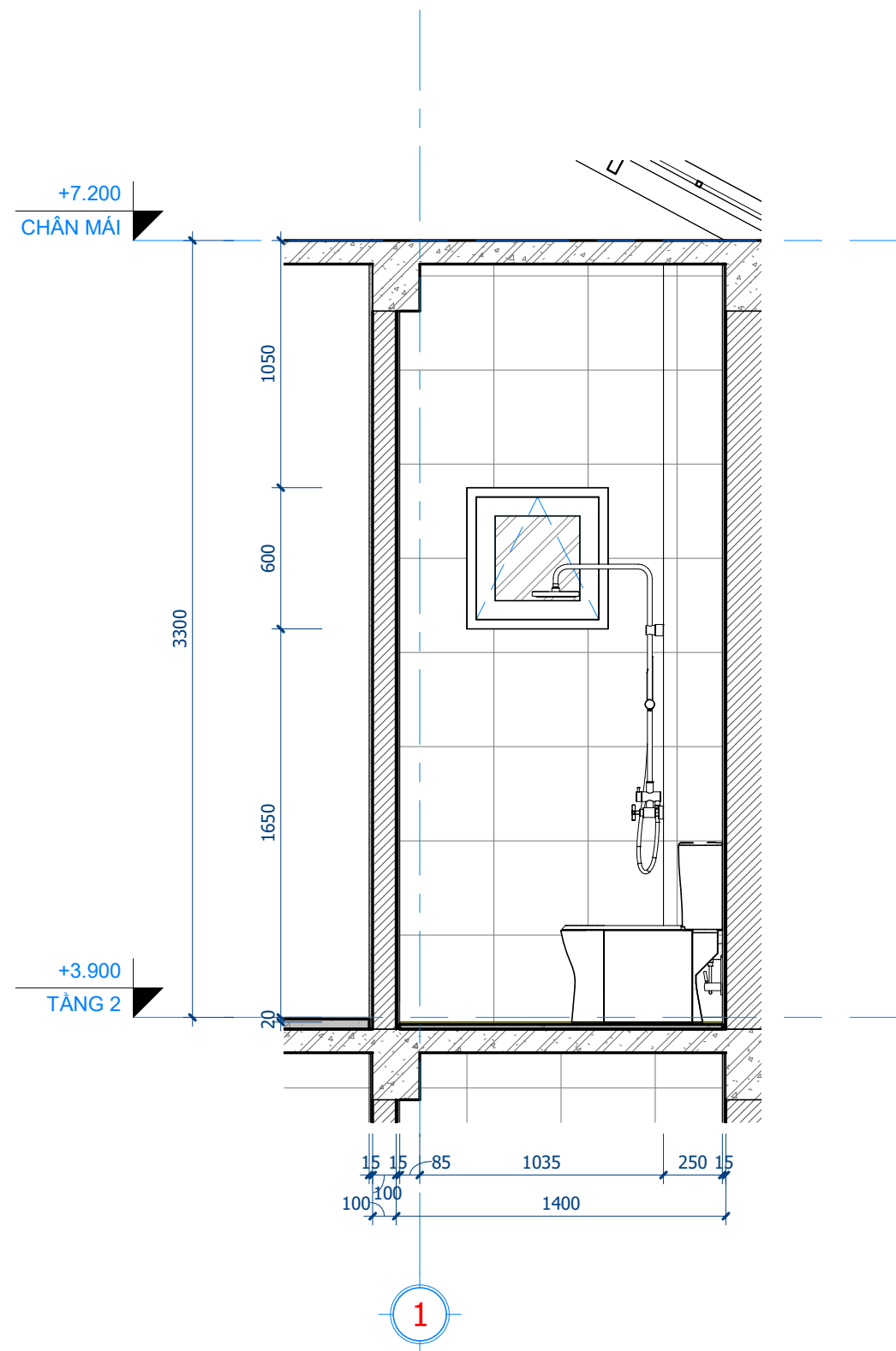
2 VS2- MẶT CẮT 2-2 1 : 25
