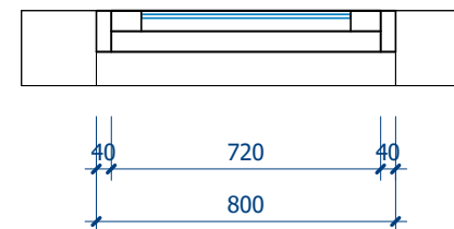
○ CỬA S5 1 : 20
