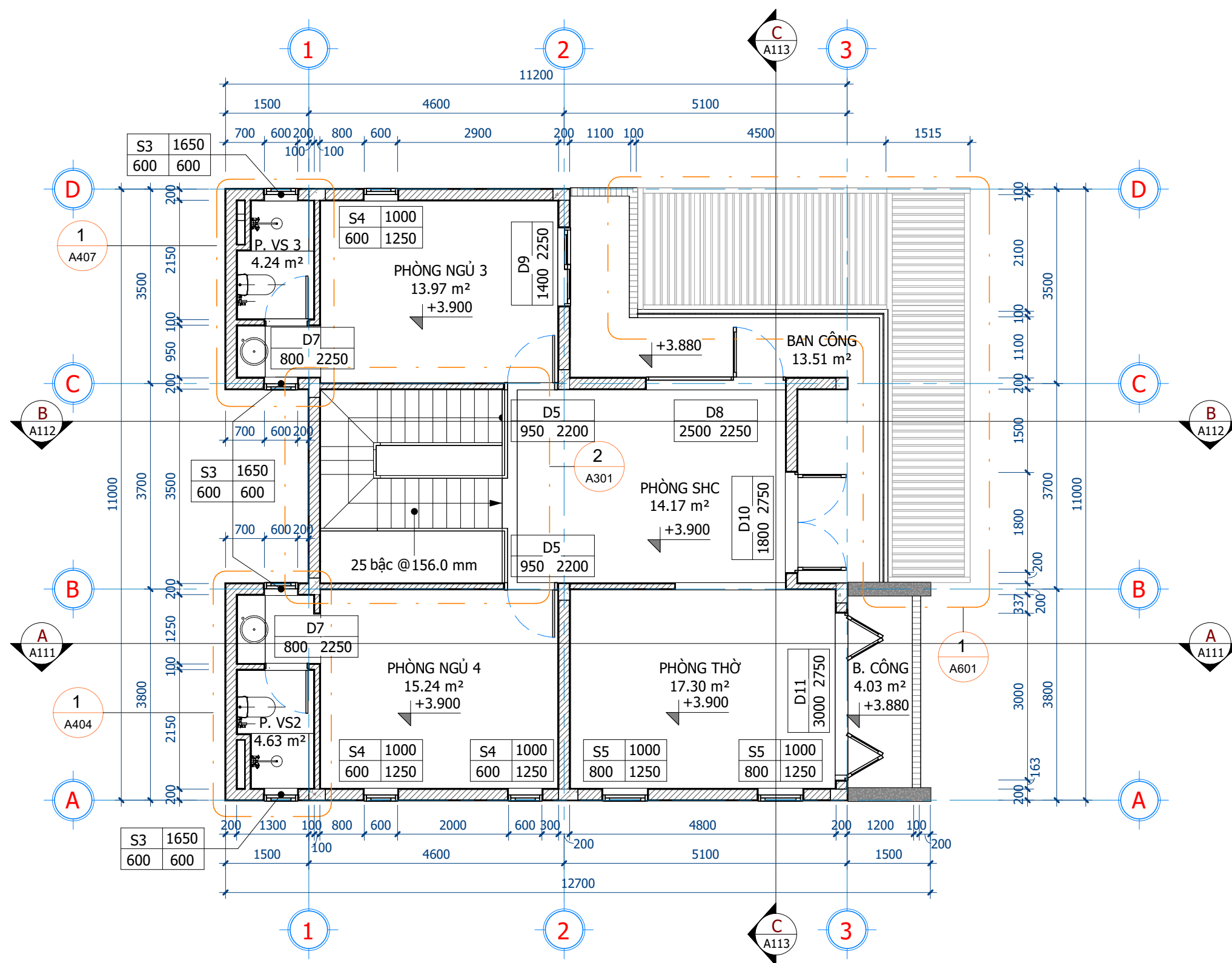
1 MẶT BẰNG KÍCH THƯỚC TẦNG 2 1 : 75
