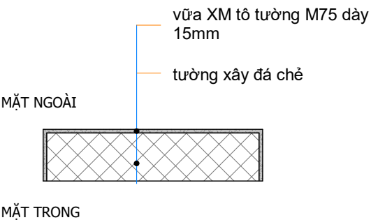
TƯỜNG T15 1 : 20
