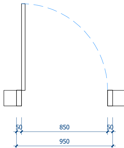
○ CỬA D5 1 : 20
