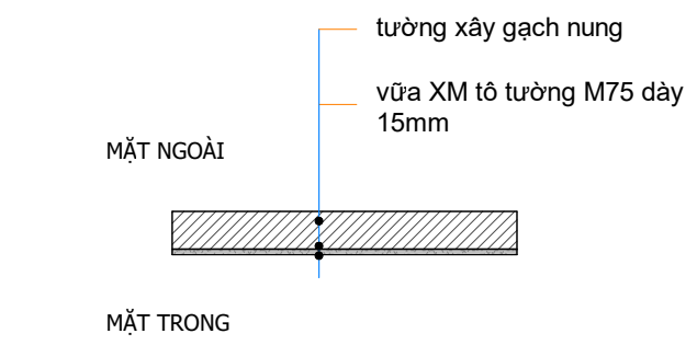
TƯỜNG T4 1 : 20
