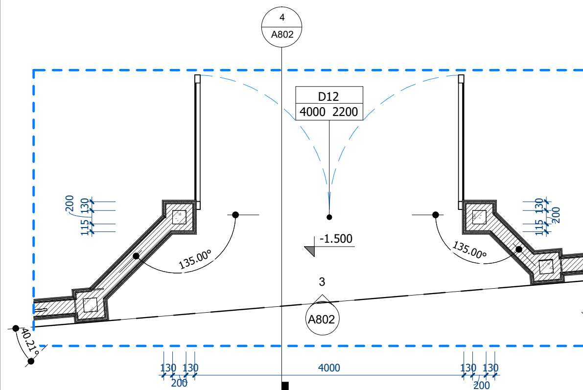
1 MẶT BẰNG CỔNG CHÍNH 1 : 50
