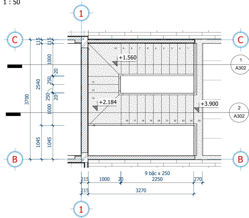
2 MB CẦU THANG TẦNG 2 1 : 50
