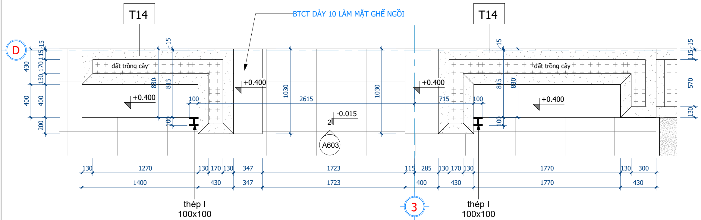
1 BỒN HOA- MẶT BẰNG CHI TIẾT 1 : 25
