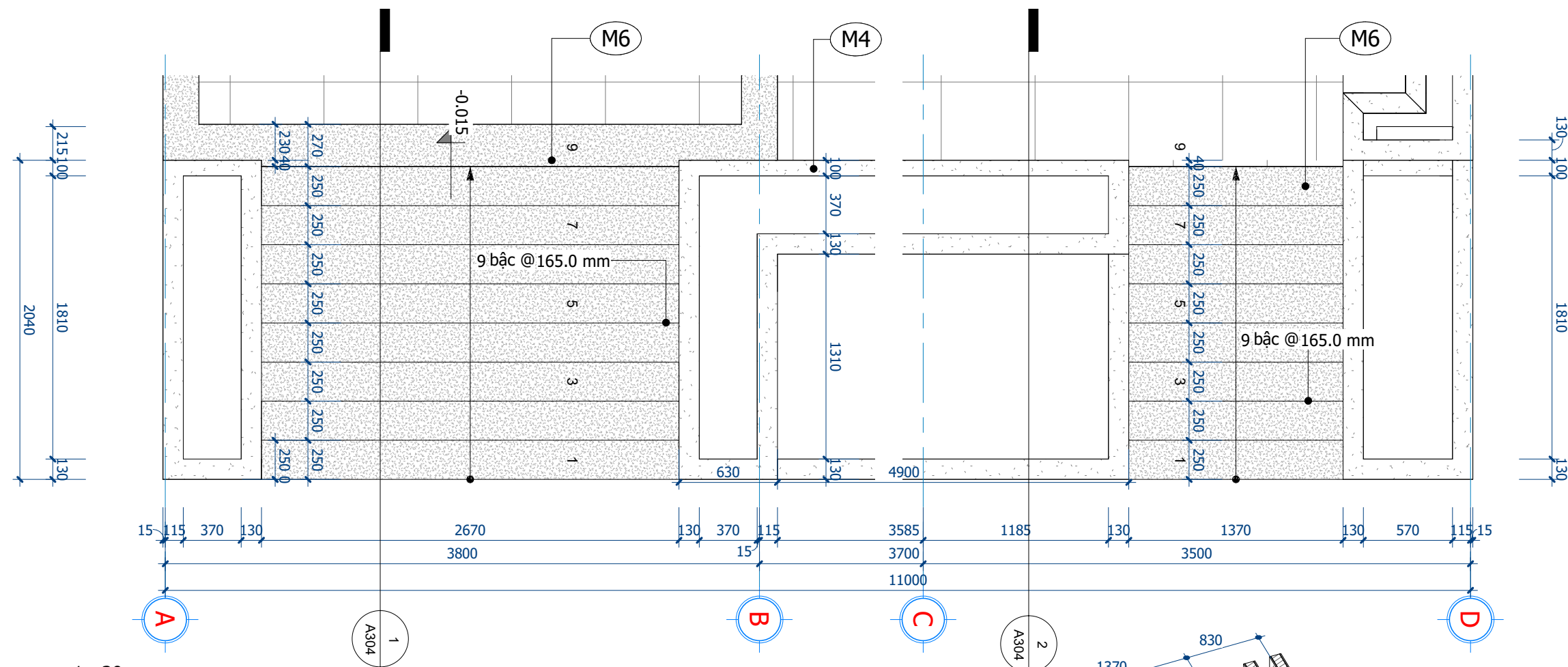
1 : 30 BẬC CẤP 01- MẶT BẰNG CHI TIẾT
