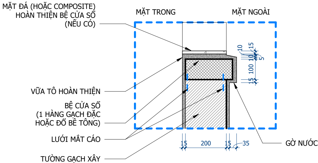
CẤU TẠO ĐẦU CỬA-BÊ CỬA 1 : 10
