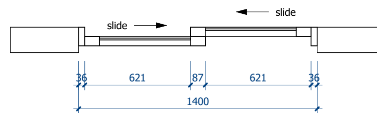
CỬA D4 1 : 20
