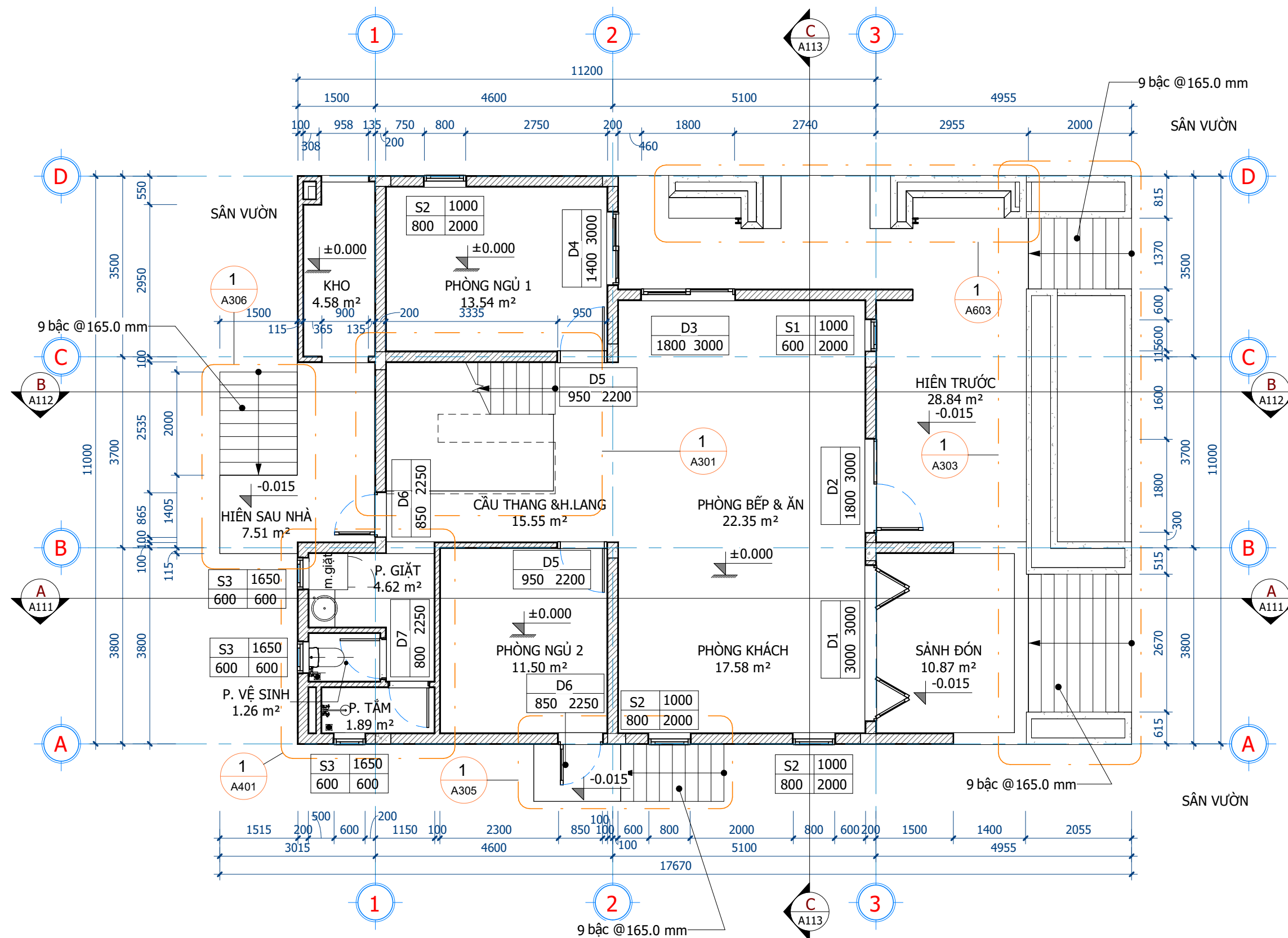
1 MẶT BẰNG KÍCH THƯỚC TẦNG 1 1 : 75
