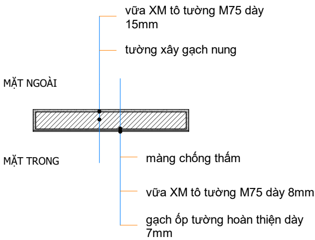
TƯỜNG T15 1 : 20
