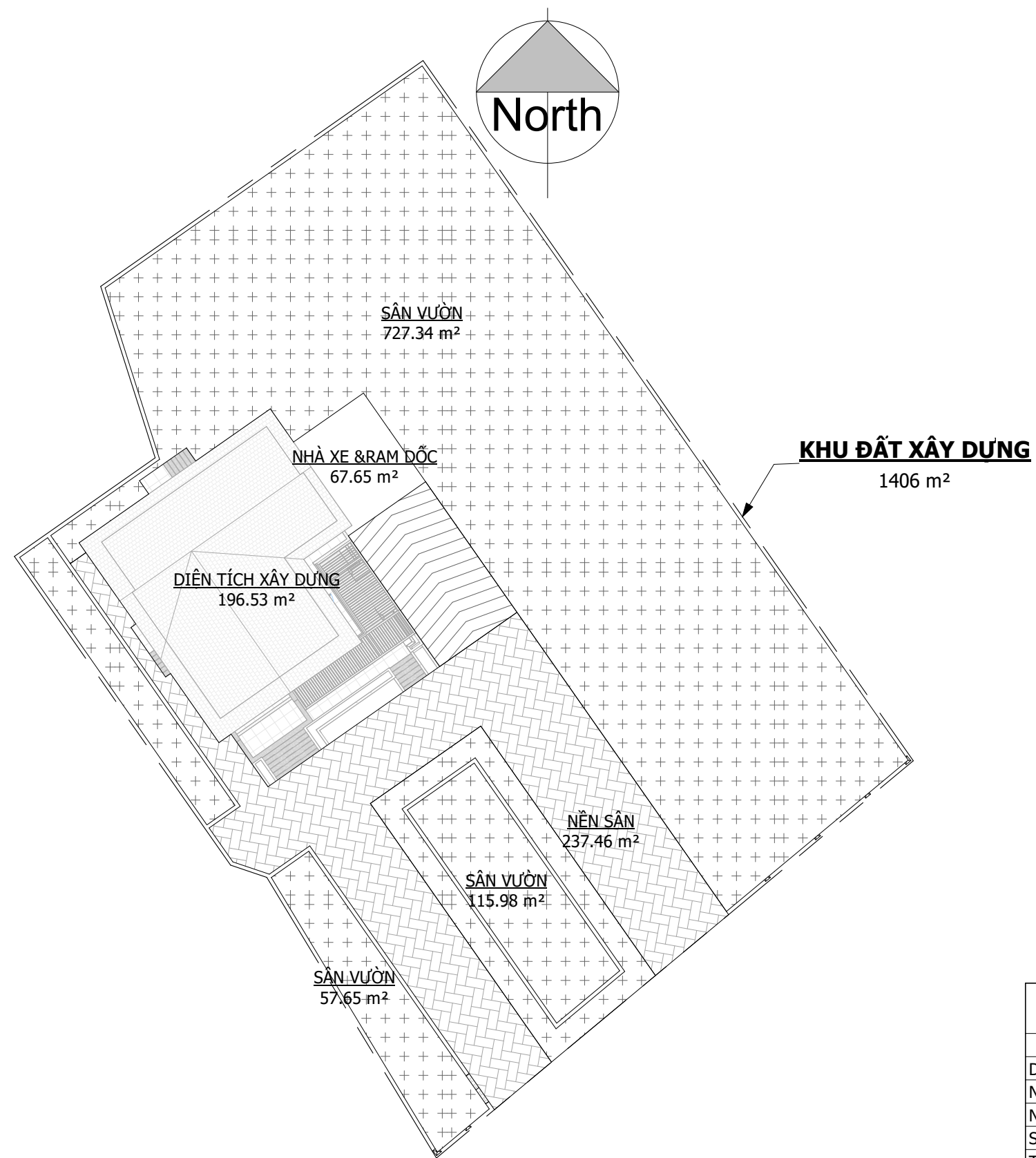
1 MẶT BẰNG TỔNG THỂ 1 : 250
