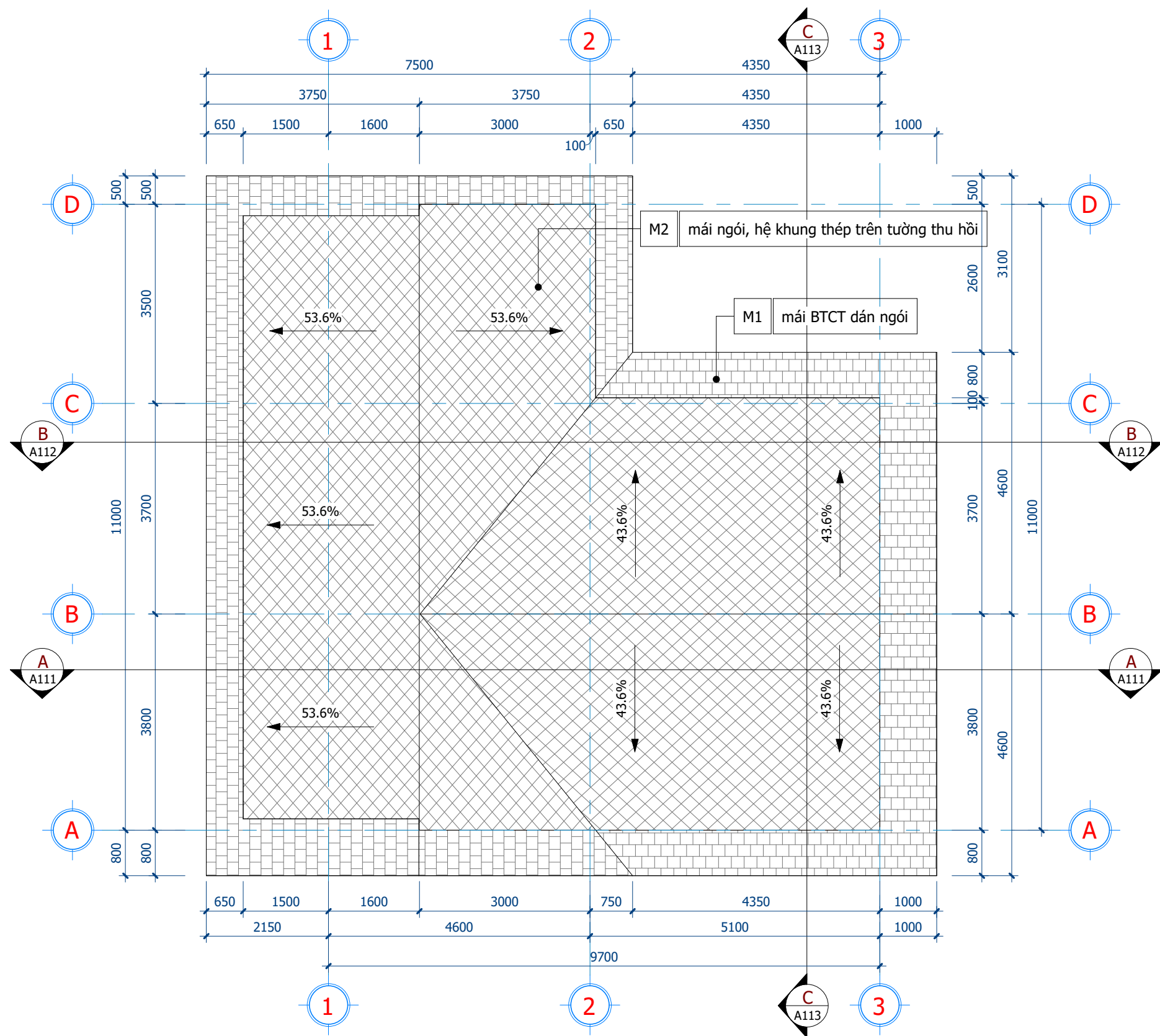
1 MẶT BẰNG KÍCH THƯỚC MÁI 1 : 75
