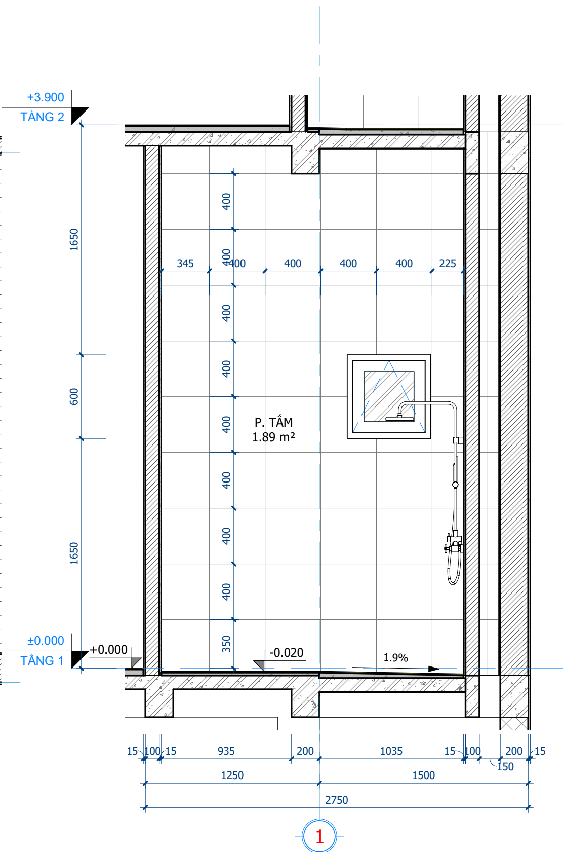
2 VS1- MẶT CẮT 2-2 1 : 25
