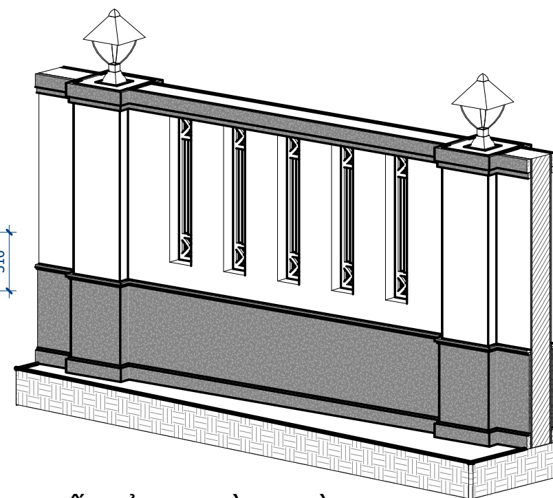
2 PHỐI CẢNH TƯỜNG RÀO
