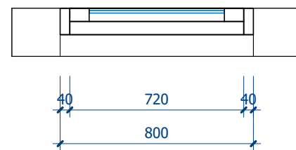
○ CỬA S2 1 : 20
