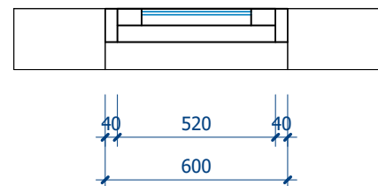
○ CỬA S4 1 : 20
