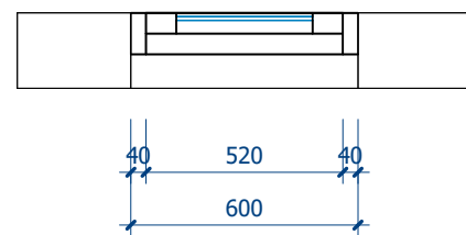
○ CỬA S1 1 : 20
