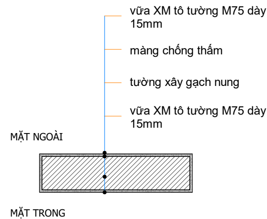
TƯỜNG T1&T3 1 : 20
