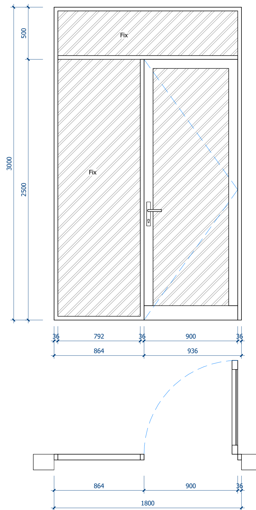
CỬA D2 1 : 20
