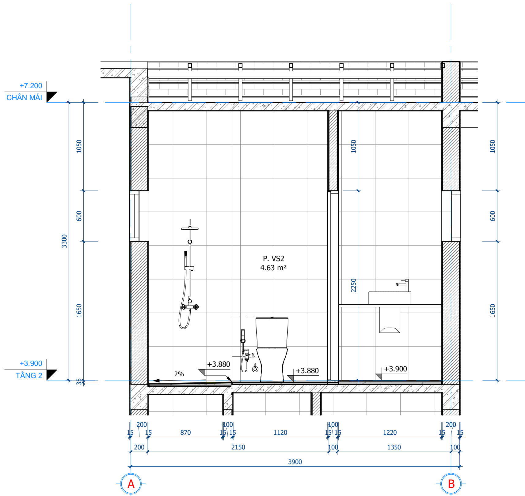
1 VS2- MẶT CẮT 1-1 1 : 25
