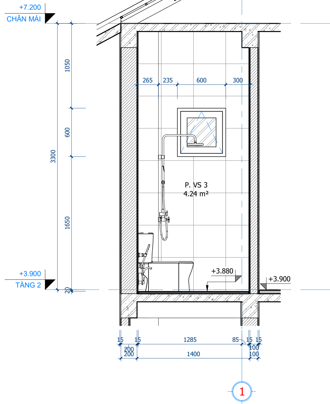
2 VS3- MẶT CẮT 2-2 1 : 25
