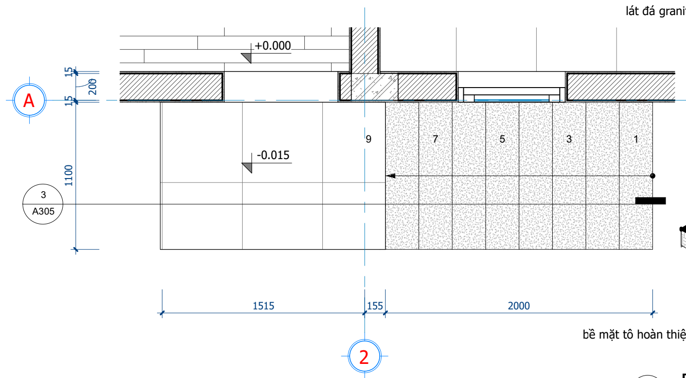
1 BẬC CẤP 02- MẶT BẰNG CHI TIẾT 1 : 25
