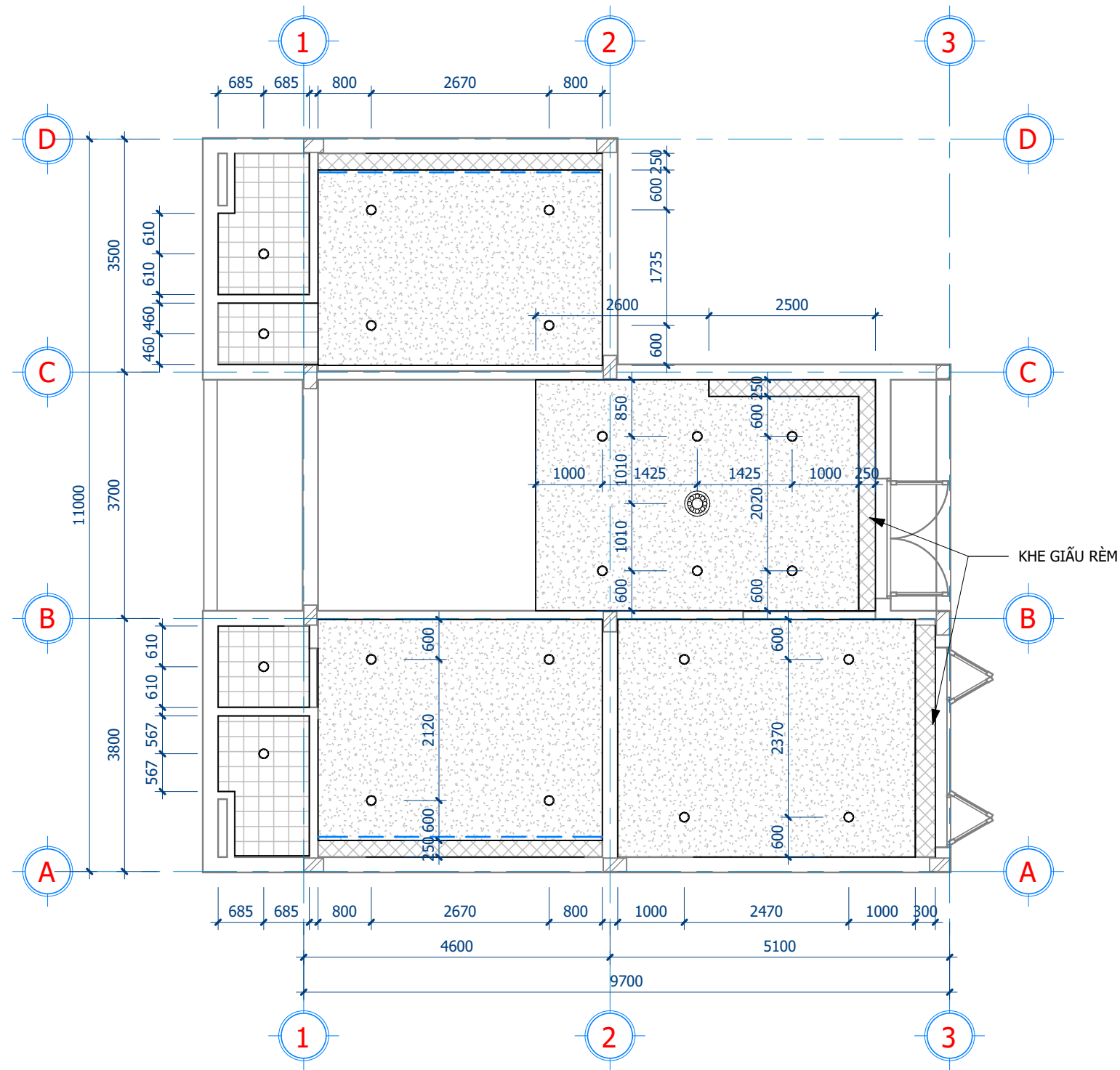
1 MẶT BẰNG TRẦN TẦNG 2 1 : 75
