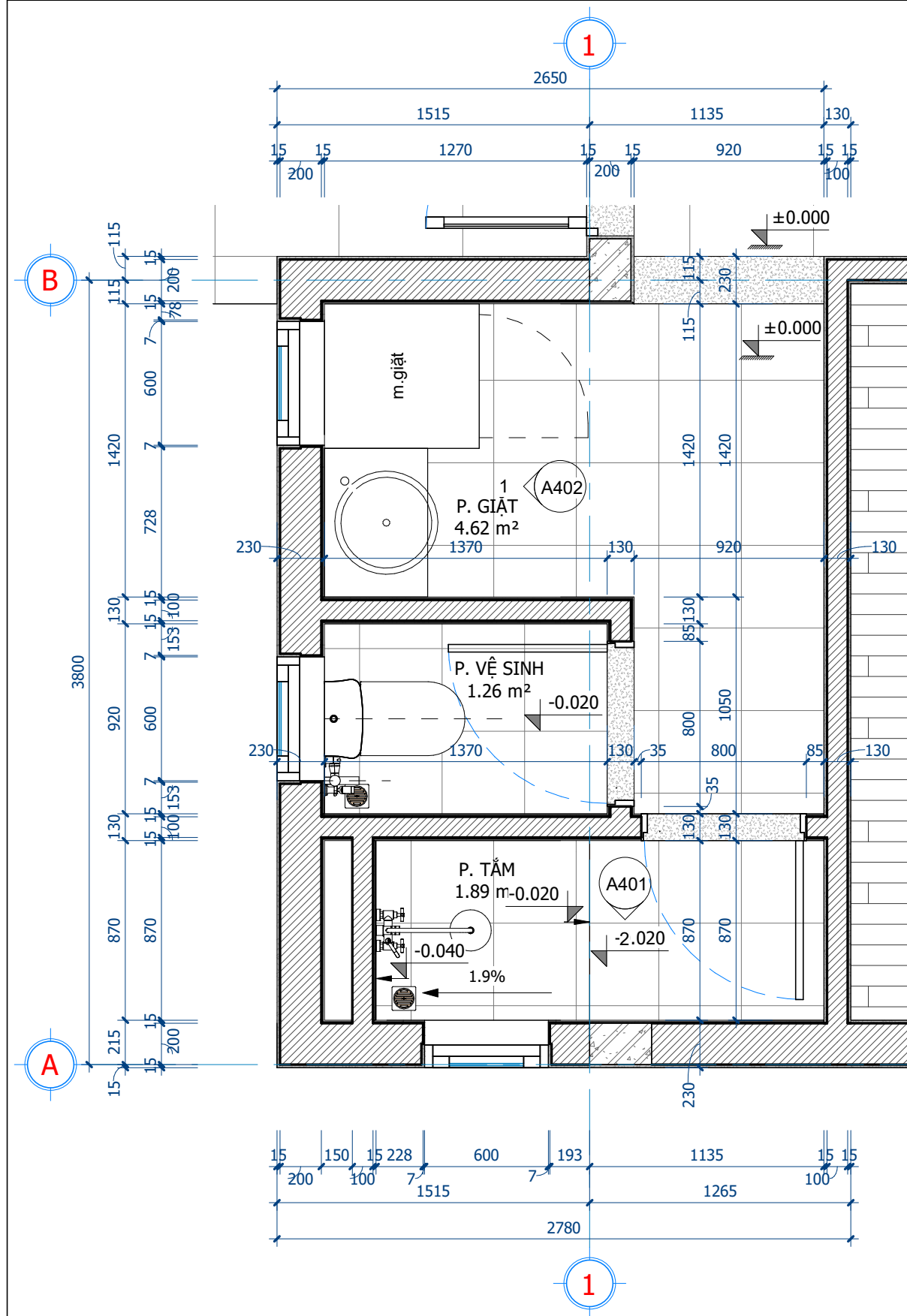
1 MẶT BẰNG PHÒNG VS 1 1 : 25
