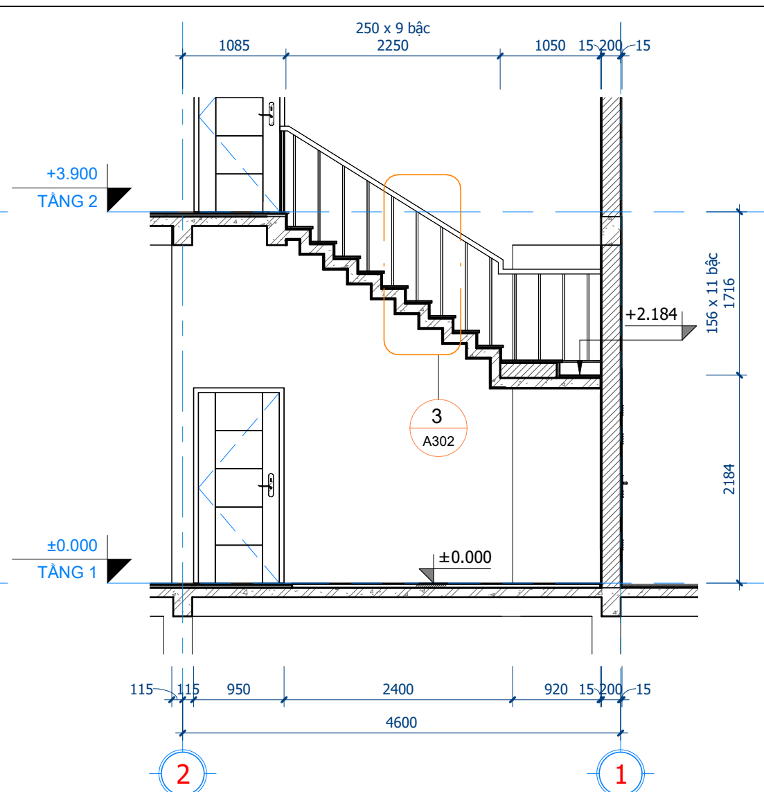
2 MẶT CẮT 2-2 1 : 50
