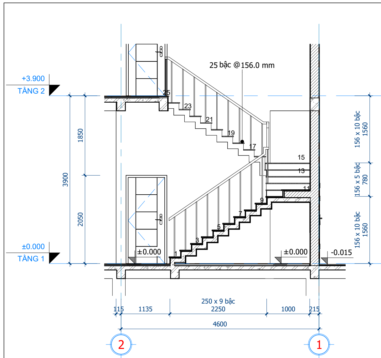
1 MẶT CẮT 1-1 1 : 50
