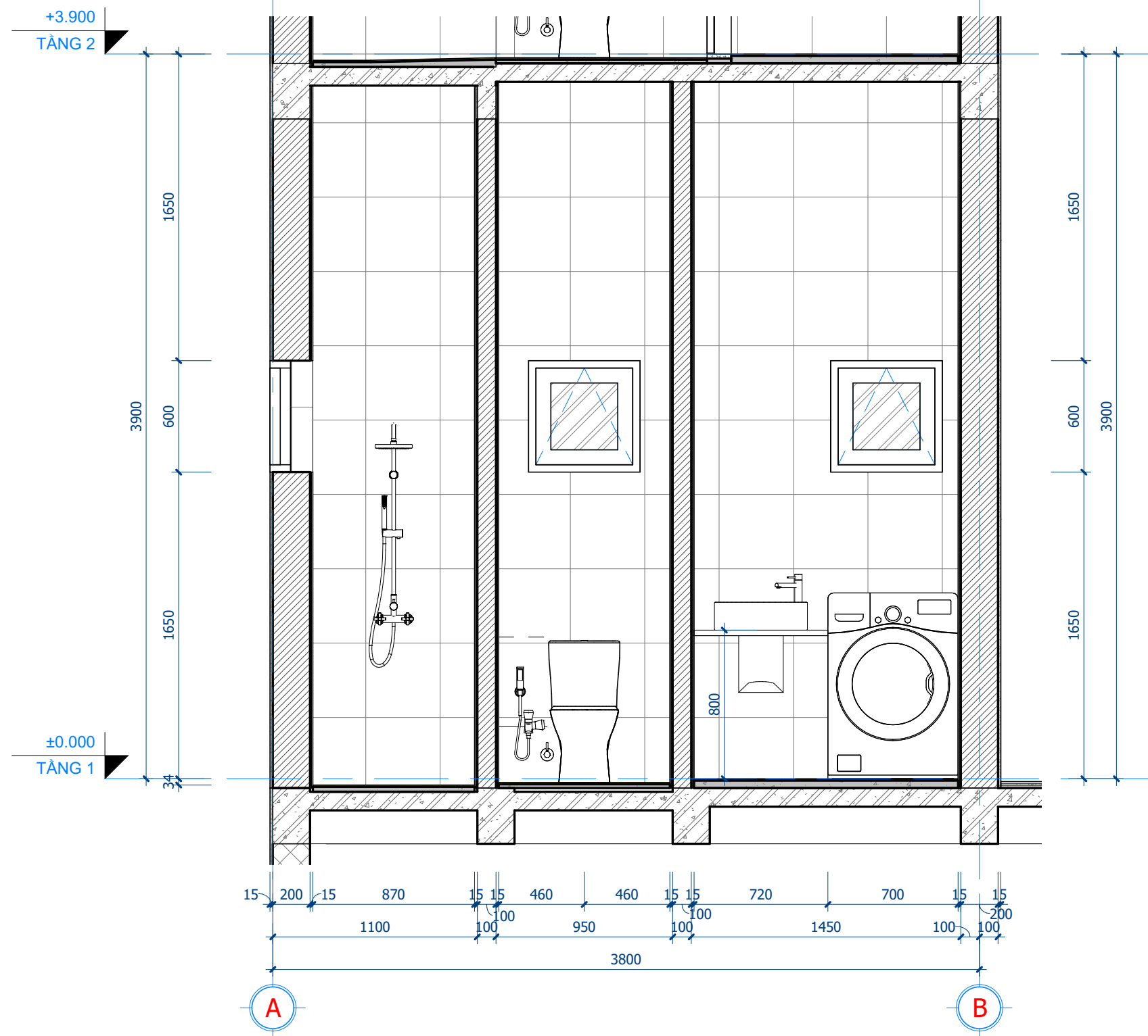
1 VS1-MẶT CẮT 1-1 1 : 25
