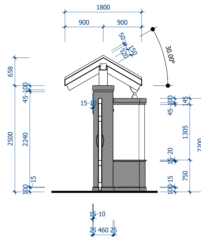
4 MC CỔNG CHÍNH 1 : 50
