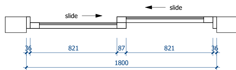
CỬA D3 1 : 20
