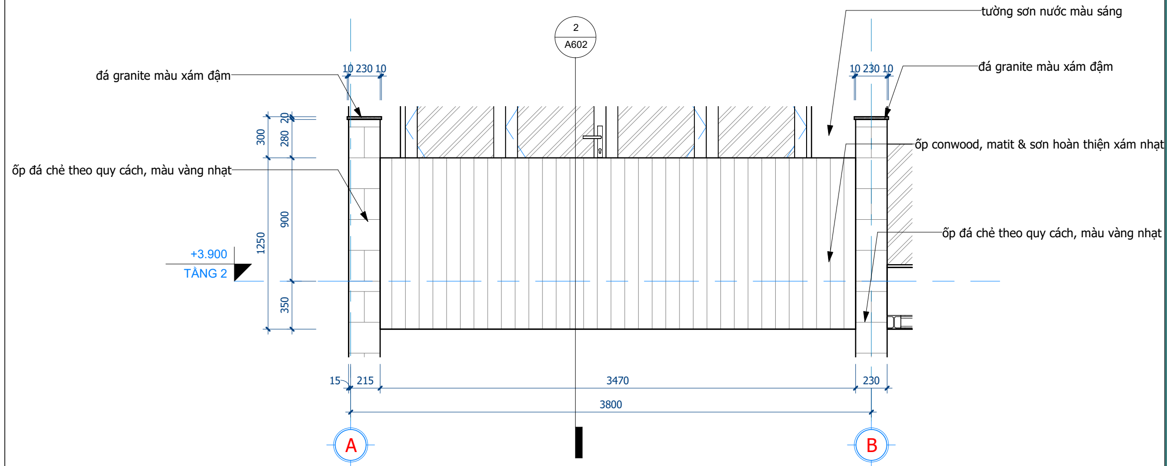
1 CHI TIẾT LAN CAN 01 1 : 25
