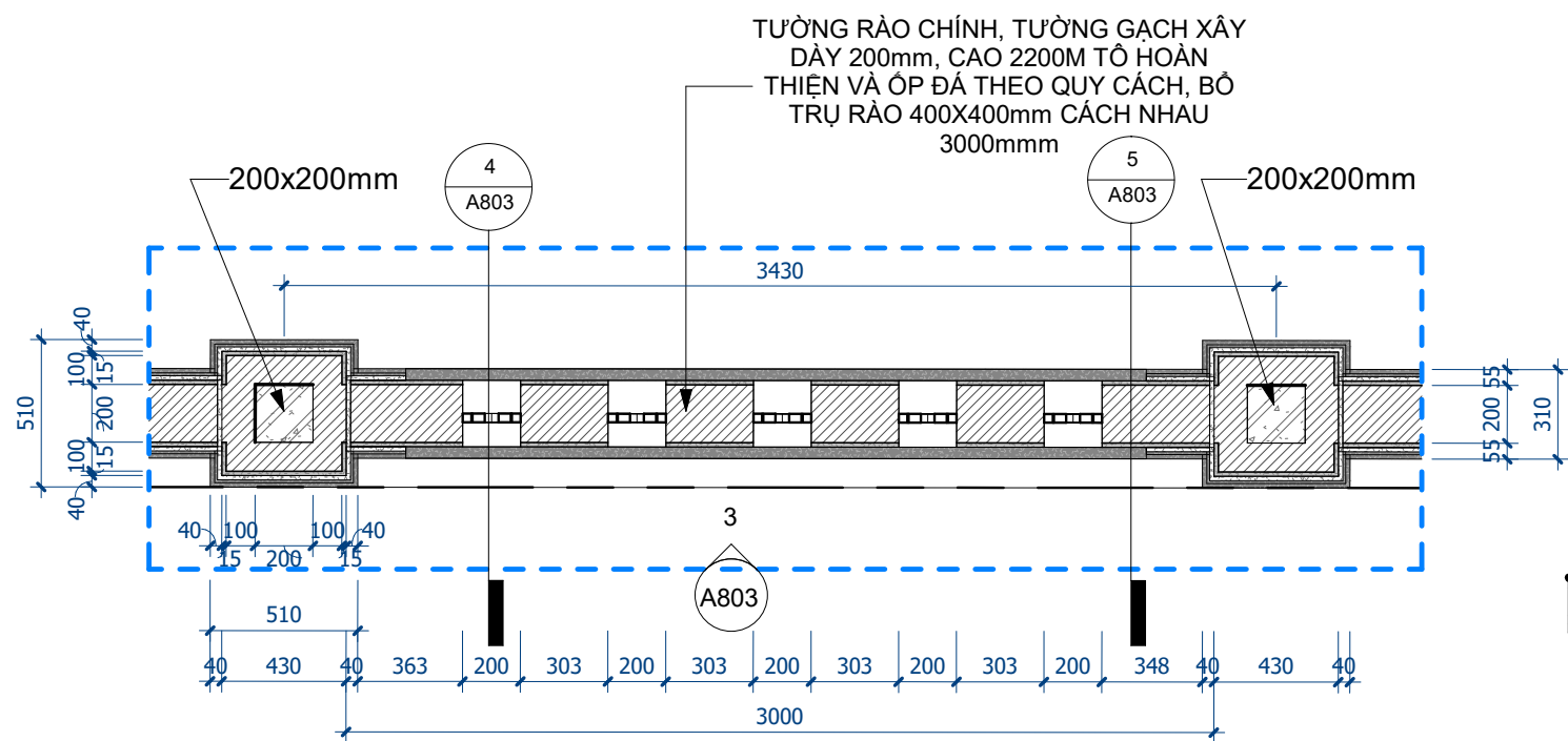
1 MB TRÍCH ĐOẠN HÀNG RÀO CHÍNH 1 : 25
