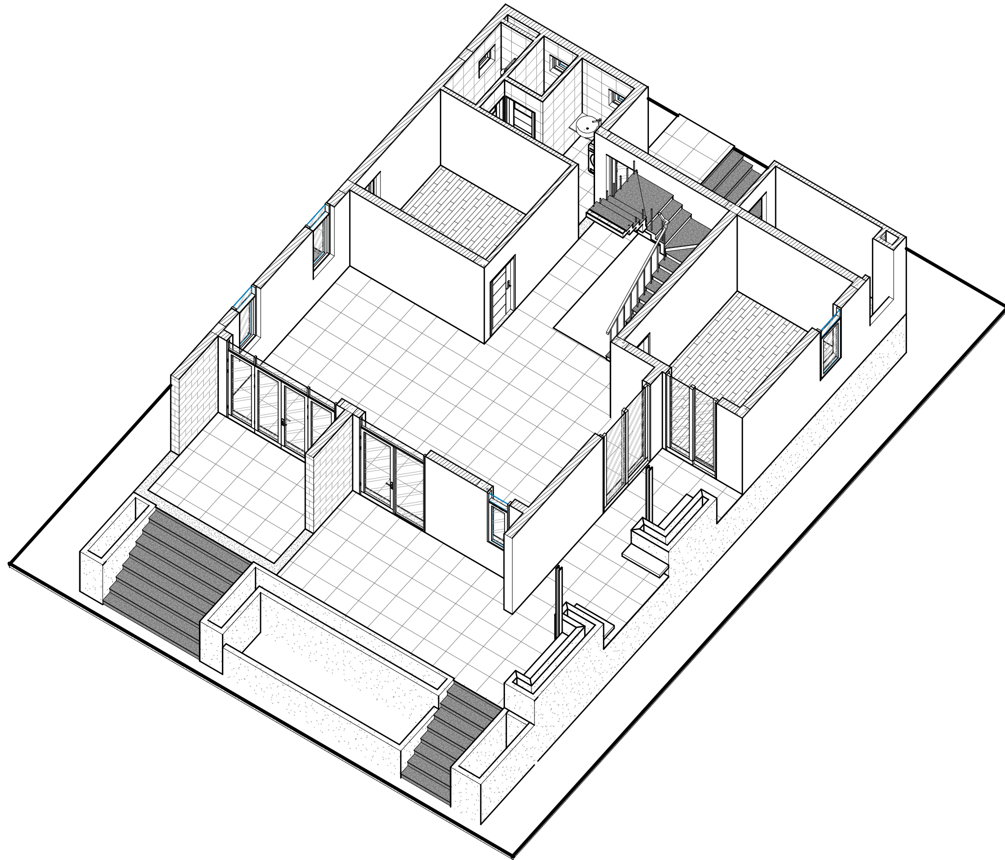
1 PHỐI CẢNH TẦNG 1
