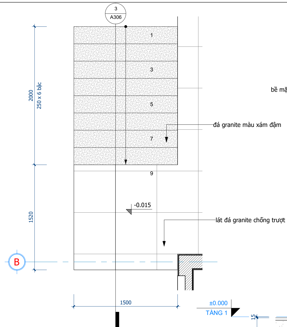
1 BẬC CẤP 03-MẶT BẰNG CHI TIẾT 1 : 25
