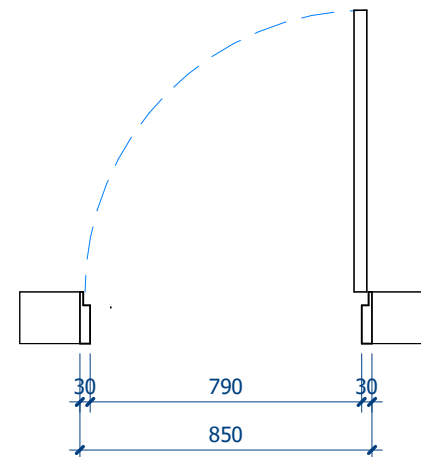
○ CỬA D7 1 : 20
