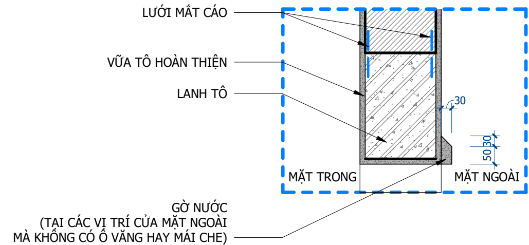
CẤU TẠO ĐẦU CỬA-BÊ CỬA 1 : 10
