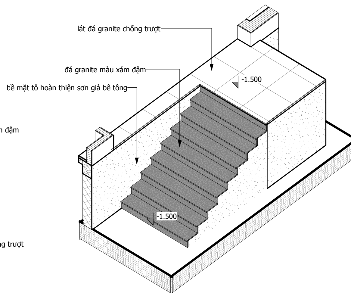
2 PHỐI CẢNH BẬC CẤP 03
