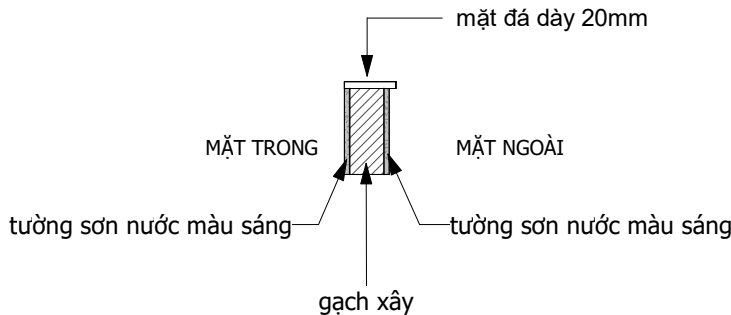
TƯỜNG T12 1 : 20
