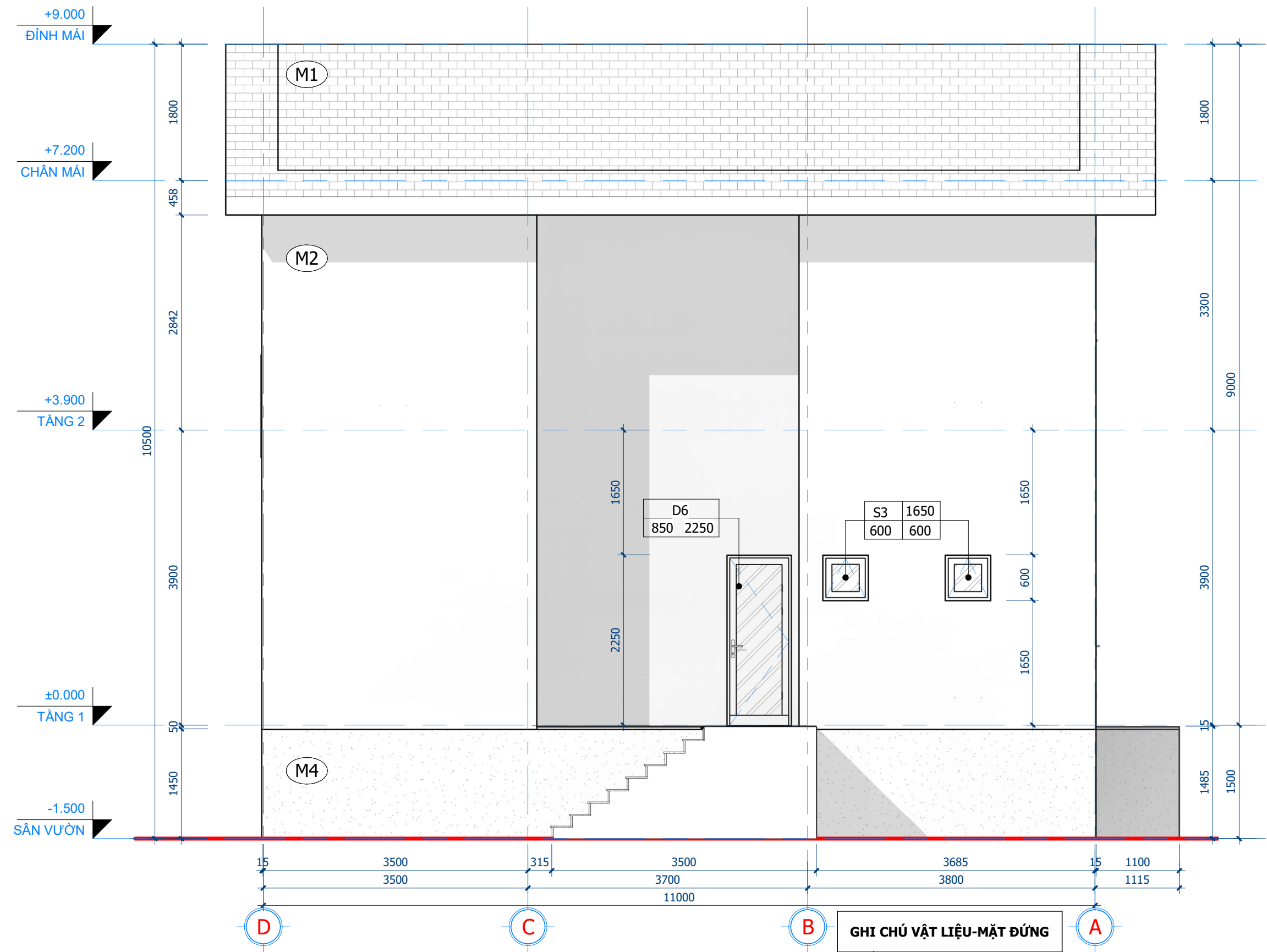
1 MẶT ĐỨNG TRỰC D-A 1 : 50
