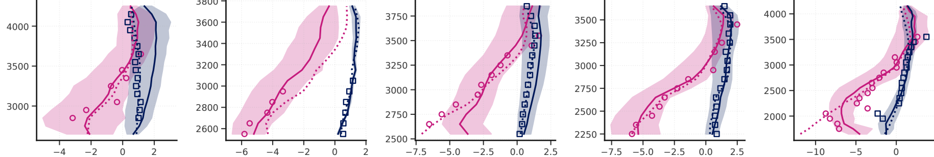
Allalin (1956-2024) Otemma (2020-2022) Findelen (2005-2024) Rhone (2007-2024) Aletsch (1951-2024)
