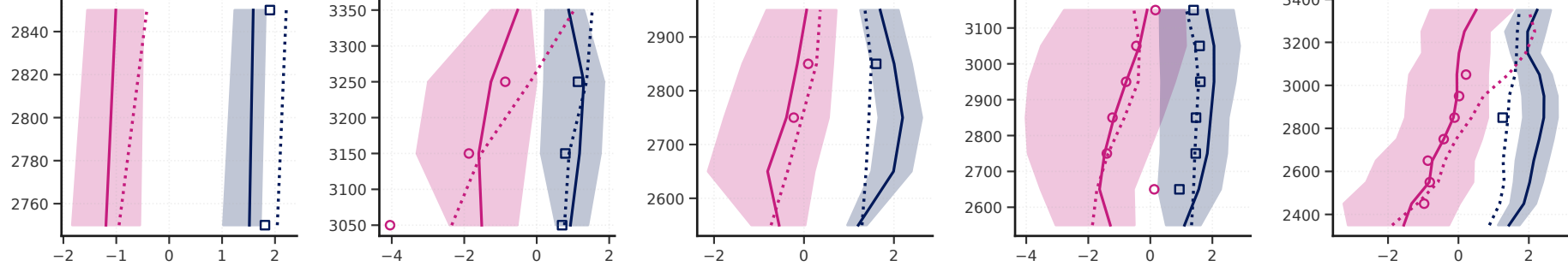
Adler (2007-2024) Hohlaub (1956-2024) Albigna (1955-1960) Tsanfleuron (2010-2024) Silvretta (1951-2024)
