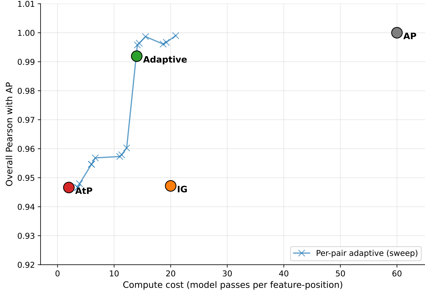
Pareto frontier: all methods
