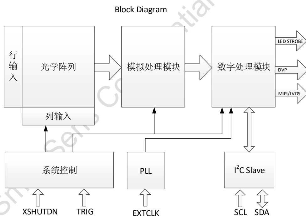
图 1-1 SC035HGS 结构图
