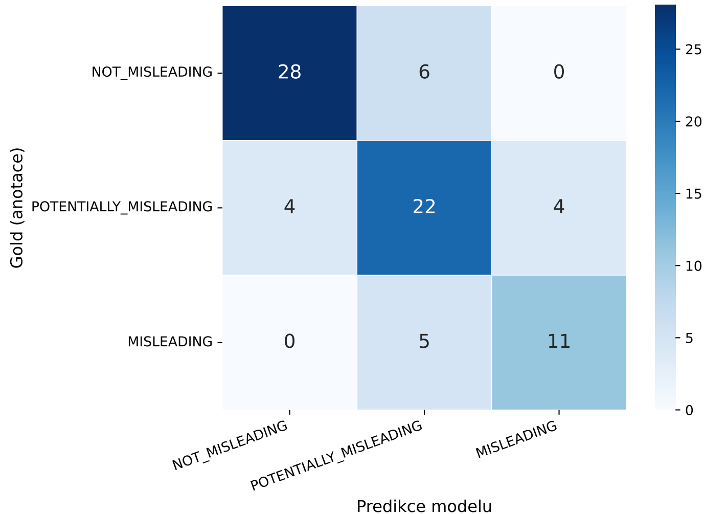
Confusion Matrix — llama_instruct_zs E1-misleading_header_model_final
