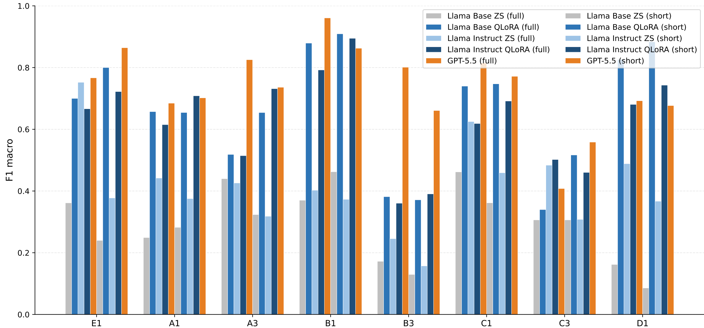
F1 macro napříč anotačními poli
