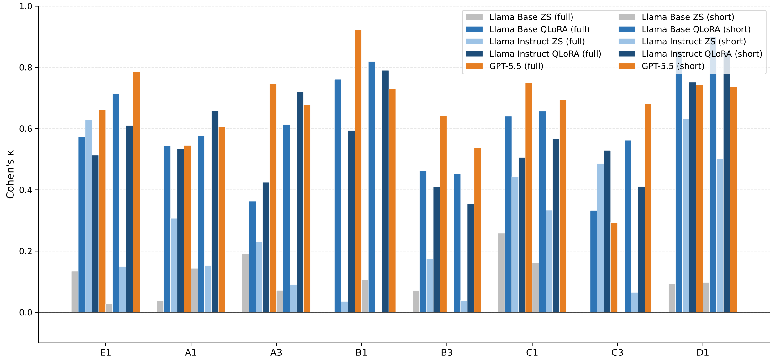
Cohenova \kappa napříč anotačními poli
