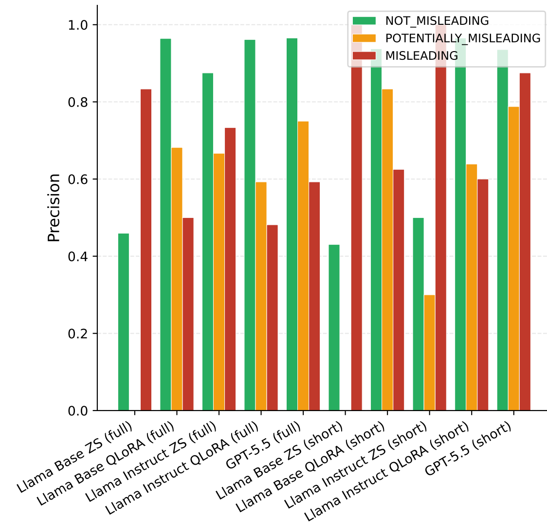
E1 — Precision per třída
