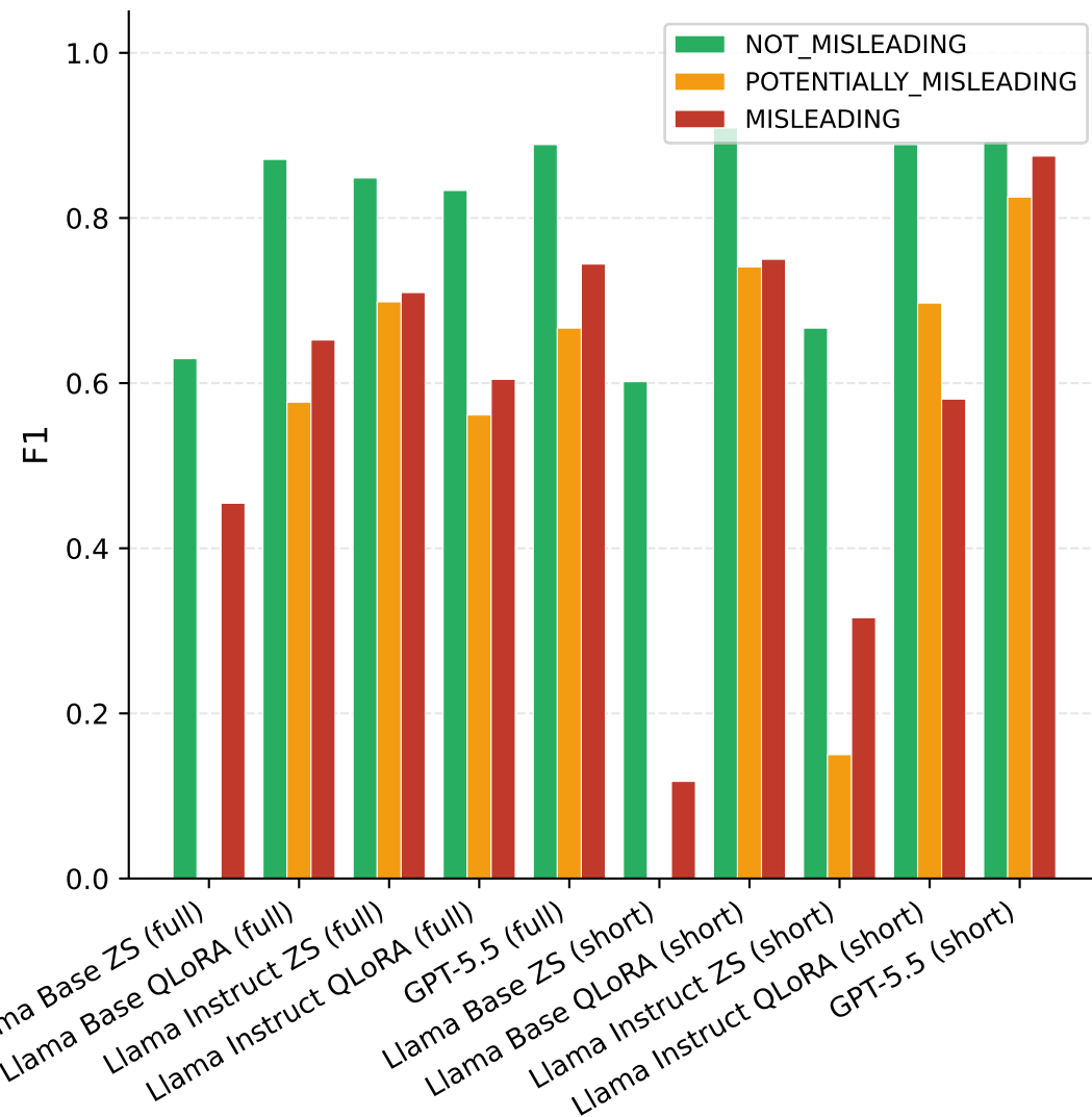
E1 — F1 per třída
