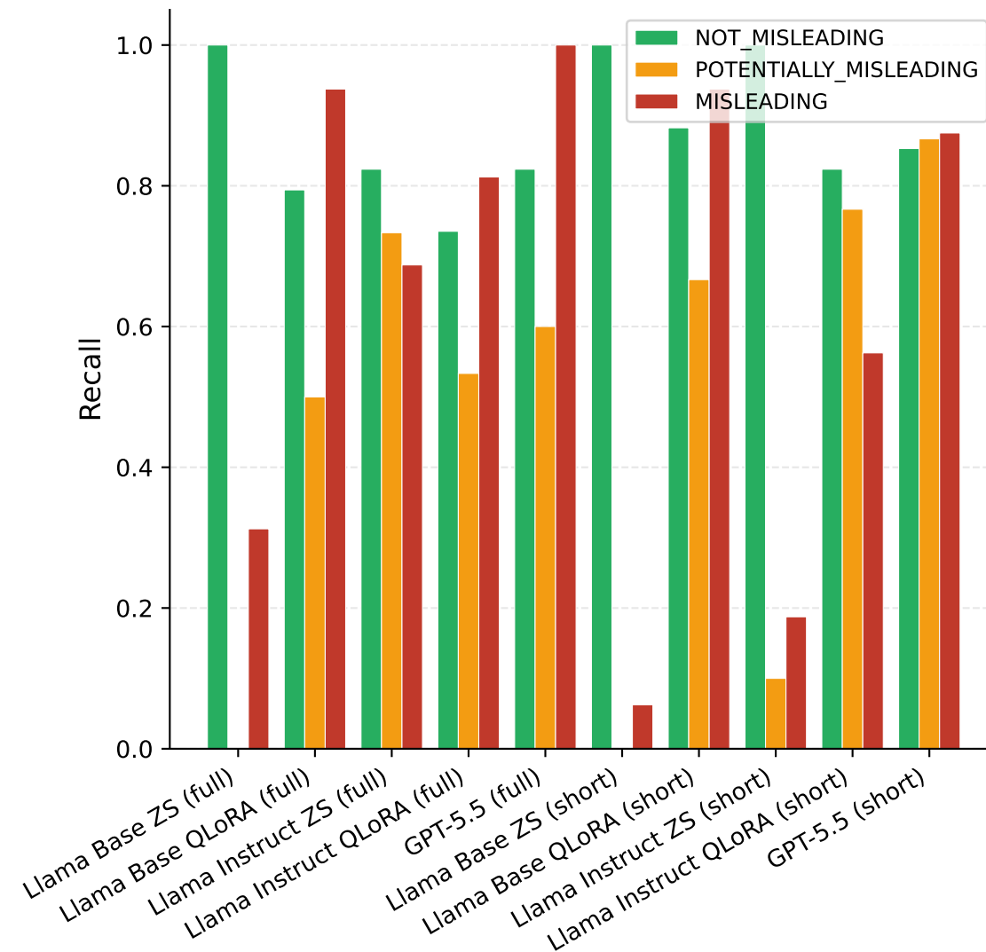
E1 — Recall per třída
