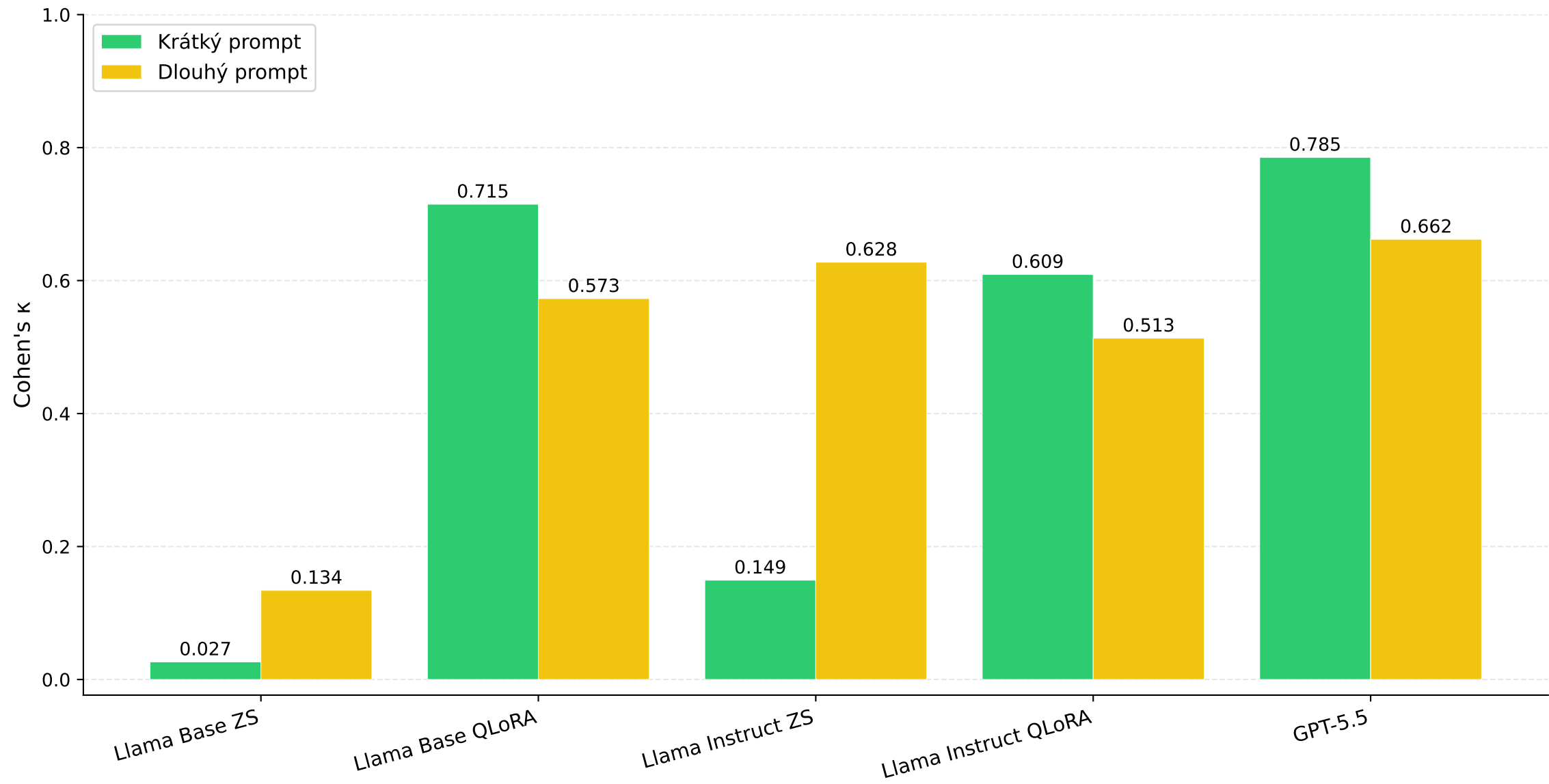
Srovnání shody s experty ( \kappa ) — krátký vs. dlouhý prompt
