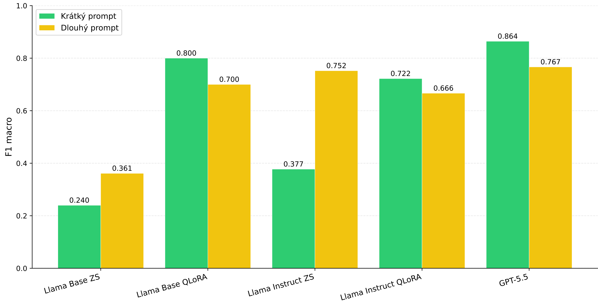
Srovnání F1 macro pro E1 — krátký vs. dlouhý prompt
