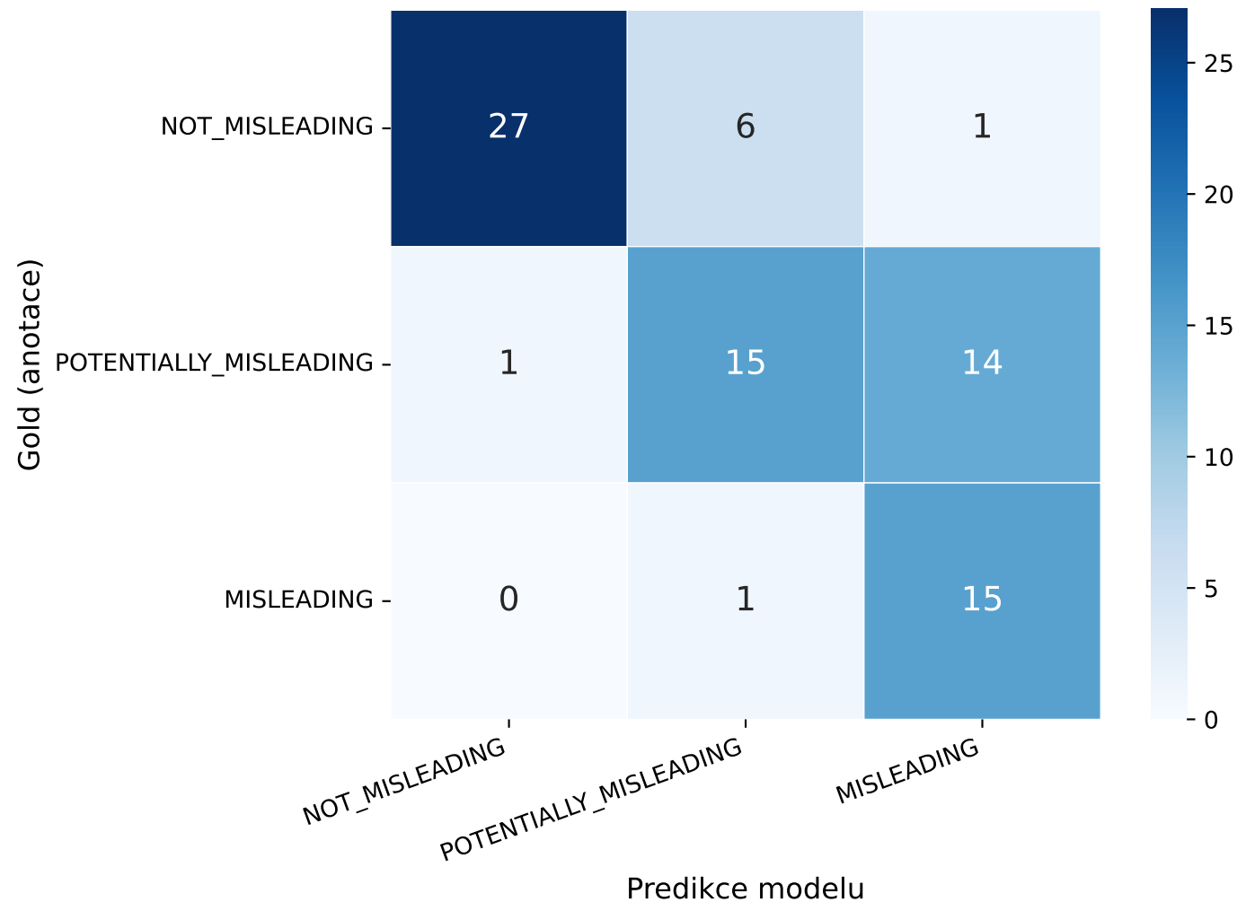
Confusion Matrix — llama_base_qlora_zs E1-misleading_header_model_final
