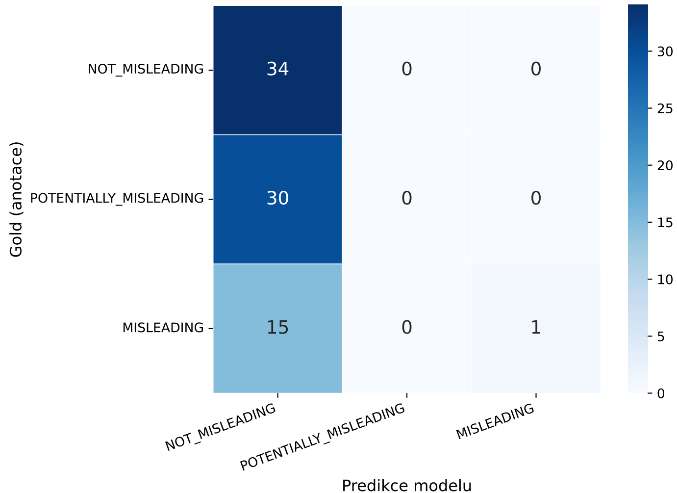
Confusion Matrix — llama_base_zs_short E1-misleading_header_model_final
