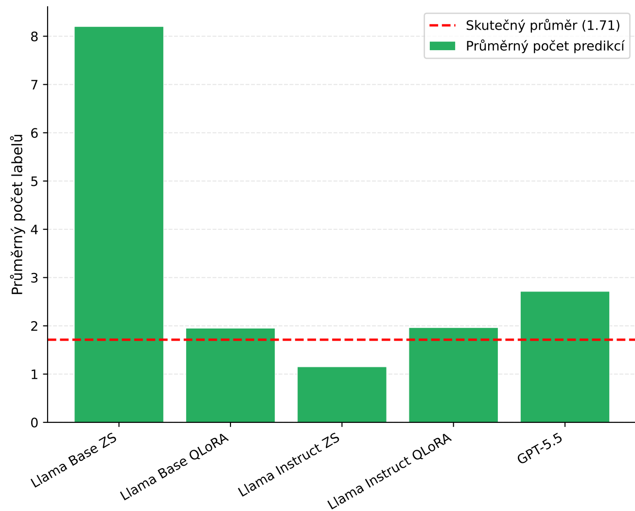
B2: Počet predikovaných štítků vs. realita
