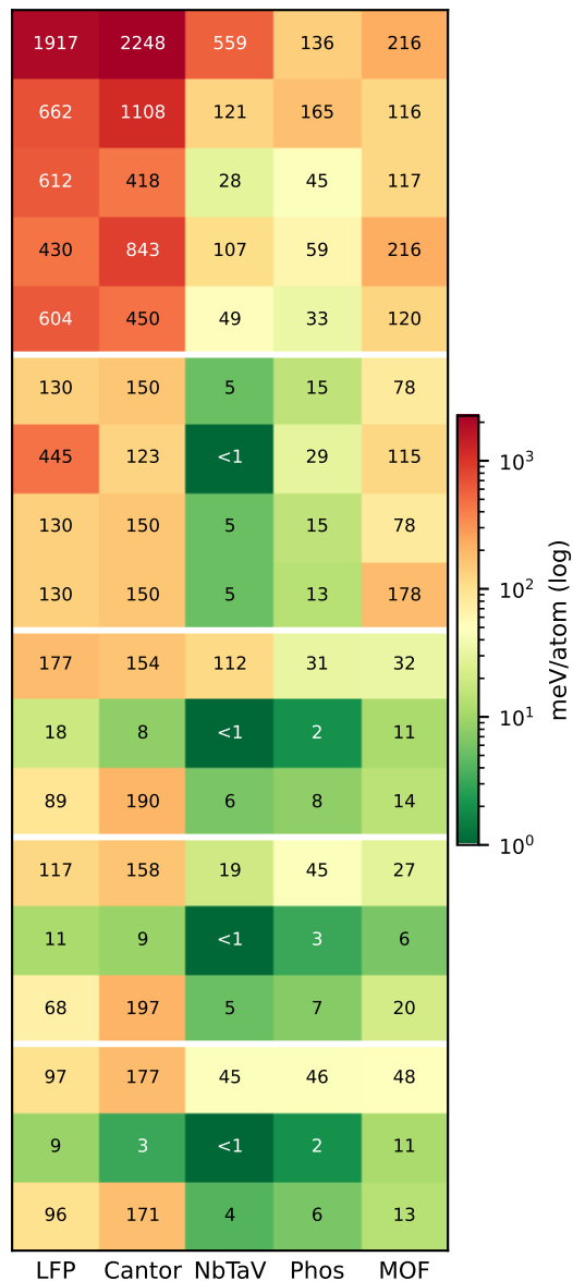
(b) Energy MAE (meV/atom)
