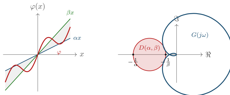
Figura 25.4: Il criterio del cerchio. A sinistra: la non linearità \varphi appartiene al settore [\alpha, \beta] , cioè il suo grafico resta confinato fra le rette y = \alpha x e y = \beta x (regione grigia). A destra: il disco proibito D(\alpha, \beta) , che ha per diametro il segmento reale da -1/\alpha a -1/\beta ; se il diagramma di Nyquist della parte lineare G non entra nel disco (e lo circonda tante volte quanti sono i poli instabili di G ) il sistema in retroazione è assolutamente stabile. Per \alpha = \beta il disco degenera nel punto -1/\alpha e si ritrova il criterio di Nyquist.
