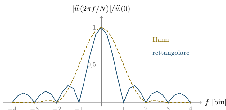
Figura 22.3: Modulo normalizzato della DTFT delle finestre rettangolare e di Hann (periodica), per N = 8 , in funzione della frequenza misurata in bin. Le ordinate sono |D_8(2\pi f/8)|/8 e l'analoga per Hann, calcolate con la forma chiusa del Lemma 22.3 e con la decomposizione in tre nuclei del Teorema 22.15: le due vie coincidono entro 2,5 \cdot 10^{-16} . Si leggono gli zeri previsti dalla Proposizione 22.8: a ogni intero non nullo per la rettangolare, solo da |f| \geq 2 per Hann, il cui lobo principale è quindi doppio in larghezza; in cambio, a f = 2,5 la rettangolare vale 0,15030 e Hann 0,02236, cioè circa sette volte meno.
