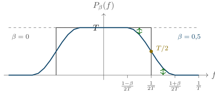
Figura 26.7: Lo spettro a coseno rialzato della Proposizione 26.7, disegnato in unità 1/(2T) = 2 cm sull'ascissa e T = 2 cm sull'ordinata. In grigio il caso ideale \beta = 0 , cioè il rettangolo del Corollario 26.6. In blu il caso \beta = 0,5 : il tratto piatto arriva a \frac{1-\beta}{2T} = 0,25/T (ascissa 1 cm) e la transizione finisce a \frac{1+\beta}{2T} = 0,75/T (ascissa 3 cm). Le ordinate del tratto in transizione sono 2 \cdot \frac{1}{2}[1 + \cos(\pi(2Tf - 0,5))] calcolate in nove punti: 2, 1,92388, 1,70711, 1,38268, 1, 0,61732, 0,29289, 0,07612, 0. I due segmenti verdi hanno la stessa lunghezza, 0,29289 cm: è la simmetria dispari attorno a (\frac{1}{2T}, \frac{T}{2}) dimostrata nel Passo 1, cioè ciò che fa sommare a T le repliche.
