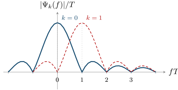
Figura 27.1: Il modulo dello spettro di due sottoportanti troncate sull'intervallo di simbolo (Proposizione 27.1), in scala |\Psi_k(f)|/T contro fT : in blu continuo k = 0 , in rosso tratteggiato k = 1 . Le ordinate sono i valori di |\text{sinc}(fT - k)| calcolati con passo 0,125 (per esempio |\text{sinc}(\frac{1}{2})| = 2/\pi = 0,6366 e |\text{sinc}(\frac{3}{2})| = 2/(3\pi) = 0,2122 ). I due spettri si sovrappongono per gran parte del lobo principale, ma ciascuno si annulla nel centro dell'altro: gli zeri cadono in fT - k = \pm 1, \pm 2, \dots , cioè esattamente nei centri f = \ell/T delle altre sottoportanti. È l'ortogonalità letta nel dominio della frequenza.
