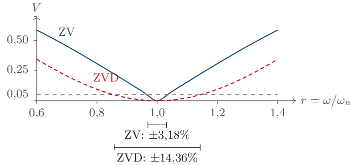
Figura 30.4: Curve di sensibilità di ZV (continua) e ZVD (tratteggiata) nel caso non smorzato, V_{ZV}(r) = |\cos \frac{\pi r}{2}| e V_{ZVD}(r) = \cos^2 \frac{\pi r}{2} (Proposizione 30.9). Ordinate del disegno: 1 unità = 0,25 di vibrazione residua; la linea tratteggiata orizzontale è la soglia del 5%. Valori esatti usati: V_{ZV}(0,9) = 0,156434 , V_{ZVD}(0,9) = 0,024472 ; V_{ZV}(0,8) = 0,309017 , V_{ZVD}(0,8) = 0,095492 . Le due barre sotto l'asse misurano le bande al 5%: \pm 3,18\% per lo ZV e \pm 14,36\% per lo ZVD, in rapporto 4,51.
