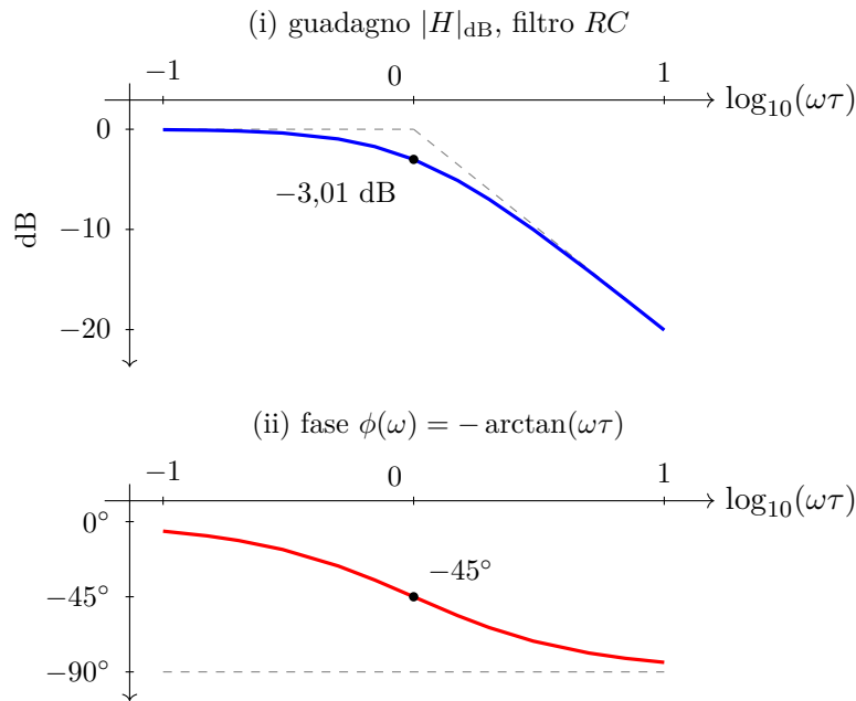
Figura 24.1: Risposta in frequenza del filtro RC dell'Esempio 24.4, in scala logaritmica delle pulsazioni. Le coordinate dei tredici punti di ciascuna curva sono state calcolate dalle formule chiuse |H|_{\text{dB}} = -10\log_{10}(1 + \omega^2\tau^2) e \phi = -\arctan(\omega\tau) e riverificate con uno script: per esempio a \omega\tau = 1 si ha -3,010\,30 dB e -45^\circ , a \omega\tau = 10 si ha -20,043\,21 dB e -84,289\,41^\circ . Le rette tratteggiate sono gli asintoti 0 dB e -20 dB/decade, che si incontrano proprio sulla pulsazione di taglio.
