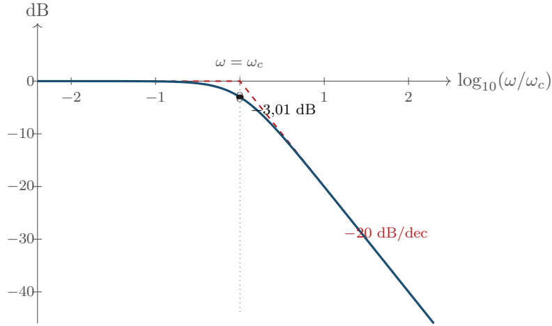
Figura 25.1: Diagramma di Bode del modulo di G(s) = 1/(1 + s/\omega_c) . In rosso tratteggiato le due asintoti (0 dB e -20 dB/decade) che si incontrano nella pulsazione di taglio \omega_c ; in blu il modulo esatto. Lo scarto massimo fra curva e asintoti si ha proprio in \omega = \omega_c e vale -20 \log_{10} \sqrt{2} = -3,01 dB: è il motivo per cui \omega_c si chiama anche pulsazione a -3 dB .
