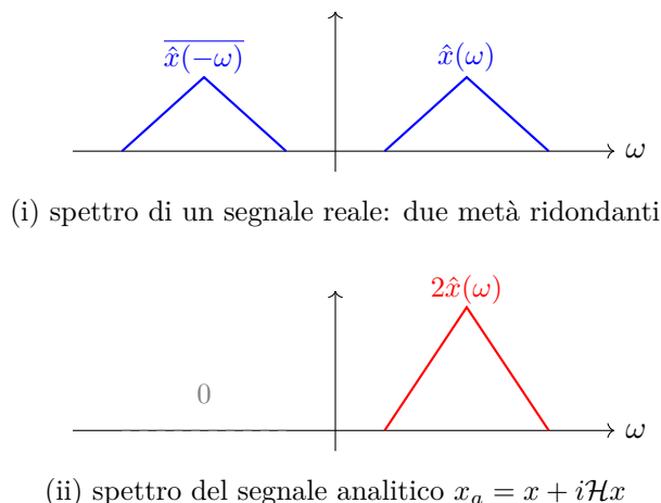
Figura 24.5: Il Teorema 24.11 in figura. Lo spettro di un segnale reale (i) ha due metà legate dalla simmetria hermitiana del Teorema 24.6(iii): la metà negativa non porta informazione nuova. Il segnale analitico (ii) la elimina e raddoppia la metà positiva, così che l'energia si conserva: infatti, per il Teorema 24.11 e per Plancherel, \|x_a\|_2^2 = \frac{1}{2\pi} \int_0^{+\infty} 4|\hat{x}|^2 = \frac{2}{2\pi} \int_{\mathbb{R}} |\hat{x}|^2 = 2\|x\|_2^2 , coerente con \|x_a\|_2^2 = \|x\|_2^2 + \|\mathcal{H}x\|_2^2 = 2\|x\|_2^2 della Proposizione 24.4. I due vertici sono a (\pm 1,6; 0,9) nel pannello (i) e a (1,6; 1,5) nel pannello (ii): il rapporto 1,5/0,9 = 5/3 è solo grafico, la figura è schematica e non in scala di energia.
