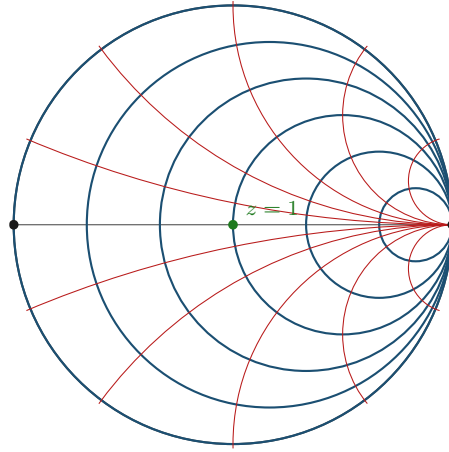
Figura 25.6: Lo scheletro della carta di Smith. In blu i cerchi a resistenza normalizzata costante r ( r = 0; 0,2; 0,5; 1; 2; 5 ), di centro (r/(1+r), 0) e raggio 1/(1+r) : sono tutti tangenti fra loro in \Gamma = 1 . In rosso gli archi a reattanza normalizzata costante x ( x = \pm 0,2; \pm 0,5; \pm 1; \pm 2; \pm 5 ), archi di cerchi di centro (1, 1/x) e raggio 1/|x| , anch'essi tangenti in \Gamma = 1 . Le due famiglie sono ortogonali perché immagini, secondo la trasformazione di Möbius \Gamma = (z-1)/(z+1) , delle rette ortogonali \Re z = r e \Im z = x . Il centro \Gamma = 0 è l'adattamento z = 1 ; il bordo |\Gamma| = 1 è il carico puramente reattivo.
