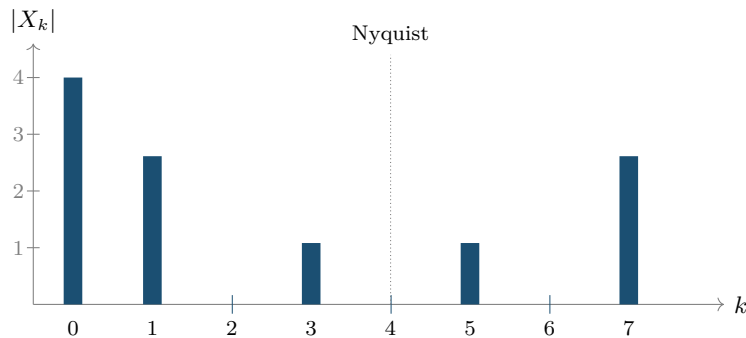
Figura 22.4: Modulo dello spettro di x = (1, 1, 1, 1, 0, 0, 0, 0) . Le altezze sono i valori esatti 4, \sqrt{4 + 2\sqrt{2}} = 2,61313 , 0, \sqrt{4 - 2\sqrt{2}} = 1,08239 , 0, 1,08239, 0, 2,61313, calcolati a mano nel Passo 2 e ricontrollati con lo script. La simmetria attorno al bin 4 (frequenza di Nyquist) è quella del Corollario 22.8(iii): |X_{8-k}| = |X_k| .
