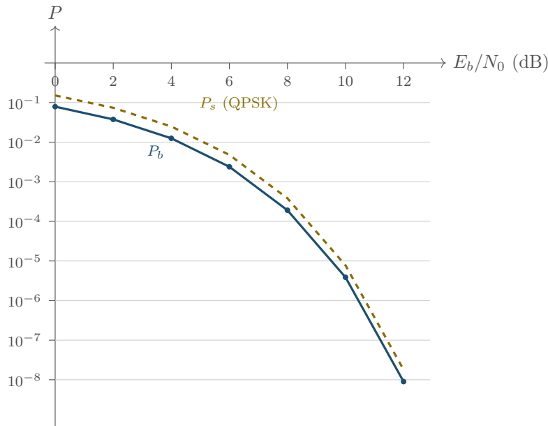
Figura 26.6: Le due curve dell'Esempio 26.6, disegnate dai valori tabulati e non da una misura. La scala orizzontale è 0,55 cm per decibel e quella verticale 0,75 cm per decade: l'ordinata di un punto è 0,75 \log_{10} P . Per esempio a 10 dB si ha P_b = 3,8721082 \cdot 10^{-6} , \log_{10} P_b = -5,41205 e ordinata -4,0590 ; a 12 dB, \log_{10} P_b = -8,04547 e ordinata -6,0341 . La curva continua vale sia per la BPSK sia per la probabilità di bit della QPSK (Teorema 26.10): le due coincidono, e questo è il contenuto grafico del Corollario 26.3. La curva tratteggiata è la probabilità d'errore di simbolo della QPSK, che sta poco sopra perché P_s = 2P_b - P_b^2 \approx 2P_b quando P_b è piccola: uno scarto di 10 \log_{10} 2 = 3,01 dB in ordinata, non in ascissa.
