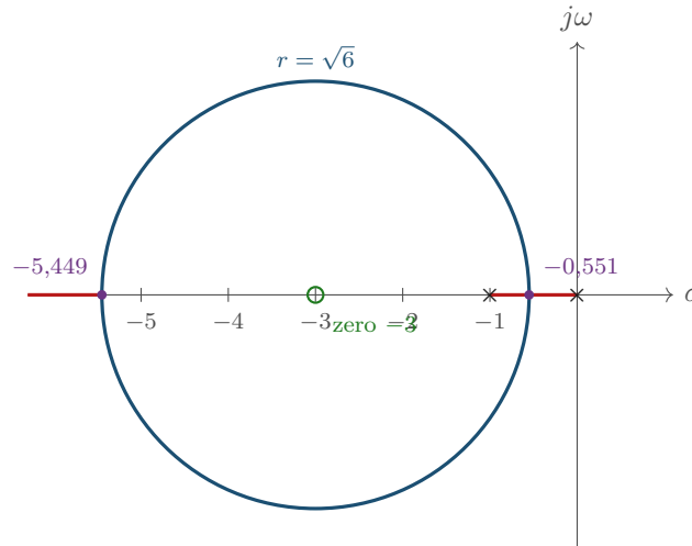
Figura 25.5: Il luogo delle radici di L(s) = K(s + 3)/(s(s + 1)) : poli in 0 e -1 (crocini), zero in -3 (cerchietto). I rami che lasciano l'asse reale descrivono esattamente un cerchio di centro lo zero -3 e raggio \sqrt{(3 - 0)(3 - 1)} = \sqrt{6} \simeq 2,449 . In rosso i tratti di asse reale appartenenti al luogo: il punto di distacco è -3 + \sqrt{6} = -0,551 , quello di rientro -3 - \sqrt{6} = -5,449 . Quando un solo zero finito è presente, il luogo complesso è sempre un cerchio centrato in quello zero.
