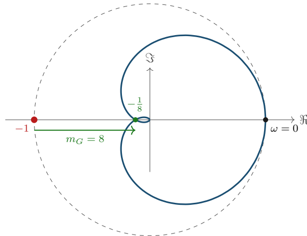
Figura 25.2: Diagramma di Nyquist di L(s) = 1/(1+s)^3 (il ramo per \omega < 0 è il coniugato di quello per \omega > 0 ). La curva non circonda -1 : poiché L non ha poli nel semipiano destro, il criterio di Nyquist dà N = P = 0 e il sistema chiuso è stabile. L'attraversamento dell'asse reale negativo avviene in \omega = \sqrt{3} , dove |L| = 1/8 : il margine di guadagno è m_G = 8 (18,06 dB).
