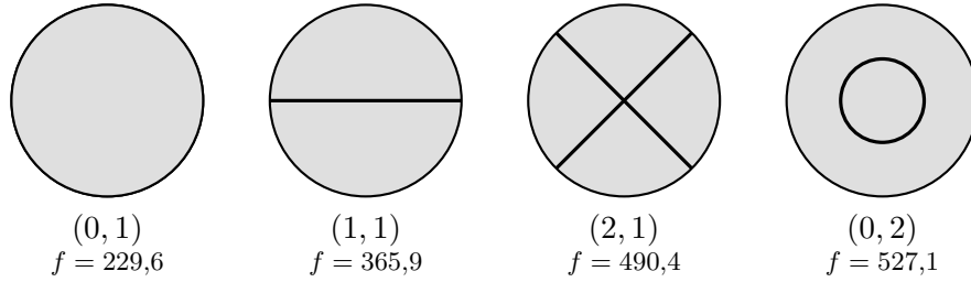
Figura 18.4: Le linee nodali dei primi quattro modi della membrana circolare, con le frequenze in hertz dell'Esempio 18.6. Il modo (0, 1) non ha linee nodali interne; (1, 1) ha un diametro nodale, (2, 1) due diametri (a 45^\circ e 135^\circ : i vertici disegnati sono (\pm 0,813173, \pm 0,813173) , cioè 1,15 \cos 45^\circ = 0,8131728 per il raggio unitario riscaldato a 1,15 cm), e (0, 2) un cerchio nodale di raggio a j_{0,1}/j_{0,2} = 0,4356510 a (qui 0,4356510 \times 1,15 = 0,5009987 cm). Tutte le coordinate sono state calcolate a mano e verificate numericamente.
