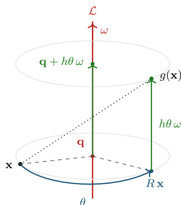
Figura 29.1: Il moto elicoidale del Teorema 29.5. Il punto \mathbf{x} ruota di \theta attorno all'asse \mathcal{L} (freccia blu, lungo l'ellisse che è il cerchio di rotazione visto in prospettiva) e poi trasla di h\theta\omega lungo l'asse (freccia verde). La composizione, in linea punteggiata, è lo spostamento totale g(\mathbf{x}) - \mathbf{x} . I punti dell'asse subiscono la sola traslazione, ed è per questo che sono i punti di spostamento minimo (Proposizione 29.4). Le ellissi hanno semiassi 2 e 0,6; i due punti sul cerchio inferiore corrispondono ai parametri 200^\circ e 320^\circ , cioè (-1,8794, -0,2052) e (1,5321, -0,3857) .
