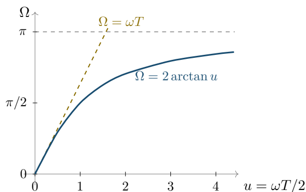
Figura 21.3: Il warping del Corollario 21.5. I valori usati per tracciare la curva sono calcolati esattamente: 2 \arctan u vale 0, 0,927 295 2, 1,570 796 3, 1,965 587 4, 2,214 297 4, 2,498 091 5, 2,651 635 3 e 2,694 639 5 per u = 0; 0,5; 1; 1,5; 2; 3; 4; 4,4 , con asintoto \pi = 3,141 592 7 ; nel disegno l'unità in ordinata è 1,2 cm, cosicché \pi \mapsto 3,77 cm e \pi/2 \mapsto 1,885 cm, e l'unità in ascissa è 1,2 cm. Per u piccolo la curva è indistinguibile dalla retta \Omega = 2u = \omega T ; verso l'alto satura a \pi , cioè alla frequenza di Nyquist: la bilineare comprime tutto l'asse reale delle frequenze continue dentro una sola banda di Nyquist, senza aliasing ma con deformazione.
