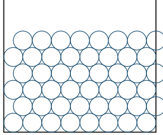
Figura 14.4: Sezione trasversale del carico su bancale (larghezza utile 800 mm): tubi impacchettati a nido d'ape. Le righe sfalsate si annidano con passo verticale d\sqrt{3}/2 = 0,866 d contro il passo d della griglia (Teorema 14.5(iii)): a parità di altezza entrano più strati. I tubi hanno l'asse lungo il lato da 1200 mm del bancale. Nel disegno il diametro è l'unità, la larghezza è 8 diametri e il passo verticale 0,866.
