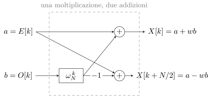
Figura 23.1: La farfalla della Definizione 23.3. Il fattore di rotazione \omega_N^k moltiplica il solo ramo basso; il prodotto wb = t è calcolato una volta sola e usato due volte, con segno opposto — l'etichetta -1 sta sull'arco che porta t al nodo somma inferiore, mentre i tre archi senza etichetta hanno peso 1. Il costo è di una moltiplicazione e due addizioni complesse (Proposizione 23.2).
