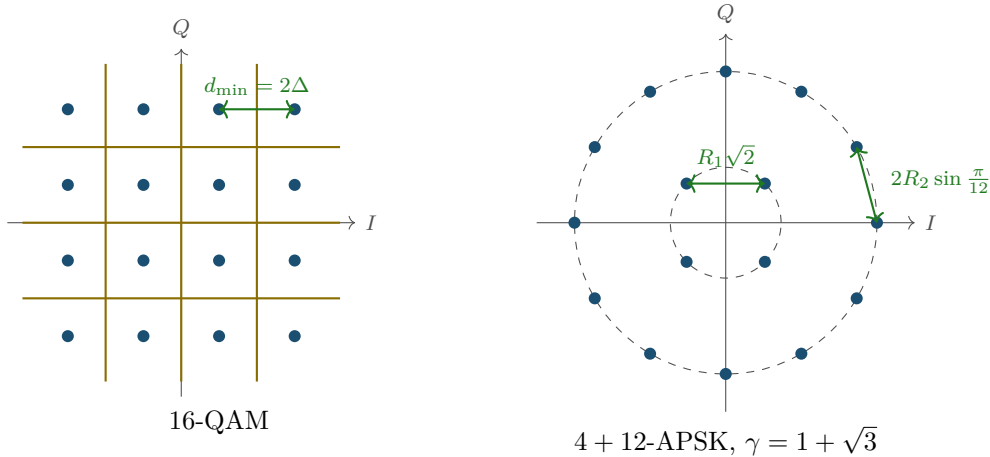
Figura 26.4: A sinistra la 16-QAM della Definizione 26.6 con \Delta = 0,5 cm: i sedici punti stanno in (\pm 0,5, \pm 0,5) , (\pm 0,5, \pm 1,5) , (\pm 1,5, \pm 0,5) , (\pm 1,5, \pm 1,5) , e le rette di decisione a minima distanza sono I, Q \in \{-1, 0, 1\} , cioè i punti medi fra livelli adiacenti (Teorema 26.7). A destra la 4 + 12-APSK ottima del Teorema 26.5, disegnata con R_2 = 2 cm e dunque R_1 = 2/\gamma^* = 2/(1 + \sqrt{3}) = 0,7321 cm: i quattro punti interni stanno a 45^\circ + k \cdot 90^\circ , con coordinate 0,7321 \cdot \frac{\sqrt{2}}{2} = 0,5176 , e i dodici esterni a j \cdot 30^\circ , con coordinate 2 \cos 30^\circ = 1,7321 , 2 \cos 60^\circ = 1 , 2 e 0 . I due segmenti verdi sono le due distanze che nell'ottimo si eguagliano: è la coincidenza h_1 = h_2 della dimostrazione. Tutte le coordinate sono calcolate dalle formule, non misurate.
