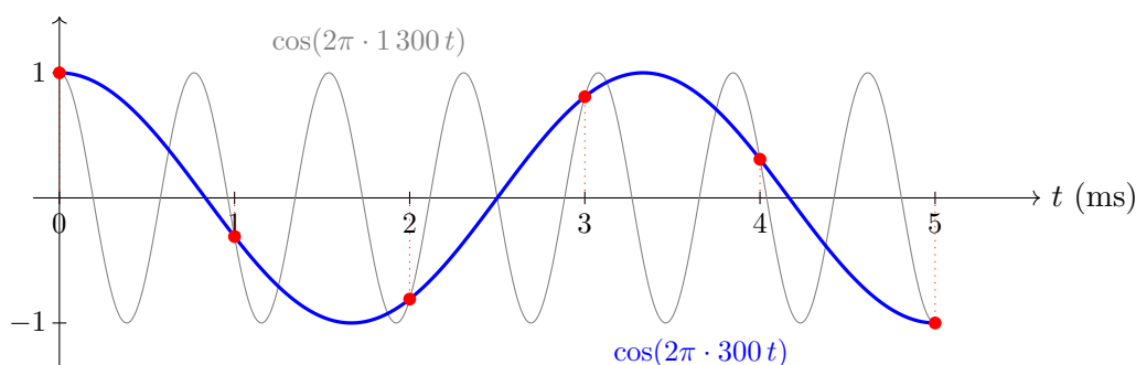
Figura 24.4: Aliasing, Esempio 24.8(a): campionando a \nu_c = 1\,000 Hz (passo 1 ms) la sinusoide a 1300 Hz (grigia) e quella a 300 Hz (blu) passano per gli stessi sei punti rossi, i cui valori 1, -0,309\,017 , -0,809\,017 , 0,809\,017 , 0,309\,017 , -1 sono i coseni degli angoli 0^\circ , 108^\circ , 216^\circ , 324^\circ , 432^\circ , 540^\circ , calcolati a mano e confermati dallo script. Dai soli campioni le due sinusoidi sono indistinguibili, come afferma il Teorema 24.10.
