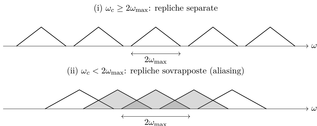
Figura 24.3: Campionare nel tempo replica periodicamente lo spettro di passo \omega_c = 2\pi/T : se \omega_c \geq 2\omega_{\max} le repliche restano separate (i) e il segnale si ricostruisce esattamente; altrimenti si sovrappongono (ii, zone ombreggiate) e l'informazione persa non è più recuperabile — esattamente i due casi della dimostrazione appena vista.
