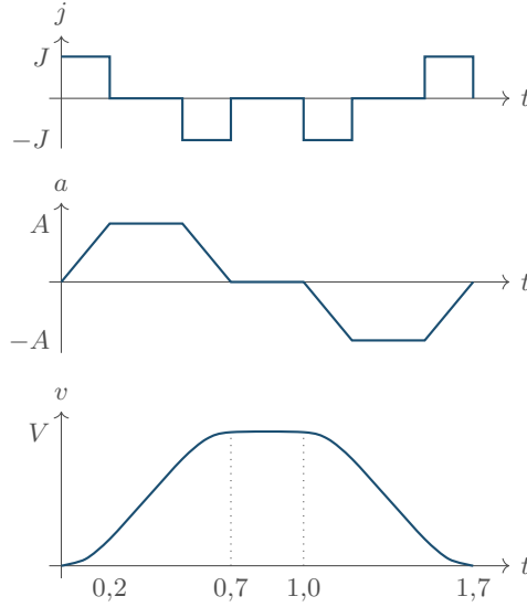
Figura 30.3: Profilo a S a sette segmenti per L = 1 m, V = 1 m/s, A = 2 m/s 2 , J = 10 m/s 3 (Teorema 30.5, caso (a)). Istanti di raccordo, in secondi: 0, 0,2, 0,5, 0,7, 1,0, 1,2, 1,5, 1,7; in quegli istanti l'accelerazione vale 0, 2, 2, 0, 0, -2, -2, 0 (m/s 2 ), la velocità 0; 0,2; 0,8; 1; 1; 0,8; 0,2; 0 (m/s) e la posizione 0; 0,0133; 0,1633; 0,35; 0,65; 0,8367; 0,9867; 1 (m). Il jerk è costante a tratti, l'accelerazione è continua (trapezio), la velocità è C^1 e la posizione C^2 . Le ordinate del disegno sono in scala: J \rightarrow 0,5 , A \rightarrow 0,7 , V \rightarrow 1,6 unità.
