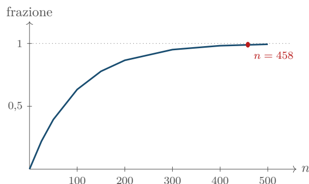
Figura 11.2: La frazione di volume della palla unitaria B^n contenuta nel guscio esterno di spessore \varepsilon = 0,01 , cioè 1 - 0,99^n , in funzione della dimensione. In dimensione 10 vale 0,0956, in dimensione 100 già 0,6340, e supera il 99% a partire da n = 459 (punto rosso: il valore critico 458,21 del Teorema 11.6, Passo 4). L'intuizione bidimensionale, dove la stessa frazione vale 0,0199, è del tutto fuorviante.
