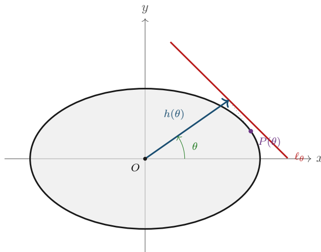
Figura 4.1: La funzione di supporto di un convesso. Per ogni direzione \theta si considera la retta di appoggio \ell_\theta ortogonale a (\cos \theta, \sin \theta) che lascia il corpo tutto da una parte; h(\theta) è la sua distanza con segno dall'origine, e P(\theta) il punto di contatto. La funzione h determina il convesso completamente, e trasforma i problemi geometrici in problemi di analisi di Fourier: il perimetro è L = \int_0^{2\pi} h (formula di Cauchy), l'area è A = \frac{1}{2} \int_0^{2\pi} (h^2 - h'^2) , la larghezza nella direzione \theta è w(\theta) = h(\theta) + h(\theta + \pi) e il raggio di curvatura è \rho = h + h'' . Per l'ellisse disegnata h(\theta) = \sqrt{a^2 \cos^2 \theta + b^2 \sin^2 \theta} .
