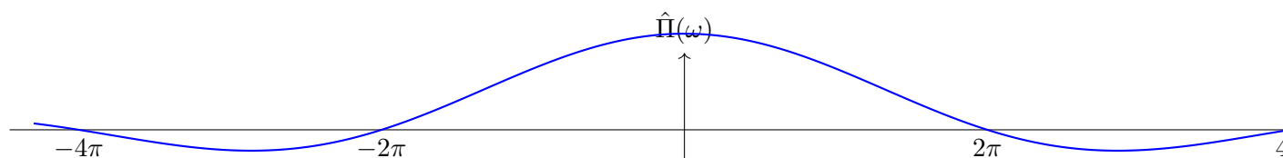
Figura 19.1: La trasformata di Fourier del rettangolo \Pi(t) è la funzione \text{sinc}(\omega/2) : un impulso stretto nel tempo ha uno spettro largo in frequenza, e viceversa (principio di indeterminazione tempo-frequenza).
