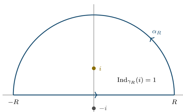
Figura 15.3: Il contorno a D della Proposizione 15.4: segmento [-R, R] più semicirconferenza \alpha_R di raggio R > 1 , percorsi in senso antiorario. Il punto i (ordinata 1) è racchiuso, il punto -i è fuori. Nel disegno R = 3 e il vertice dell'arco è (0, 3) ; il punto -i è disegnato a (0, -0,5) per non uscire dalla figura, ma nel piano complesso ha ordinata -1 : in ogni caso sta nel semipiano inferiore, che il contorno non tocca.
