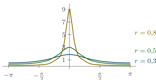
Figura 16.1: Il nucleo di Poisson P_r(t) = \frac{1-r^2}{1-2r \cos t + r^2} per r = 0,3 , r = 0,5 e r = 0,8 . Coordinate calcolate a mano nei punti notevoli e confermate al settimo decimale: P_r(0) = \frac{1+r}{1-r} vale \frac{1,3}{0,7} = 1,8571429 , \frac{1,5}{0,5} = 3 e \frac{1,8}{0,2} = 9 ; P_r(\pi) = \frac{1-r}{1+r} vale 0,5384615 , 0,3333333 e 0,1111111 ; P_{0,5}(\pi/3) = \frac{0,75}{1-0,5+0,25} = 1 esattamente. \checkmark L'area sotto ciascuna curva, divisa per 2\pi , vale 1 (Lemma 16.8): al crescere di r la massa si concentra in t = 0 .
