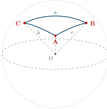
Figura 8.1: Un triangolo sferico sulla sfera unitaria, in proiezione ortografica sull'emisfero visibile. I vertici sono \mathbf{A} di latitudine 70^\circ e longitudine 90^\circ , \mathbf{B} di latitudine 35^\circ e longitudine 45^\circ , \mathbf{C} di latitudine 35^\circ e longitudine 135^\circ ; i lati risultano a = 70,7925^\circ e b = c = 42,5156^\circ , gli angoli A = 117,9875^\circ e B = C = 39,1930^\circ . La somma degli angoli vale 196,3736^\circ : l'eccesso sferico è 16,3736^\circ . Le rette tratteggiate sono i raggi OA , OB , OC : i lati del triangolo sono, per definizione, gli angoli fra questi raggi.
