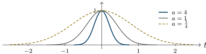
Figura 19.3: Le gaussiane e^{-\pi a t^2} per a = 4 , a = 1 e a = \frac{1}{4} : stessa altezza, larghezze in rapporto 1 : 2 : 4. La trasformata della più stretta ( a = 4 ) è \frac{1}{2} e^{-\pi \xi^2/4} (Corollario 19.2), cioè la curva più larga del disegno dimezzata in altezza, e viceversa: stringere nel tempo allarga in frequenza, esattamente nella proporzione fissata dal Teorema 19.13, per il quale il prodotto delle due dispersioni vale \frac{1}{16\pi^2} = 0,0063326 per ogni a . Valori di controllo sulla curva a = 4 : e^{-4\pi(0,25)^2} = e^{-\pi/4} = 0,4559381 e e^{-4\pi(0,5)^2} = e^{-\pi} = 0,0432139 . ✓
