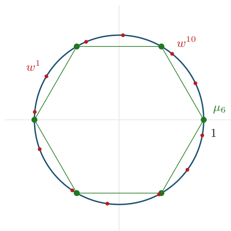
Figura 13.1: I due tipi di sottogruppo. In verde il sottogruppo chiuso \mu_6 : sei punti, vertici di un esagono regolare, di coordinate (\pm 1, 0) , (\pm 0,5, \pm 0,86603) . In rosso i primi dodici punti dell'orbita w^n = e^{2\pi i n \sqrt{2}} , n = 1, \dots, 12 : il sottogruppo che generano è infinito, quindi denso (Teorema 13.8), e nessun punto si ripete. Le coordinate sono (\cos 2\pi n \sqrt{2}, \sin 2\pi n \sqrt{2}) ; per esempio w^1 = (-0,85822, 0,51329) e w^{10} = (0,62703, 0,77900) .
