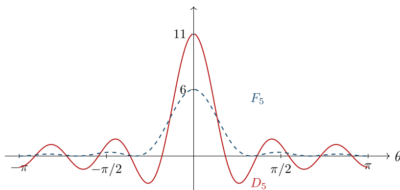
Figura 17.3: Il nucleo di Dirichlet D_5 (continuo) e il nucleo di Fejér F_5 (tratteggiato) su [-\pi, \pi] . Scala: ascisse x = 1,5\theta centimetri, ordinate y = 0,3K centimetri. Valori di controllo calcolati a mano: D_5(0) = 2 \cdot 5 + 1 = 11 e F_5(0) = 5 + 1 = 6 (le altezze marcate sull'asse); D_5(\pi/6) = \sin(11\pi/12)/\sin(\pi/12) = 1 perché \sin(11\pi/12) = \sin(\pi/12) ; D_5(\pi) = \sin(11\pi/2) = -1 ; F_5(\pi/2) = (\sin(3\pi/2)/\sin(\pi/4))^2/6 = 2/6 = 1/3 ; F_5(\pi/3) = 0 perché \sin(\pi) = 0 . D_5 cambia segno, F_5 no: è tutta qui la differenza fra i due mondi.
