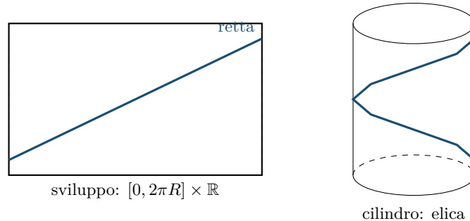
Figura 9.1: Lo sviluppo del cilindro sul piano è un'isometria locale (Proposizione 9.1(i)): le rette del rettangolo diventano le eliche del cilindro. I nodi della spezzata sono i punti (8 + 1,2 \cos t, 0,3 + 2,4t/(2\pi)) per t = 0, \pi/4, \dots, 2\pi , calcolati a mano: 9,200; 8,849; 8,000; 7,151; 6,800; 7,151; 8,000; 8,849; 9,200.
