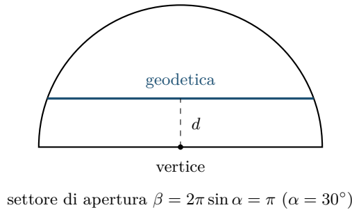
Figura 9.2: Sviluppo del cono di semiapertura \alpha = 30^\circ : un settore di apertura \beta = 2\pi \sin 30^\circ = \pi . Le geodetiche sono i segmenti; quello disegnato ha estremi (3 \cos 20^\circ, 3 \sin 20^\circ) = (2,819; 1,026) e (3 \cos 160^\circ, 3 \sin 160^\circ) = (-2,819; 1,026) , coordinate calcolate a mano, e dista d = 1,026 dal vertice. Per \alpha < 30^\circ il settore è più stretto di \pi e la geodetica, richiudendo il cono, si autointerseca (Proposizione 9.3).
