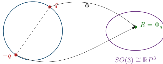
S^3 : i quaternioni unitari
