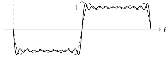
Figura 17.1: Somme parziali dell'onda quadra con 5 termini (tratteggiata) e 10 termini (continua): l'overshoot vicino al salto in \theta = \pi non si riduce passando da 5 a 10 termini, si comprime solo verso il punto di discontinuità — il fenomeno di Gibbs.
