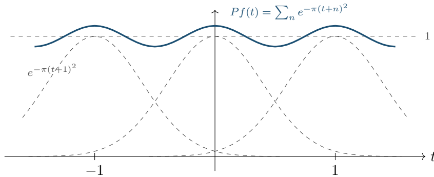
Figura 19.2: Periodizzazione della gaussiana f(t) = e^{-\pi t^2} . Le curve tratteggiate sono le traslate f(t + n) per n = -1, 0, 1 ; la curva spessa è la loro somma su tutti gli n \in \mathbb{Z} , che è 1-periodica e oscilla fra Pf(\frac{1}{2}) = 0,9135791 e Pf(0) = 1,0864348 = \vartheta(1) . La formula di Poisson (Teorema 19.12) dice che i coefficienti di Fourier di questa curva sono i campioni \hat{f}(n) = e^{-\pi n^2} : 1, e^{-\pi} = 0,0432139, e^{-4\pi} = 0,0000035, \dots , e infatti 1 + 2(0,0432139) + 2(0,0000035) = 1,0864348 e 1 - 2(0,0432139) + 2(0,0000035) = 0,9135791 . ✓
