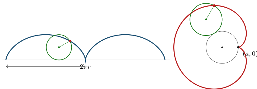
Figura 2.3: Due curve generate dal rotolamento di un cerchio. A sinistra la cicloide: un punto solidale a un cerchio di raggio r che rotola senza strisciare su una retta descrive x = r(t - \sin t) , y = r(1 - \cos t) ; ogni arco ha base 2\pi r , altezza 2r , lunghezza 8r e area 3\pi r^2 . A destra la cardioide, ottenuta facendo rotolare un cerchio di raggio a all'esterno di un cerchio fisso dello stesso raggio: x = 2a \cos t - a \cos 2t , y = 2a \sin t - a \sin 2t . In verde il cerchio generatore nella posizione indicata, in rosso il punto tracciante. È lo stesso meccanismo dei cerchi di Tolomeo e delle serie di Fourier: comporre due moti circolari.
