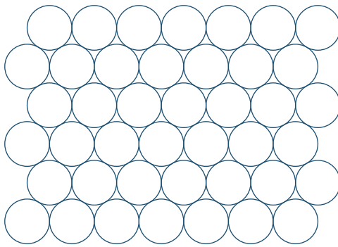
Figura 14.3: Impacchettamento triangolare (detto anche esagonale) di cerchi uguali di raggio 1: i centri stanno nel reticolo generato da (2, 0) e (1, \sqrt{3}) = (1, 1,73205) , ogni cerchio ne tocca sei (numero di bacio 6, Teorema 14.3) e la densità è \pi/\sqrt{12} = 0,9069 , cioè il 90,69% (Teorema 14.4). È la disposizione spontanea di tondini, cavi e tubi affastellati, e la base del nesting di pezzi circolari.
