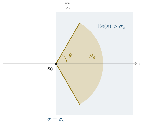
Figura 20.1: Il Teorema 20.2: se l'integrale converge in s_0 , converge in tutto il semipiano aperto \text{Re}(s) > \text{Re}(s_0) (azzurro), e uniformemente nel settore S_\theta di vertice s_0 e semiapertura \theta < \pi/2 (ocra). Nel disegno s_0 = -0,6 , \theta = 60^\circ e il settore ha raggio 2,4: i suoi due vertici stanno in (-0,6 + 2,4 \cos 60^\circ, \pm 2,4 \sin 60^\circ) = (0,6, \pm 2,0785) , con 2,4 \sin 60^\circ = 2,4 \cdot 0,8660254 = 2,0784610 . La retta tratteggiata è la frontiera \text{Re}(s) = \sigma_c , che il teorema non decide.
