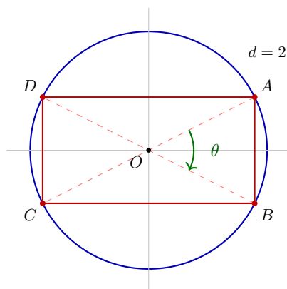
Figura 32.2: Un \theta -rettangolo inscritto nel cerchio unitario, con \theta = 2 \arctan \frac{1}{2} = 0,9272952 (cioè 53,1301024^\circ ) e diagonale d = 2 . I vertici sono (\pm 0,8944272, \pm 0,4472136) , cioè (\pm 2/\sqrt{5}, \pm 1/\sqrt{5}) ; i lati misurano 2/\sqrt{5} = 0,8944272 e 4/\sqrt{5} = 1,7888544 , in rapporto 1 : 2 (Proposizione 32.1). Controllo: (2/\sqrt{5})^2 + (1/\sqrt{5})^2 = \frac{4}{5} + \frac{1}{5} = 1 , i quattro vertici stanno sul cerchio unitario. ✓
