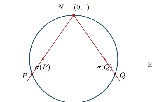
Figura 12.1: La proiezione stereografica \sigma(x, y) = x/(1 - y) di S^1 \setminus \{N\} sulla retta y = 0 : si congiunge N con il punto del cerchio e si legge l'ascissa dell'intersezione con l'asse orizzontale. Per P = (\cos 200^\circ, \sin 200^\circ) = (-0,93969, -0,34202) si ottiene \sigma(P) = -0,70021 ; per Q = (\cos 340^\circ, \sin 340^\circ) si ottiene \sigma(Q) = +0,70021 . Allontanandosi da N lungo il cerchio l'immagine resta finita; avvicinandosi a N diverge, ed è per questo che togliere un solo punto basta a distendere il cerchio su tutta la retta.
