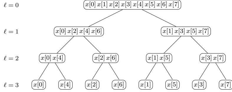
Figura 23.2: Albero della ricorsione per N = 8 . Il livello \ell contiene 2^\ell nodi di lunghezza 2^{3-\ell} , dunque a ogni livello la somma delle lunghezze vale 8, e i livelli sono \log_2 8 + 1 = 4 . Le foglie, lette da sinistra a destra, danno l'ordine x[0], x[4], x[2], x[6], x[1], x[5], x[3], x[7] : è la permutazione bit-reversal della Sezione 23.6 (Teorema 23.7).
