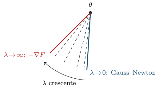
Figura 31.2: Il «ventaglio» di Levenberg–Marquardt nel caso modello J^\top J = \text{diag}(4; 0,25) , J^\top d = (1; 1) , per cui \delta(\lambda) = -(\frac{1}{4+\lambda}; \frac{1}{0,25+\lambda}) . Le direzioni disegnate corrispondono a \lambda = 0 ( -93,5763^\circ ), 0,25 ( -96,7098^\circ ), 1 ( -104,0362^\circ ), 4 ( -117,9795^\circ ), 16 ( -129,0939^\circ ) e \lambda \rightarrow \infty ( -135^\circ , cioè la direzione di -\nabla F = -2(1; 1) ). Verifica del caso limite: per \lambda \rightarrow \infty le due componenti di \lambda\delta(\lambda) tendono entrambe a -1 , dunque l'angolo tende a \arctan(-1/-1) nel terzo quadrante, cioè -135^\circ , come da Teorema 31.7(ii). \checkmark
