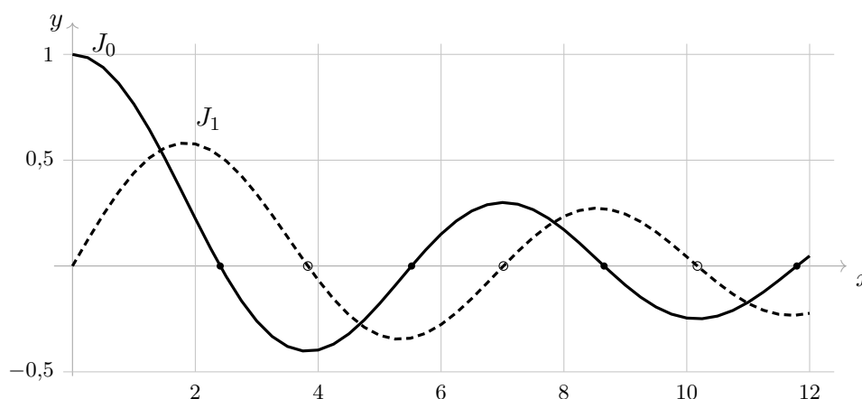
Figura 18.3: Le funzioni J_0 (continua) e J_1 (tratteggiata) su [0, 12] , campionate con passo 0,25 dalla serie della Definizione 18.7 e verificate punto per punto con un'implementazione indipendente in aritmetica multiprecisione (le cifre coincidono tutte a otto decimali). I dischi pieni sull'asse sono i primi quattro zeri di J_0 (2,404826; 5,520078; 8,653728; 11,791534), i cerchietti i primi tre di J_1 (3,831706; 7,015587; 10,173468). L'esistenza di infiniti zeri, tutti semplici, è il Teorema 18.10; l'interlacciamento j_{0,1} < j_{1,1} < j_{0,2} < \dots e la spaziatura che si avvicina a \pi si vedono nel disegno ma qui non sono dimostrati: si veda l'Osservazione 18.13.
