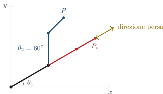
Figura 29.2: Il braccio planare 3R di lunghezze \ell_1 = 2 , \ell_2 = 1,5 , \ell_3 = 1 . Il primo membro (in grigio scuro) è comune alle due configurazioni, che hanno lo stesso \theta_1 = 30^\circ . In blu la configurazione (30^\circ, 60^\circ, -45^\circ) , con vertici (0,0) , (1,7321; 1) , (1,7321; 2,5) , (2,4392; 3,2071) e \det J = 2,598076 . In rosso la configurazione estesa (30^\circ, 0, 0) , con vertici (0,0) , (1,7321; 1) , (3,0311; 1,75) , (3,8971; 2,25) : qui \det J = \ell_1 \ell_2 \sin 0 = 0 e l'utensile, che si trova alla distanza massima 4,5 dall'origine, non può muoversi istantaneamente lungo la direzione (\cos 30^\circ, \sin 30^\circ) del braccio disteso (doppia freccia arancione).
