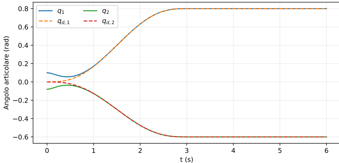
Figura F.2: Posizioni articolari e riferimenti quintici del Capitolo 36. Le due integrazioni sono indistinguibili alla scala del grafico; i loro dati separati restano in dinamica_traccia.csv .
