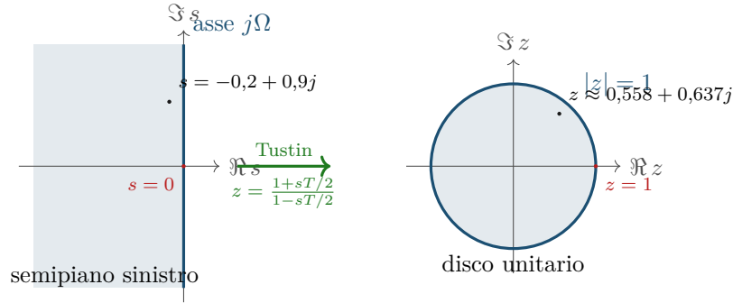
Figura 37.1: La trasformazione di Tustin manda il semipiano sinistro del piano s (in azzurro) nel disco unitario del piano z (in azzurro), e l'asse immaginario j\Omega sulla circonferenza |z| = 1 : esattamente il Teorema 37.2. Punto verificato con T = 1 : s = -0,2 + 0,9j dà 1 + sT/2 = 0,9 + 0,45j , 1 - sT/2 = 1,1 - 0,45j , quindi z = (0,9 + 0,45j)/(1,1 - 0,45j) = 0,5575 + 0,6372j , con |z| \approx 0,847 < 1 ; controllo indipendente dall'identità della dimostrazione: |1 + sT/2|^2 - |1 - sT/2|^2 = 1,0125 - 1,4125 = -0,4 = 2T \operatorname{Re} s .
