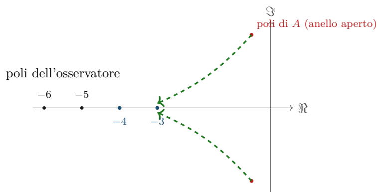
Figura 34.1: L'esempio dell'oscillatore, in un colpo d'occhio: i poli ad anello aperto (rosso, -0,5 \pm 1,9365j , radici di s^2 + s + 4 ) vengono spostati dalla retroazione di stato K = (8, 6) sui poli desiderati -3, -4 (blu, radici di s^2 + 7s + 12 , Teorema 34.3); i poli dell'osservatore -5, -6 (neri, guadagno L = (10, 16) , Esercizio 34.3) restano distinti, come richiede il principio di separazione.
