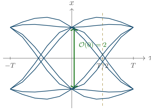
Figura 26.8: Il diagramma a occhio di ordine 2 dell'Esempio 26.8, disegnato dai valori dell'impulso a coseno rialzato con \beta = 0,5 e non da una misura. Scala: T = 2,6 cm sull'ascissa e un'unità di ampiezza = 1,3 cm sull'ordinata; ogni traccia è la spezzata sugli undici punti \tau = -1,0; -0,8; \dots; 1,0 (in unità di T ). Le otto tracce corrispondono alle otto terne (a_{-1}, a_0, a_1) e sono a due a due opposte, per la linearità della somma: le quattro con a_{-1} = -1 sono le riflesse delle quattro disegnate per prime. In \tau = 0 tutte passano per \pm 1 : l'occhio è aperto di \mathcal{O}(0) = 2 (segmento verde), ed è il contenuto della Proposizione 26.9 per un impulso di Nyquist. Sulla verticale tratteggiata \tau = T/2 le tracce si incrociano attraversando lo zero: là l'occhio è chiuso, D(T/2) = -0,1200422 .
