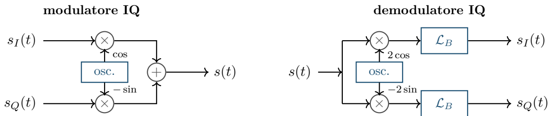
Figura 26.2: Il modulatore e il demodulatore in quadratura. A sinistra il Teorema 26.1(iv), letto come schema: le due componenti moltiplicano rispettivamente \cos(2\pi f_c t) e -\sin(2\pi f_c t) e si sommano. A destra il Corollario 26.1: si moltiplica per 2\cos(2\pi f_c t) e per -2\sin(2\pi f_c t) e si elimina con il filtro passa-basso \mathcal{L}_B il termine attorno a 2f_c che quella moltiplicazione genera. I due rami non si disturbano a vicenda perché le portanti sono ortogonali (Proposizione 26.2 e Corollario 26.2): è l'unica ragione per cui due flussi indipendenti possono occupare la stessa frequenza.
