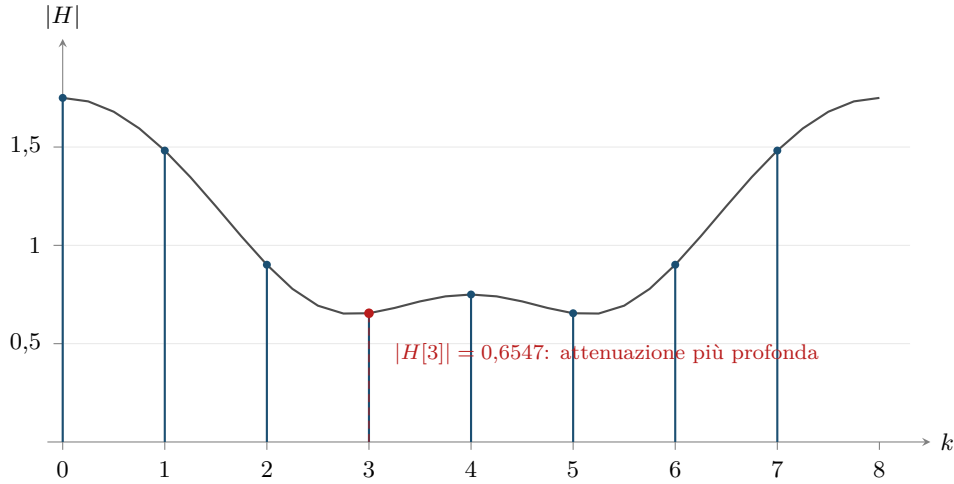
Figura 27.5: La risposta in frequenza del canale h = (1, \frac{1}{2}, \frac{1}{4}) dell'esempio N = 8 . La curva grigia è |H(\theta)| al variare continuo della frequenza, calcolata con passo 0,25 in unità di spaziatura fra sottoportanti; i segmenti blu sono gli otto campioni |H[k]| , cioè gli autovalori in modulo della matrice circolante C_h (Teorema 27.7). La sottoportante k = 3 e la sua simmetrica k = 5 cadono nel minimo e subiscono 8,54 dB di svantaggio rispetto alla sottoportante k = 0 (Corollario 27.4 ed Esempio 27.2). Il valore |H[8]| non esiste: il grafico è 8-periodico, e k = 8 coincide con k = 0 (Osservazione 27.3).
