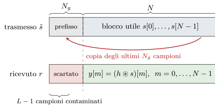
Figura 27.3: Il prefisso ciclico. In alto il blocco trasmesso: gli ultimi N_g campioni del simbolo sono copiati in testa (freccia rossa). In basso il blocco ricevuto: la coda del blocco precedente contamina soltanto i primi L - 1 campioni (Lemma 27.1), e se N_g \geq L - 1 questi cadono tutti nella regione scartata. Sui restanti N campioni il canale ha prodotto esattamente la convoluzione circolare (Teorema 27.5). La figura è disegnata per N = 8 e N_g = 2 , i valori dell'esempio della Sezione 27.9.
