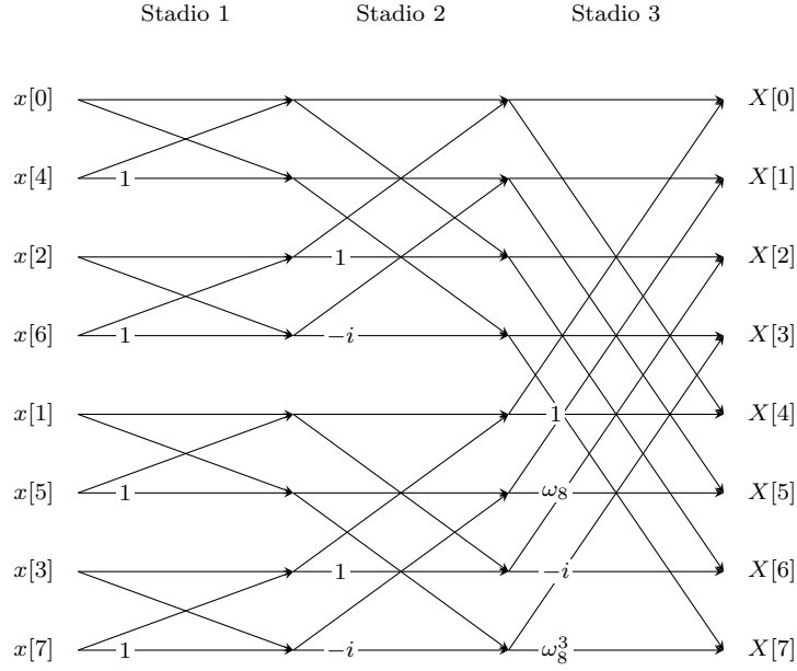
Figura 23.3: Grafo di flusso della FFT radice-2 DIT per N = 8 : stadio 1 con blocchi di lunghezza n_1 = 2 , stadio 2 con n_2 = 4 , stadio 3 con n_3 = 8 . L'ingresso è in ordine bit-reversed x[0], x[4], x[2], x[6], x[1], x[5], x[3], x[7] (Teorema 23.7), l'uscita in ordine naturale. Ogni nodo somma i valori entranti; l'etichetta posta subito dopo un nodo sorgente indica il fattore di rotazione applicato al ramo «basso» di quella farfalla. Dei due archi che escono dal nodo basso, quello che sale porta +\omega e quello orizzontale porta -\omega : sono le due formule del Corollario 23.1. Delle 12 moltiplicazioni complesse ( \frac{8}{2} \log_2 8 = 12 ), 10 hanno fattore 1 o -i e sono dunque banali: restano le sole 2 moltiplicazioni non banali, per \omega_8 e \omega_8^3 .
