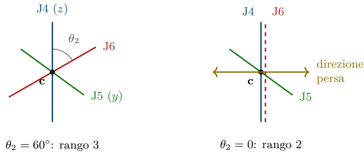
Figura 29.3: Il polso sferico ZYZ, visto nel piano xz del foglio con \theta_1 = 0 ; l'asse J5, che punta lungo y cioè fuori dal foglio, è tracciato obliquo. A sinistra la configurazione regolare \theta_2 = 60^\circ : i tre assi si incontrano nel centro \mathbf{c} e sono linearmente indipendenti; J6 forma con J4 l'angolo \theta_2 ed è diretto lungo (\sin 60^\circ, \cos 60^\circ) = (0,8660; 0,5000) . A destra la configurazione singolare \theta_2 = 0 : J6 torna a coincidere con J4 (tratteggio rosso, spostato di poco per leggibilità), le colonne indipendenti scendono a due e il polso non può ruotare attorno alla direzione R_1 \mathbf{e}_1 , ortogonale al piano di J4 e J5 (doppia freccia arancione). È la singolarità di polso, quella che i controllori segnalano quando il quinto asse attraversa lo zero.
