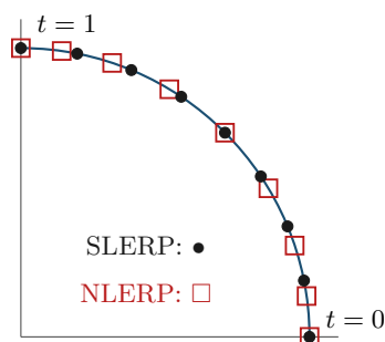
Figura 30.2: SLERP contro NLERP sull'arco fra due orientamenti a \Omega = 90^\circ (una sezione bidimensionale di S^3 vista come cerchio; raggio del disegno 3). Nove istanti equispaziati t = 0, \frac{1}{8}, \dots, 1 . I punti neri (SLERP) cadono agli angoli 0^\circ, 11,25^\circ, \dots, 90^\circ , esattamente equispaziati (Proposizione 30.5). I quadrati rossi (NLERP) cadono agli angoli \arctan \frac{t}{1-t} , cioè 0^\circ, \arctan \frac{1}{7} = 8,130^\circ, \arctan \frac{1}{3} = 18,435^\circ, \arctan \frac{3}{5} = 30,964^\circ, 45^\circ , e simmetricamente: sono addensati agli estremi e diradati al centro, perché per la Proposizione 30.7(iii) la velocità angolare della NLERP è minima agli estremi e doppia a metà percorso. Da qui il moto non uniforme dell'utensile.
