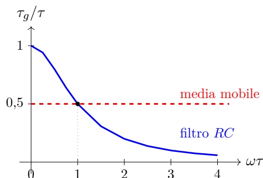
Figura 24.2: Ritardo di gruppo normalizzato. Per il filtro RC vale \tau_g/\tau = 1/(1 + \omega^2\tau^2) e decresce da 1 a 0: le componenti lente escono ritardate di \tau , quelle veloci quasi subito, e la forma d'onda si deforma. Per la media mobile di finestra T_0 = \tau vale invece \tau_g = T_0/2 = \tau/2 per ogni \omega , cioè \tau_g/\tau = 0,5 : è la retta orizzontale tratteggiata, e per il Teorema 24.7 essa significa nessuna distorsione di forma d'onda entro la banda in cui il guadagno resta costante. Le undici coordinate della curva blu sono calcolate dalla formula chiusa e verificate: a \omega\tau = 1 vale 0,5, a \omega\tau = 3 vale 0,1, a \omega\tau = 4 vale 0,058 824.
