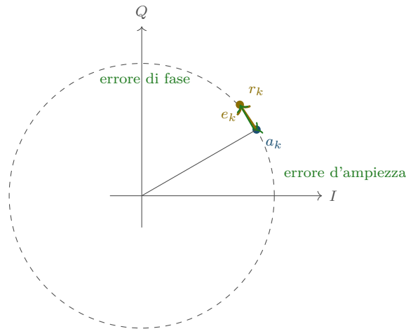
Figura 26.9: Il vettore d'errore della Definizione 26.16. Il simbolo ideale è a_k = 2,5 e^{i\pi/6} , cioè (2,5 \cos 30^\circ, 2,5 \sin 30^\circ) = (2,1651, 1,25) in centimetri; il simbolo ricevuto è r_k = (1,85, 1,72) , scelto per la figura. Il vettore d'errore è e_k = r_k - a_k = (-0,3151, 0,4700) , di modulo \sqrt{0,3151^2 + 0,4700^2} = 0,5659 . La sua decomposizione nella base (\frac{a_k}{|a_k|}, i \frac{a_k}{|a_k|}) = ((0,8660, 0,5), (-0,5, 0,8660)) dà la componente radiale -0,3151 \cdot 0,8660 + 0,4700 \cdot 0,5 = -0,0379 (errore d'ampiezza) e la componente tangenziale 0,3151 \cdot 0,5 + 0,4700 \cdot 0,8660 = 0,5646 (errore di fase). Il quadrato del modulo si ritrova dalle due componenti: 0,0379^2 + 0,5646^2 = 0,3202 = 0,5659^2 . ✓
