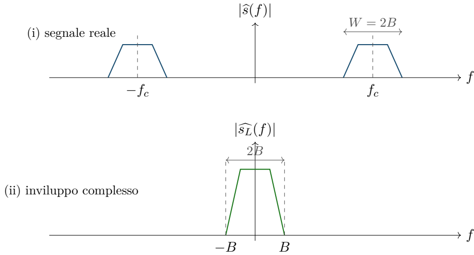
Figura 26.1: La traslazione della Definizione 26.2, disegnata con f_c = 3,2 e B = 0,8 nelle unità della figura. In (i) lo spettro di un segnale reale passa-banda: due gobbe simmetriche rispetto all'origine, di larghezza W = 2B ciascuna, legate dalla simmetria hermitiana \widehat{s}(-f) = \overline{\widehat{s}(f)} (Passo 1 della dimostrazione del Teorema 26.1). In (ii) lo spettro dell'inviluppo complesso: si tiene la sola gobba positiva, la si raddoppia e la si trasla nell'origine. La gobba di (ii) è disegnata alta il doppio di quella di (i) proprio perché \widehat{s_L}(f) = 2\widehat{s}(f + f_c) ; non è simmetrica, e non deve esserlo, perché s_L non è reale. Le altezze e le ascisse dei quattro vertici di ciascuna spezzata sono quelle scritte nel sorgente e non provengono da alcuna misura.
