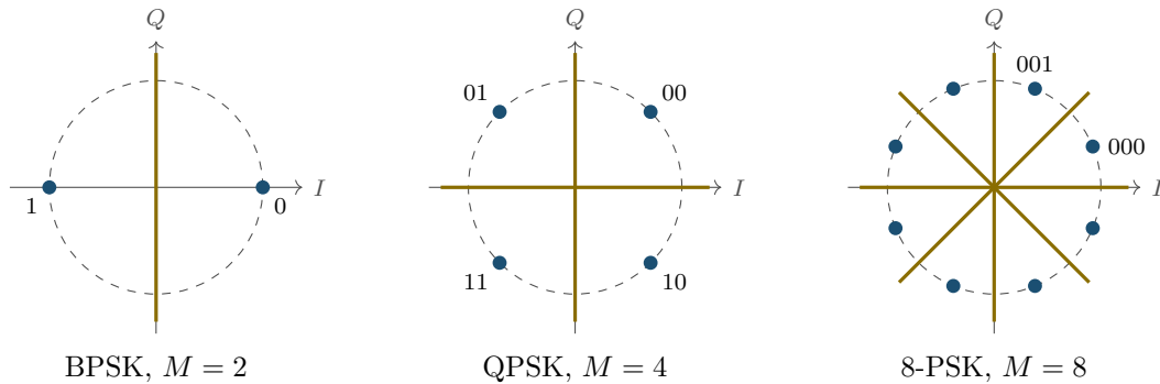
Figura 26.3: Le tre costellazioni PSK, disegnate dalla Definizione 26.4 con \varphi_0 = 0 per la BPSK, \varphi_0 = \pi/8 per la 8-PSK e \varphi_0 = \pi/4 per la QPSK e \varphi_0 = \pi/4 per la QPSK. Il raggio del cerchio tratteggiato è \sqrt{E_s} , qui 1,35 cm. Le coordinate dei punti sono R \cos \theta e R \sin \theta con R = 1,35 : per la QPSK 1,35 \cdot \frac{\sqrt{2}}{2} = 0,9546 ; per la 8-PSK 1,35 \cos 22,5^\circ = 1,2473 e 1,35 \sin 22,5^\circ = 0,5166 , e i confini fra le regioni di decisione stanno a 0^\circ, 45^\circ, \dots con 1,7 \cdot \frac{\sqrt{2}}{2} = 1,2021 . Le linee spesse sono i confini delle regioni di decisione a minima distanza (Teorema 26.7): per la PSK sono i settori circolari delimitati dalle bisettrici degli archi fra simboli adiacenti. Le etichette binarie seguono una mappatura di Gray (Proposizione 26.5).
