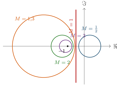
Figura 25.3: La famiglia dei cerchi M : luoghi dei punti L del piano complesso in cui il modulo della funzione ad anello chiuso |L/(1+L)| vale M . Per M \neq 1 si tratta di cerchi di centro (-M^2/(M^2-1), 0) e raggio M/|M^2-1| ; per M = 1 il cerchio degenera nella retta \Re L = -1/2 , asse del segmento fra l'origine e -1 . I cerchi con M > 1 circondano il punto critico -1 e si stringono su di esso al crescere di M : il picco di risonanza del sistema chiuso si legge come il più piccolo M il cui cerchio tocca il diagramma di Nyquist.
