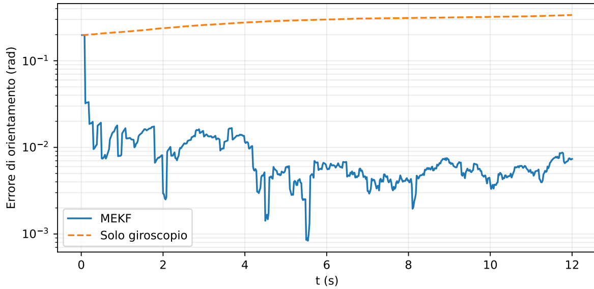
Figura F.1: Errore geodetico dell'orientamento in radianti. La scala verticale è logaritmica; i dati sono in mekf_traccia.csv .
