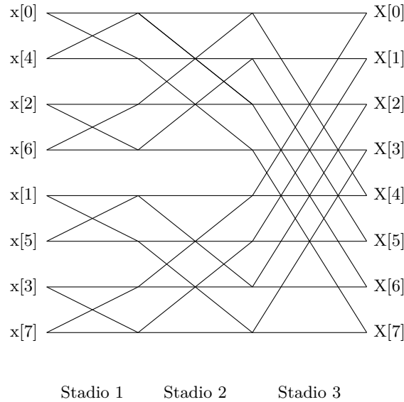
Figura 22.2: Rete a farfalla dell'algoritmo FFT radix-2 (decimazione nel tempo) per N = 8 : ingresso in ordine bit-reversed (sinistra), \log_2 8 = 3 stadi di farfalle (le linee diagonali portano il fattore di torsione \zeta_N^k ), uscita in ordine naturale (destra) — la stessa struttura implementata iterativamente nel Listato 4.3 (FB_FFT8) e alla base della domanda d'esame sulla complessità O(N \log N) (Teorema 22.14).
