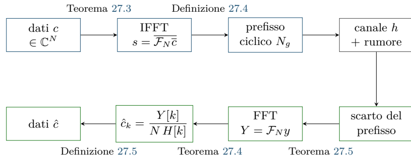
Figura 27.2: La catena OFDM completa. In alto il trasmettitore, in basso il ricevitore letto da destra a sinistra. Ogni blocco è un risultato di questo capitolo: l'unica operazione costosa è la coppia FFT/IFFT (Corollario 27.2), e l'equalizzazione del canale si riduce a N divisioni complesse (Definizione 27.5).
