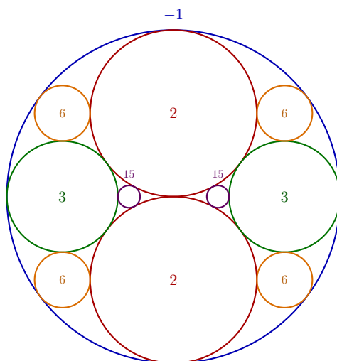
Figura 32.3: Le prime generazioni dell’impacchettamento apolloneo di quaterna radice (-1, 2, 2, 3) , con le curvature indicate. Centri e raggi, tutti calcolati a mano e verificati nell’Esempio 32.4: curvatura -1 , centro (0, 0) , raggio 1 ; curvatura 2 , centri (0, \pm \frac{1}{2}) , raggio \frac{1}{2} ; curvatura 3 , centri (\pm \frac{2}{3}, 0) , raggio \frac{1}{3} ; curvatura 6 , centri (\pm \frac{2}{3}, \pm \frac{1}{2}) , raggio \frac{1}{6} ; curvatura 15 , centri (\pm \frac{4}{15}, 0) , raggio \frac{1}{15} . Tutte le curvature sono intere, come impone il Corollario 32.2.
