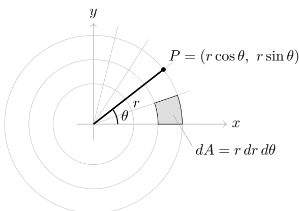
Figura 18.1: Le coordinate polari: i cerchi r = \text{cost} e i raggi \theta = \text{cost} si incontrano ortogonalmente. Il punto disegnato ha r = 2,2 e \theta = 38^\circ , cioè x = 2,2 \cos 38^\circ = 1,7336238 e y = 2,2 \sin 38^\circ = 1,3544553 (valori verificati per doppio calcolo). L'elemento d'area ombreggiato ha lati dr e r d\theta : è il fattore r del determinante jacobiano del Lemma 18.1, e la stessa asimmetria fra le due direzioni produce il termine \frac{1}{r} u_r del Teorema 18.1.
