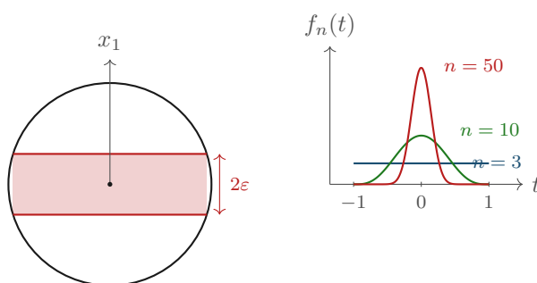
Figura 11.3: La concentrazione della misura sulla sfera. A sinistra: la fascia equatoriale |x_1| \leq \varepsilon ; in dimensione alta essa contiene quasi tutta la misura superficiale, per quanto sottile la si prenda. A destra: la densità della prima coordinata di un punto uniforme su S^{n-1} , f_n(t) = c_n(1 - t^2)^{(n-3)/2} , per n = 3, 10, 50 . Per n = 3 essa è costante (teorema di Archimede: la proiezione della sfera sull'asse è uniforme); al crescere di n la densità si stringe attorno a t = 0 con larghezza dell'ordine di 1/\sqrt{n} .
