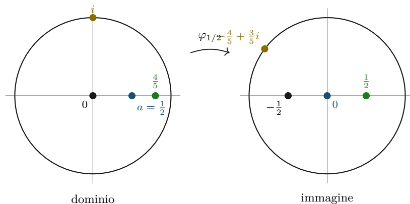
Figura 15.2: Il fattore di Blaschke \varphi_{1/2}(z) = \frac{z - \frac{1}{2}}{1 - \frac{1}{2}z} . Coordinate calcolate a mano: \varphi_{1/2}(\frac{1}{2}) = 0 ; \varphi_{1/2}(0) = \frac{-1/2}{1} = -\frac{1}{2} ; \varphi_{1/2}(\frac{4}{5}) = \frac{4/5 - 1/2}{1 - 2/5} = \frac{3/10}{3/5} = \frac{1}{2} ; \varphi_{1/2}(i) = \frac{i - \frac{1}{2}}{1 - \frac{i}{2}} = \frac{(i - \frac{1}{2})(1 + \frac{i}{2})}{1 + \frac{1}{4}} = \frac{-1 + \frac{3}{4}i}{5/4} = -\frac{4}{5} + \frac{3}{5}i , di modulo \sqrt{\frac{16}{25} + \frac{9}{25}} = 1 , coerentemente con il Lemma 15.10(ii). ✓ Il punto i resta sul bordo, i punti interni restano interni, e a va nel centro.
