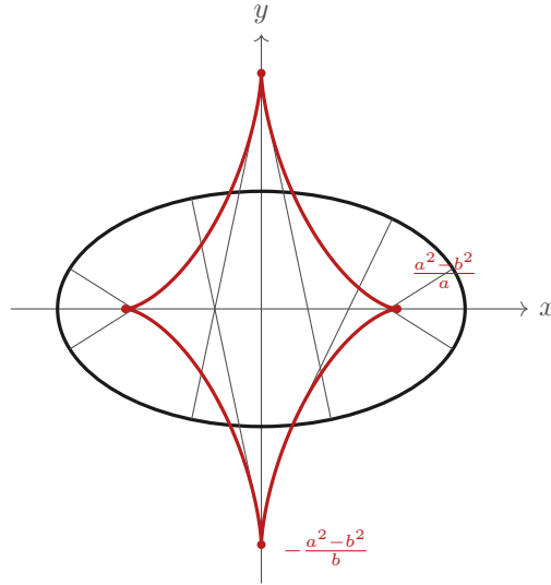
Figura 2.2: L'evoluta dell'ellisse, cioè il luogo dei centri dei cerchi osculatori, di equazioni parametriche X = \frac{a^2-b^2}{a} \cos^3 t , Y = -\frac{a^2-b^2}{b} \sin^3 t : è un'astroide dilatata. Le rette sottili sono le normali all'ellisse, e l'evoluta ne è l'inviluppo: ogni normale la tocca nel centro di curvatura del punto da cui parte. I quattro punti angolosi (cuspidi) corrispondono ai quattro vertici dell'ellisse, cioè ai punti di curvatura stazionaria: sono esattamente i quattro previsti dal teorema dei quattro vertici. Si noti che l'evoluta esce dall'ellisse lungo l'asse minore, perché il raggio di curvatura nei vertici (0, \pm b) vale a^2/b = 4,507 > b .
