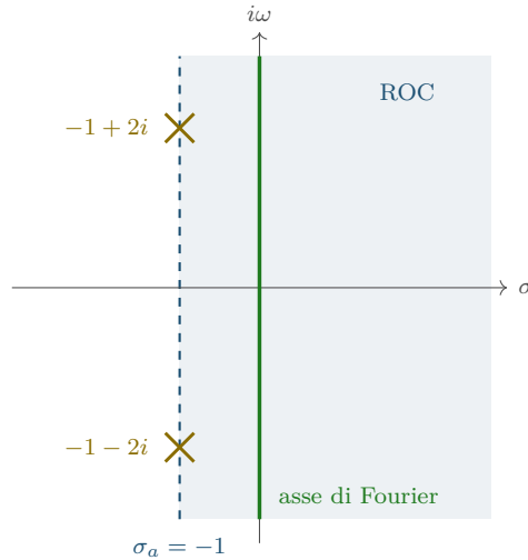
Figura 20.2: Mappa dei poli e regione di convergenza di e^{-t} \cos(2t) u(t) , la cui trasformata è \frac{s+1}{(s+1)^2+4} (Corollario 20.8 con c = 1 , \omega = 2 ). I due poli sono s = -1 \pm 2i (croci ocra), la ROC è il semipiano aperto \text{Re}(s) > -1 (azzurro), e l'asse immaginario (verde) le appartiene: per il Teorema 20.19 il segnale ha allora anche trasformata di Fourier, ottenuta ponendo s = i\omega . Coordinate verificate: annullando (s+1)^2 + 4 si ottiene s+1 = \pm 2i .
