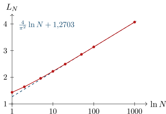
Figura 17.2: Le costanti di Lebesgue L_N (punti, calcolati per quadratura) in funzione di \ln N , con la retta asintotica \frac{4}{\pi^2} \ln N + 1,2703 (tratteggiata). Ascisse: x = 0,8 \ln N centimetri; ordinate: y = 1,2 (L_N - 1) centimetri. La crescita è lineare in \ln N : è il contenuto del Teorema 17.10.
