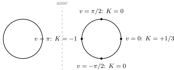
Figura 10.2: Sezione assiale del toro T_{2,1} : due circonferenze di raggio b = 1 con centri a distanza a = 2 dall'asse. La curvatura gaussiana K = \cos v / (b(a + b \cos v)) vale +1/3 = 0,333333 sull'equatore esterno, 0 sulle due circonferenze estreme e -1 = -1/(1 \cdot 1) sull'equatore interno (Proposizione 10.7); il suo integrale sull'intero toro è nullo (Corollario 10.2). Coordinate calcolate a mano: centri (\pm 2, 0) , raggio 1, punti notevoli (3, 0) , (1, 0) , (2, \pm 1) .
