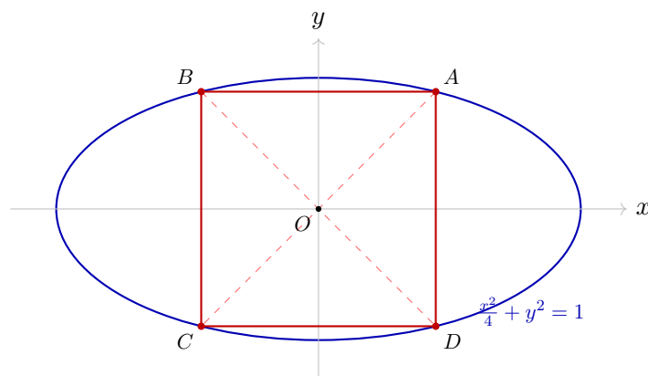
Figura 32.1: Il quadrato inscritto nell'ellisse x^2/4 + y^2 = 1 costruito nell'Esempio 32.1: i vertici sono (\pm 2/\sqrt{5}, \pm 2/\sqrt{5}) = (\pm 0,8944272, \pm 0,8944272) , il centro è l'origine, il lato vale 4/\sqrt{5} = 1,7888544 . Le coordinate sono calcolate a mano e verificate per sostituzione nell'equazione dell'ellisse.
