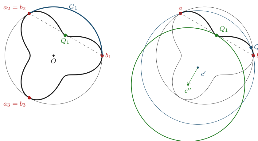
Figura 4.3: La dimostrazione sulla curva r = 1 + 0,35 \cos 3\theta (non convessa: k scende a -5,92 nelle rientranze). A sinistra: il cerchio circoscritto minimo ha raggio R = 1,35 e tre punti di contatto, a 0^\circ , 120^\circ , 240^\circ , dove k = 2,469 \geq 1/R = 0,741 ; le tre lacune hanno ampiezza 120^\circ \leq 180^\circ . A destra, la lacuna G_1 da b ad a : la circonferenza C' per b , a e il punto Q della curva a 10^\circ ha raggio R' = 1,576 > R e centro c' = (-0,191; -0,331) ; traslata nella direzione -\nu di t^* = 0,544 tocca per l'ultima volta l'arco \alpha' nel punto Q_1 a 60^\circ , dove k(Q_1) = -5,92 \leq 1/R' = 0,634 < 1/R , e il suo centro c'' sta dalla parte della normale interna ( \langle n_c, N \rangle = 1 ). La curva ha esattamente 6 = 2 \cdot 3 vertici, a 0^\circ, 60^\circ, \dots, 300^\circ . Valori calcolati a mano e con uno script indipendente.
