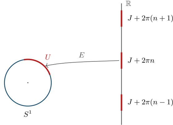
Figura 12.2: L'intorno uniformemente rivestito. Sopra l'arco aperto U \subset S^1 (in rosso sul cerchio) la controimmagine E^{-1}(U) è l'unione disgiunta di infiniti intervalli aperti J + 2\pi n , n \in \mathbb{Z} (i segmenti rossi sulla retta), ciascuno mandato omeomorficamente su U da E . È la «pila di piatti» di Munkres: la retta si avvolge sul cerchio con passo 2\pi , e localmente l'avvolgimento è invertibile. L'inversa locale è la sezione \psi_j + 2\pi n del Lemma 12.2.
