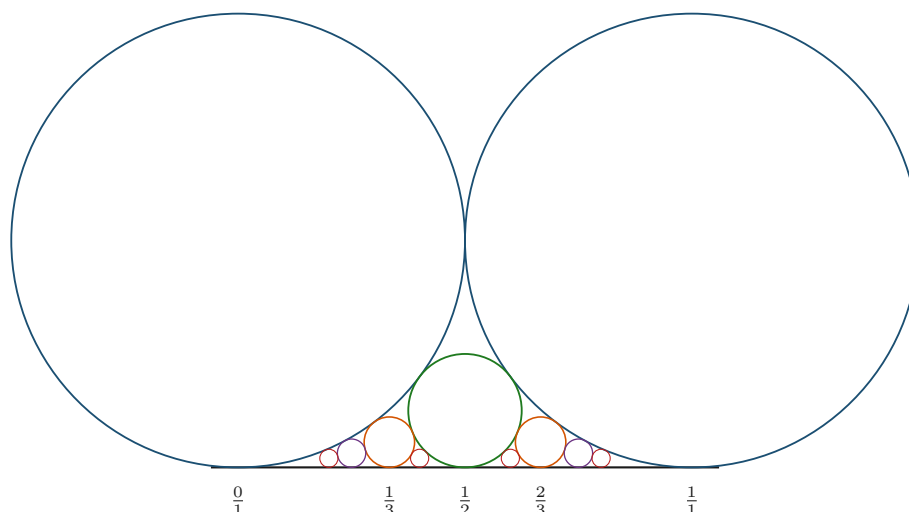
Figura 14.1: I cerchi di Ford delle frazioni di F_5 nell'intervallo [0, 1] . Il cerchio di p/q ha centro (p/q, 1/(2q^2)) e raggio 1/(2q^2) : raggio 0,5 per q = 1 , 0,125 per q = 2 , 1/18 = 0,05556 per q = 3 , 1/32 = 0,03125 per q = 4 , 0,02 per q = 5 . Due cerchi si toccano esattamente quando le frazioni sono vicine di Farey (Teorema 14.2); per esempio \frac{1}{3} e \frac{1}{2} ( |ps - rq| = 1 ) si toccano, mentre \frac{1}{3} e \frac{2}{3} ( |ps - rq| = 3 ) restano lontani. Nessuna coppia si sovrappone mai.
