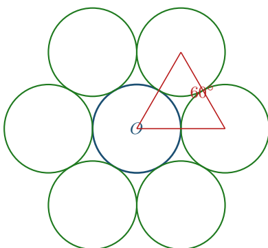
Figura 14.2: Il numero di bacio del piano vale 6. I sei centri stanno sui vertici di un esagono regolare di lato 2 inscritto nel cerchio di raggio 2: coordinate (\pm 2, 0) e (\pm 1, \pm 1,73205) . Il triangolo rosso ha i tre lati di lunghezza 2 ( |(2, 0) - (1, \sqrt{3})|^2 = 1 + 3 = 4 ), dunque è equilatero e l'angolo al centro è esattamente 60^\circ : sei angoli di 60^\circ riempiono il giro senza avanzo, e un settimo cerchio richiederebbe un altro angolo \geq 60^\circ (Teorema 14.3, Passo 2).
