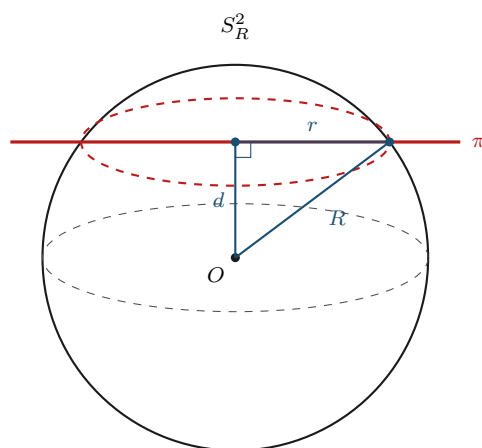
Figura 7.2: La sezione piana di una sfera è sempre un cerchio. Se il piano \pi dista d < R dal centro O , il triangolo rettangolo di cateti d e r e ipotenusa R dà immediatamente r = \sqrt{R^2 - d^2} : il raggio della sezione dipende solo dalla distanza del piano dal centro, non dalla sua giacitura. Per d = 0 si ottiene il cerchio massimo ( r = R ), per d \rightarrow R il cerchio si riduce a un punto. È la stessa relazione della corda di un cerchio del Volume I, trasportata di una dimensione.
