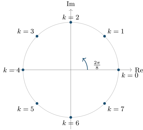
Figura 22.1: I punti \omega_8^{-k} = e^{2\pi i k/8} , k = 0, \dots, 7 , sui quali la DFT a otto punti valuta il polinomio \sum_n x[n]z^{-n} (Teorema 22.12). Le coordinate sono (\cos(2\pi k/8), \sin(2\pi k/8)) : (\pm 1, 0) , (0, \pm 1) e i quattro punti di coordinate \pm\sqrt{2}/2 = \pm 0,70711 , calcolate a mano da \cos(\pi/4) = \sin(\pi/4) = \sqrt{2}/2 e ricontrollate numericamente.
