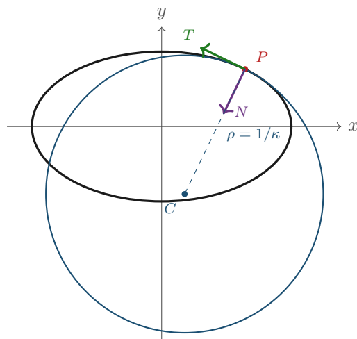
Figura 2.1: Il riferimento di Frenet e il cerchio osculatore in un punto P dell'ellisse x^2/a^2 + y^2/b^2 = 1 con a = 2,6 , b = 1,5 . Il versore tangente T e il versore normale N formano una base ortonormale mobile; il cerchio osculatore ha centro C = P + \rho N sulla normale interna e raggio \rho = 1/\kappa . Qui \kappa = 0,360 e \rho = 2,779 . Il cerchio osculatore è l'unico cerchio che ha con la curva un contatto del secondo ordine: fra tutti i cerchi tangenti in P , è quello che ne riproduce anche la curvatura.
