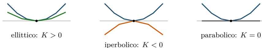
Figura 10.1: Sezioni normali nelle due direzioni principali. Le ordinate sono calcolate a mano dalle parabole y = 0,5x^2 (nodi 0,72; 0,32; 0,08; 0), y = 0,25x^2 (nodi 0,36; 0,09; 0) e y = -0,4x^2 (nodi -0,576; -0,144; 0). Nel punto ellittico le due sezioni stanno dalla stessa parte del piano tangente, in quello iperbolico da parti opposte, in quello parabolico una delle due è rettilinea (Proposizione 10.5).
