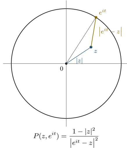
Figura 16.2: La geometria del nucleo di Poisson. Coordinate calcolate a mano: z = 0,45 + 0,30i , dunque |z|^2 = 0,2025 + 0,09 = 0,2925 e 1 - |z|^2 = 0,7075 ; t = 1 radiante dà e^{it} = 0,5403023 + 0,8414710i , dunque e^{it} - z = 0,0903023 + 0,5414710i e |e^{it} - z|^2 = 0,0081545 + 0,2931908 = 0,3013453 . Quindi P(z, e^{it}) = 0,7075/0,3013453 = 2,3478047 . Controllo indipendente con la forma polare del Lemma 16.4: |z| = 0,5408327 , \arg z = \arctan(0,30/0,45) = 0,5880026 , e P_{|z|}(\arg z - t) = \frac{0,7075}{1 - 2 \cdot 0,5408327 \cos(0,4119974) + 0,2925} = 2,3478047 . ✓
