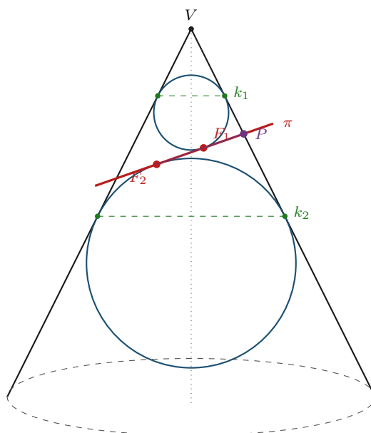
Figura 7.1: Le sfere di Dandelin, viste nella sezione assiale del cono. Le due sfere sono inscritte nel cono (in sezione: i due cerchi tangenti a entrambe le generatrici) e tangenti al piano secante \pi (in rosso). I punti di tangenza F_1 e F_2 sono i fuochi della conica sezione; le circonferenze k_1, k_2 lungo cui le sfere toccano il cono determinano le direttrici. Per un punto P della conica, i segmenti PF_1 e PF_2 hanno la stessa lunghezza dei segmenti di generatrice compresi fra P e k_1, k_2 : da qui PF_1 + PF_2 = \overline{k_1 k_2} costante, cioè l'ellisse.
