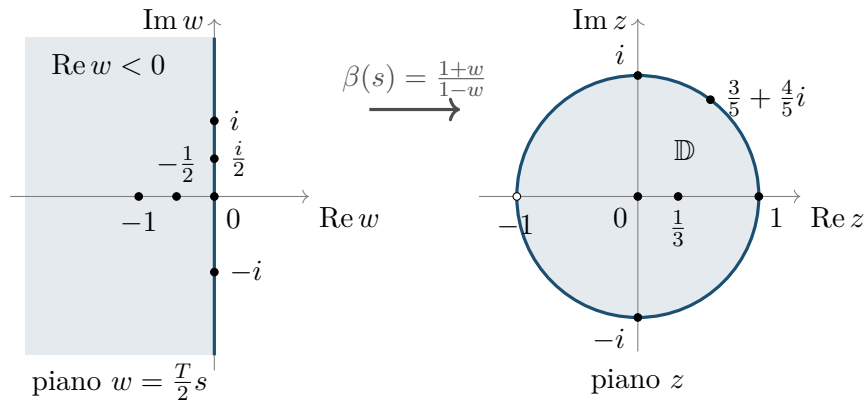
Figura 21.2: La trasformazione bilineare del Teorema 21.14: il semipiano sinistro va sul disco unitario, l'asse immaginario sul cerchio unitario privato di -1 (cerchietto vuoto). Le corrispondenze disegnate sono esatte: 0 \mapsto 1 , -\frac{1}{2} \mapsto \frac{1}{3} , -1 \mapsto 0 , \frac{i}{2} \mapsto \frac{3}{5} + \frac{4}{5}i , \pm i \mapsto \pm i ; e infatti \frac{1+i/2}{1-i/2} = \frac{(1+i/2)^2}{5/4} = \frac{3/4+i}{5/4} = \frac{3}{5} + \frac{4}{5}i , di modulo 1. Il raggio del disco è 1,6 cm e i punti sono collocati moltiplicando per 1,6 le coordinate esatte.
