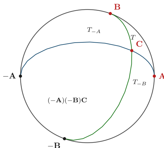
Figura 8.3: Il Passo 2 della dimostrazione del teorema di Girard, visto in proiezione ortografica sulla semisfera H delimitata dal cerchio massimo \gamma_c per \mathbf{A} e \mathbf{B} (il bordo del disco). I due archi disegnati sono le metà di \gamma_b (in blu, da \mathbf{A} a -\mathbf{A} per \mathbf{C} ) e di \gamma_a (in verde, da \mathbf{B} a -\mathbf{B} per \mathbf{C} ). Essi tagliano H nei quattro triangoli T , T_{-A} , T_{-B} e (-\mathbf{A})(-\mathbf{B})\mathbf{C} . I punti sono calcolati con \mathbf{A} sull'equatore a longitudine 0^\circ , \mathbf{B} sull'equatore a longitudine 70^\circ , \mathbf{C} a latitudine 40^\circ e longitudine 30^\circ , e la proiezione è (x, y, z) \mapsto (3x, 3y) .
