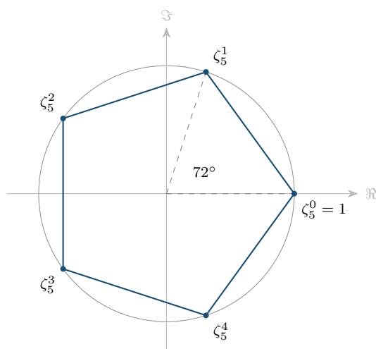
Figura 6.1: Le cinque radici quinte dell'unità e il pentagono regolare che ne è l'involuppo convesso. Le coordinate dei vertici sono (\cos(72k)^\circ, \sin(72k)^\circ) per k = 0, \dots, 4 , cioè (1; 0) , (0,30902; 0,95106) , (-0,80902; 0,58779) , (-0,80902; -0,58779) , (0,30902; -0,95106) ; il lato misura 2 \sin 36^\circ = 1,17557 (Teorema 6.3(ii)) e l'angolo interno 108^\circ .
