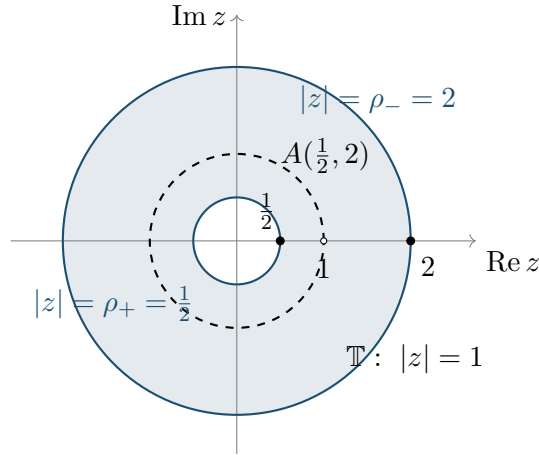
Figura 21.1: La regione di convergenza di x[n] = (\frac{1}{2})^n u[n] - 2^n u[-n-1] : la corona A(\frac{1}{2}, 2) del Teorema 21.1. Il bordo interno è dettato dalla parte causale, quello esterno dalla parte anticausale, e i due poli di X(z) = \frac{z}{z-1/2} + \frac{z}{z-2} stanno esattamente sulle due circonferenze. Poiché \rho_+ = \frac{1}{2} < 1 < 2 = \rho_- , il cerchio unitario \mathbb{T} (tratteggiato) è contenuto nella corona: il segnale è sommabile e ha DTFT.
