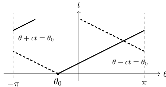
Figura 18.2: Le caratteristiche \theta \pm ct = \text{cost} nella striscia \mathbb{T} \times [0, +\infty) per c = 2 e \theta_0 = -1 . Coordinate calcolate a mano: la caratteristica destra \theta = \theta_0 + ct raggiunge \theta = \pi al tempo t = (\pi - \theta_0)/c = (3,1415927 + 1)/2 = 2,0707963 e rientra da \theta = -\pi ; quella sinistra \theta = \theta_0 - ct raggiunge \theta = -\pi al tempo t = (\theta_0 + \pi)/c = (3,1415927 - 1)/2 = 1,0707963 e rientra da \theta = \pi . Al tempo t = 2\pi/c = \pi entrambe sono tornate al punto di partenza: è la Proposizione 18.8.
