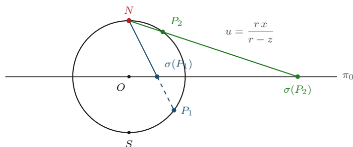
Figura 7.4: La proiezione stereografica, vista nella sezione assiale della sfera unitaria ( r = 1 ). Il punto P_1 = (0,8, 0, -0,6) dell'emisfero australe si proietta in \sigma(P_1) = (0,5, 0) , dentro il cerchio equatoriale, perché u = x/(1 - z) = 0,8/1,6 = 0,5 ; il punto P_2 = (0,6, 0, 0,8) dell'emisfero boreale si proietta in \sigma(P_2) = (3, 0) , molto lontano, perché u = 0,6/0,2 = 3 . L'equatore resta fisso punto per punto, e avvicinandosi al polo N l'immagine fugge all'infinito: è la ragione per cui N corrisponde al punto all'infinito della sfera di Riemann.
