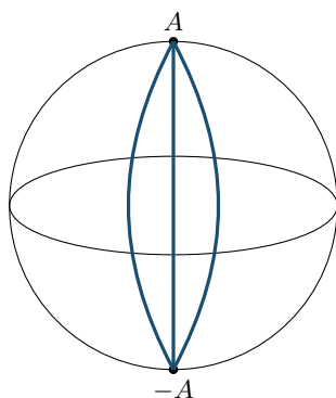
Figura 9.3: Il punto coniugato. Tutte le geodetiche uscenti da A — i meridiani — si riincontrano nell'antipodo -A dopo lunghezza \pi r , indipendentemente dalla direzione iniziale (Proposizione 9.5). Prima di -A ciascun arco è il cammino più breve; oltre -A nessuno lo è più (Teorema 9.5).
