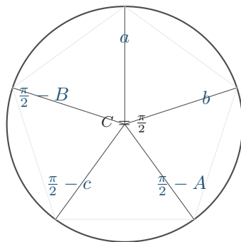
Figura 8.2: Il pentagono delle parti circolari di Napier per un triangolo rettangolo in C . L'angolo retto non compare; le cinque parti circolari sono, nell'ordine ciclico in cui si presentano sul triangolo, a , b , \frac{\pi}{2} - A , \frac{\pi}{2} - c , \frac{\pi}{2} - B . I vertici del pentagono regolare sono calcolati a mano su un cerchio di raggio 2,2: (0; 2,2) , (2,2 \cos 18^\circ; 2,2 \sin 18^\circ) = (2,0923; 0,6798) , (2,2 \cos(-54^\circ); 2,2 \sin(-54^\circ)) = (1,2931; -1,7798) e i due simmetrici rispetto all'asse verticale.
