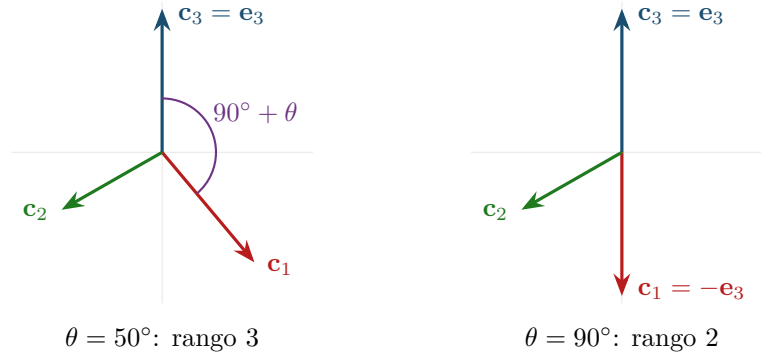
Figura 28.3: Il gimbal lock come collasso di due colonne dello jacobiano. Con \psi = 0 le colonne di J sono \mathbf{c}_1 = (\cos \theta, 0, -\sin \theta)^\top , \mathbf{c}_2 = (0, 1, 0)^\top e \mathbf{c}_3 = (0, 0, 1)^\top : la prima e la terza stanno nel piano xz (qui il piano del foglio, con z verso l'alto), la seconda esce dal foglio ed è disegnata obliqua. L'angolo fra \mathbf{c}_1 e \mathbf{c}_3 vale 90^\circ + \theta : a \theta = 50^\circ è 140^\circ e le tre colonne sono indipendenti; a \theta = 90^\circ è 180^\circ , cioè \mathbf{c}_1 = -\mathbf{c}_3 , e il rango scende a 2. Le coordinate disegnate a \theta = 50^\circ sono 2 \cos 50^\circ = 1,2856 e -2 \sin 50^\circ = -1,5321 .
