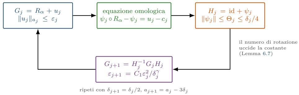
Figura 6.3: Lo schema di Newton come diagramma a blocchi: a ogni giro l'errore passa da \varepsilon_j a C_1 \varepsilon_j^2 / \delta_j^\gamma (quadratico) e la striscia da a_j ad a_j - 3\delta_j (perdita sommabile). Il passaggio dal blocco in alto a destra a quello in basso usa il Lemma 6.7, cioè l'ipotesi \rho(F) = \rho : è l'unico punto in cui il numero di rotazione entra nella dimostrazione. Figura a mano, senza dati numerici.
