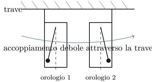
Figura 13.3: Schema del dispositivo di Huygens (1665, Osservazione 13.2, livello A): due orologi a pendolo appesi a una stessa trave, sostenuta da due sedie; il pendolo di sinistra è disegnato in un istante in cui i due pendoli sono quasi in opposizione di fase, il regime che Huygens osservò stabilirsi entro circa mezz'ora indipendentemente dalle condizioni iniziali.
