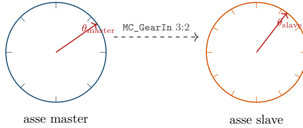
Figura 14.7: Schema qualitativo (non in scala) di MC_GearIn: due assi modulo (due copie di S^1 , otto tacche sul master e dodici sullo slave, nel rapporto 3:2) sincronizzati da un blocco funzione PLCopen; l'angolo dello slave è una funzione lineare (coniugazione) di quello del master, \theta_{\text{slave}} = \frac{3}{2}\theta_{\text{master}} + c .
