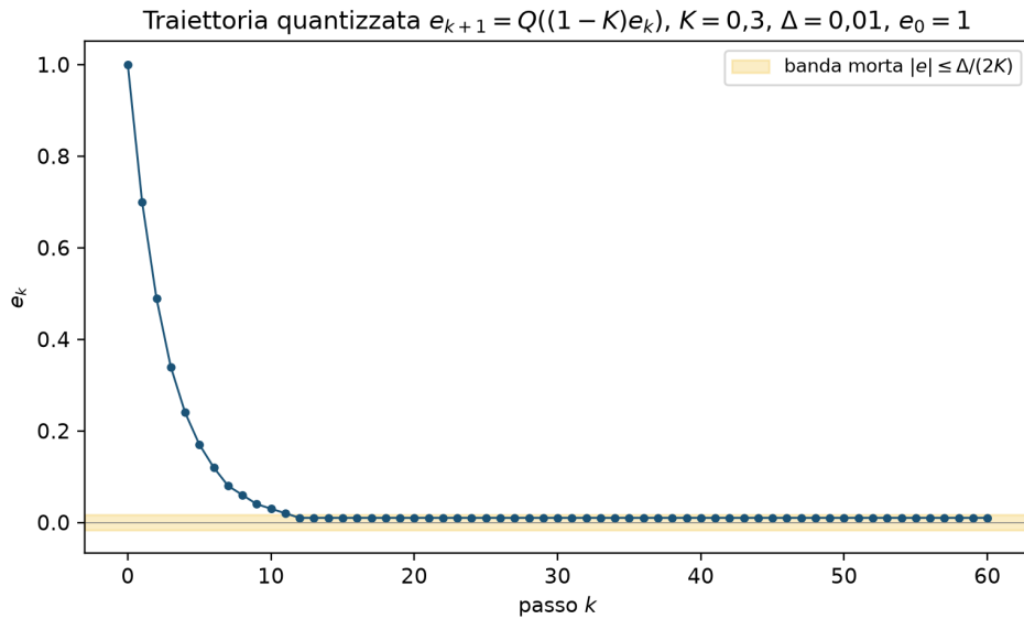
Figura 14.6: Traiettoria quantizzata e_{k+1} = Q_\Delta((1-K)e_k) per K = 0,3 , \Delta = 0,01 , e_0 = 1 : |e_k| decresce (Teorema 14.4(ii)) fino a raggiungere, al passo k = 12 , il punto fisso esatto e_\infty = 0,01 , dentro la banda morta teorica |e| \leq \Delta/(2K) = 0,0167 (zona ombreggiata). Calcolata numericamente con doppio controllo (ricorsione reale e ricorsione intera ridotta, Passo 0 della dimostrazione); script fig14_banda_morta.py , Appendice B. ✓
