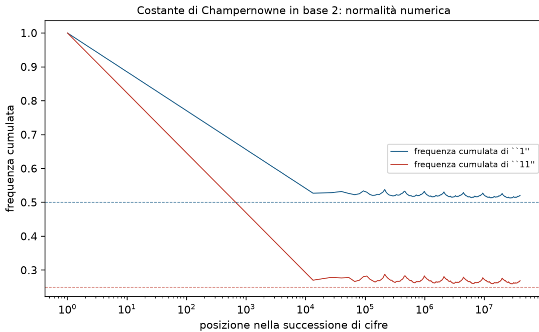
Figura 9.3: Frequenza cumulata (asse N in scala logaritmica) della cifra “1” (blu, attesa 1/2 ) e del blocco “11” (rosso, atteso 1/4 ) nelle cifre binarie della costante di Champernowne, concatenazione delle rappresentazioni binarie di 1, 2, 3, \dots, 2\,000\,000 (39 902 870 cifre in tutto). La convergenza verso le rette tratteggiate è presente ma lenta, come discusso nell’Esempio 9.2. Calcolata numericamente, script fig09_champernowne_binario.py (Appendice B), eseguito il 16 settembre 2026. ✓
