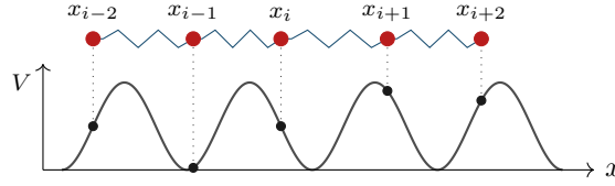
Figura 16.2: La catena di Frenkel–Kontorova (Osservazione 16.3): atomi (pallini rossi) collegati da molle armoniche e immersi nel potenziale periodico V(x) = 0,35 - 0,35 \cos(2\pi x) di periodo 1 (curva grigia; i pallini neri sono le proiezioni degli atomi sul potenziale). Le ascisse disegnate, 0,25; 1,05; 1,75; 2,60; 3,35, danno ordinate 0,350; 0,017; 0,350; 0,633; 0,556 rispettivamente. La competizione fra l’energia elastica, che vorrebbe spaziature uguali, e l’energia di substrato, che vorrebbe ogni atomo in un minimo di V , è esattamente la competizione fra i due termini dell’azione W .
