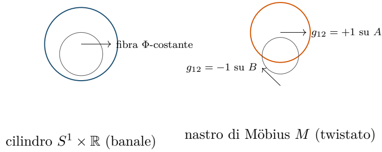
Figura 2.2: I due fibrati in rette reali su S^1 (Teorema 2.7, n = 1 ): il cilindro banale e il nastro di Möbius, distinti dalla monodromia \pm 1 (Teorema 2.4).
