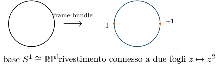
Figura 2.11: Il frame bundle (riferimenti ortonormali) del nastro di Möbius è il rivestimento connesso a due fogli p_2(z) = z^2 del Capitolo 1: i due riferimenti \pm 1 si scambiano lungo la monodromia (Esempio Svolto 2.4, Sezione 2.17).
