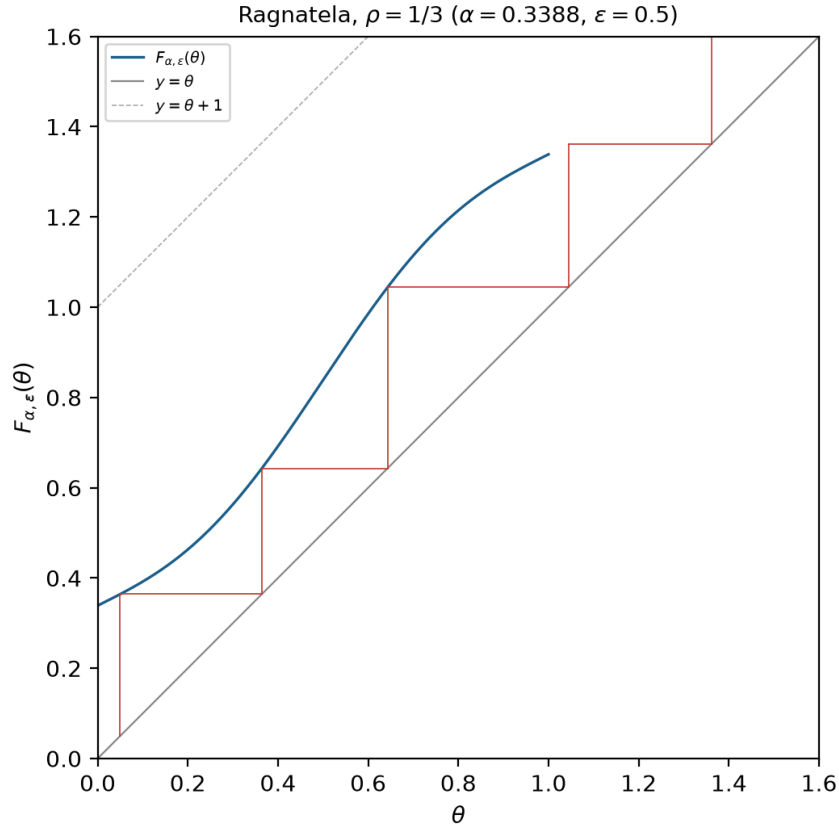
Figura 4.5: Diagramma a ragnatela per f_{\alpha, \varepsilon} con \varepsilon = 0,5 e \alpha = 0,338781 (centro della lingua 1/3 , individuato per bisezione), generato dallo script Sorgenti/Vol4/appendiceB_laboratorio/fig04_ragnatela_rho13.py (eseguito il 16 settembre 2026): la traiettoria (rossa) a partire da \theta_0 = 0,05 converge in poche iterazioni all'orbita attrattiva di periodo 3 \{0,996545, 0,337053, 0,607866\} . Controllo: F^3(\theta^*) - \theta^* - 1 = 0 a precisione macchina \checkmark (Teorema 4.3 con p = 1, q = 3 ).
