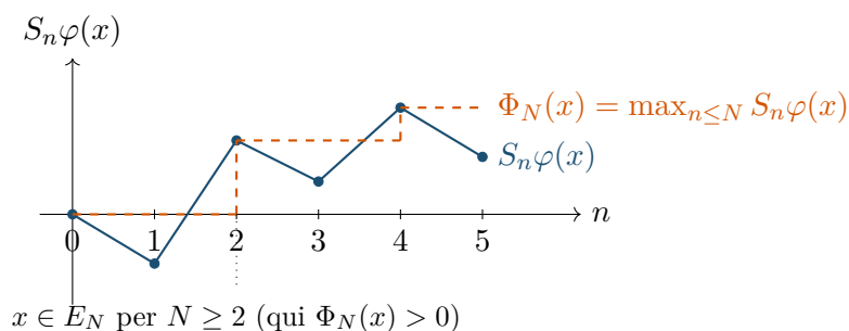
Figura 9.1: Schema del “trucco” di Garsia (Teorema 9.6): un percorso illustrativo dei valori S_n \varphi(x) , n = 0, \dots, 5 (blu, valori 0, -0,6, 0,9, 0,4, 1,3, 0,7 ) e la successione crescente del massimo parziale \Phi_N(x) = \max_{0 \leq n \leq N} S_n \varphi(x) (arancio tratteggiato, a gradini: 0, 0, 0,9, 0,9, 1,3, 1,3 ): il punto x appartiene a E_N = \{\Phi_N > 0\} non appena la successione ha toccato un valore positivo, qui a N = 2 . Figura a mano, schematica (un solo percorso illustrativo, non dati numerici); coordinate verificate nel testo.
