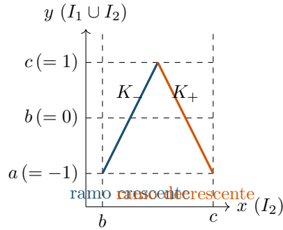
Figura 8.2: Il ferro di cavallo dentro I_2 = [b, c] generato da un'orbita di periodo 3: f|_{I_2} ha due rami monotoni K_- , K_+ (qui rappresentati in modo schematico, coordinate normalizzate I_2 \rightarrow [0, 2] , I_1 \cup I_2 \rightarrow [-1, 1] ), ciascuno dei quali ricopre l'intero I_1 \cup I_2 . Il ricoprimento a due rami è esattamente la struttura di un ferro di cavallo di Smale unidimensionale, e produce un'immersione dello shift pieno a 2 simboli: h_{\text{top}}(f) \geq \log 2 (Teorema 8.9). Figura a mano; coordinate verificate: i due segmenti hanno pendenza \pm 2 e uniscono (0, -1) – (1, 1) – (2, -1) , coerenti con f(K_-) = f(K_+) = I_1 \cup I_2 .
