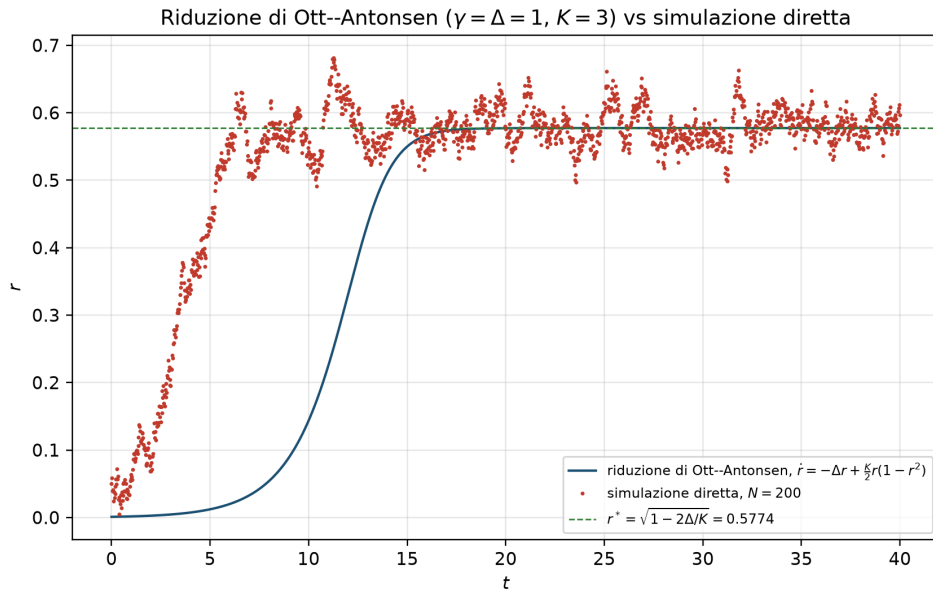
Figura 13.7: Riduzione di Ott–Antonsen ( \Delta = \gamma = 1 , K = 3 > K_c = 2 , Teorema 13.6): integrazione Runge–Kutta 4 dell’equazione ridotta \dot{r} = -\Delta r + \frac{K}{2}r(1-r^2) da r(0) = 10^{-3} (curva blu), a confronto con la simulazione diretta dei medesimi N = 200 oscillatori lorentziani della Figura 13.5 (punti rossi). Il punto fisso in forma chiusa r^* = \sqrt{1 - 2\Delta/K} = 0,577350 (retta tratteggiata verde) è raggiunto dall’integrazione numerica dell’ODE ridotta entro 9,0 \times 10^{-10} ✓, e coincide esattamente (entro 10^{-12} ) con il valore teorico dell’autoconsistenza \sqrt{1 - K_c/K} del Corollario 13.3 (Osservazione 13.5) ✓; la simulazione diretta a N = 200 converge a r \approx 0,5813 , con lo scarto 0,0039 atteso dalle fluttuazioni di taglia finita. Calcolata numericamente, script Appendice B, fig13_ott_antonsen.py.
