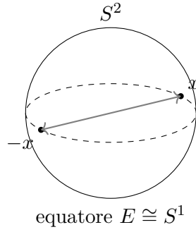
Figura 1.3: Il teorema di Borsuk–Ulam (forma BU1): esiste x \in S^2 con f(x) = f(-x) ; nella dimostrazione la restrizione all’equatore E \cong S^1 trasporta la questione al grado di una mappa dispari S^1 \rightarrow S^1 . Coordinate del punto x : \cos 35^\circ = 0,819 , \sin 35^\circ = 0,574 .
