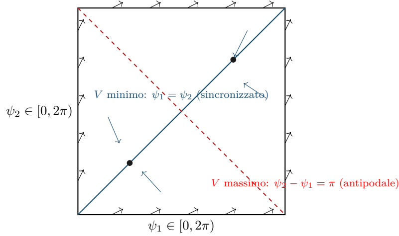
Figura 13.4: Il potenziale V(\psi_1, \psi_2) = -K \cos(\psi_1 - \psi_2) (Lemma 13.1 con N = 2 ) sul toro \mathbb{T}^2 = [0, 2\pi)^2 con i lati opposti identificati: la diagonale \psi_1 = \psi_2 (blu) è la varietà dei minimi globali (stato sincronizzato, Teorema 13.4), l'antidiagonale \psi_2 - \psi_1 = \pi (rossa, tratteggiata) è la varietà dei massimi (equilibrio instabile della Proposizione 13.1); le frecce blu indicano il flusso gradiente -\nabla V , che porta ogni orbita (tranne quelle che partono esattamente sull'antidiagonale) verso la diagonale.
