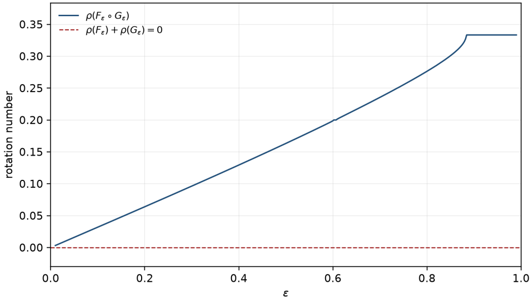
Figura 15.2: Il difetto del quasi-morfismo, calcolato numericamente: la curva è \varepsilon \mapsto \rho(F_\varepsilon \circ G_\varepsilon) per la coppia dell'Esempio 15.1, mentre la retta tratteggiata è \rho(F_\varepsilon) + \rho(G_\varepsilon) = 0 , valore esatto perché entrambe le mappe hanno un punto fisso. Lo scarto fra le due curve è il difetto di additività: nullo solo nel limite \varepsilon \rightarrow 0^+ (dove entrambe le mappe tendono all'identità), pari a 0,080053 per \varepsilon = 0,25 , a 0,163239 per \varepsilon = 0,50 , a 0,255189 per \varepsilon = 0,75 e a 1/3 esatto per \varepsilon = 0,90 (orbita periodica di tipo (1, 3) , Esempio 15.1(5)). La curva ha la struttura di una scala del diavolo: oltre al lungo gradino finale a quota 1/3 se ne vede uno molto più corto a quota 1/5 , che il blocco [C15-1] localizza per \varepsilon \in [0,6020, 0,6070] cercando le orbite periodiche di tipo (1, 5) con passo 0,001 ✓. Script fig15_quasimorfismo.py , Appendice B; 400 valori di \varepsilon , 2,4 \times 10^5 iterazioni ciascuno, scarto massimo fra N e 2N iterazioni pari a 1,3 \times 10^{-6} .
