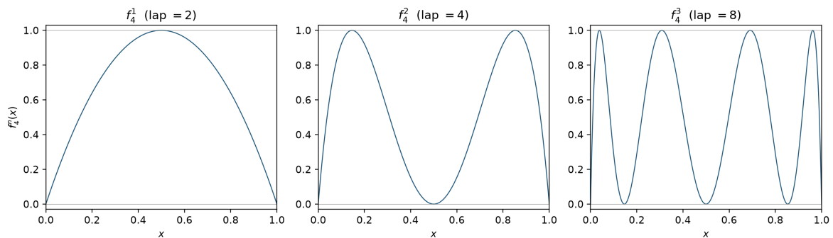
Figura 8.1: Grafici di f_4^n per n = 1, 2, 3 sull’intervallo [0, 1] , con il numero di tratti di monotonia (lap number) verificato per conteggio dei cambi di segno della derivata discreta: 2, 4, 8, esattamente 2^n . Calcolata numericamente, script fig08_lap_number.py (Appendice B), eseguito il 16 settembre 2026. ✓
