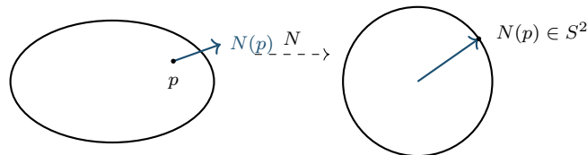
Figura 2.8: La mappa di Gauss N : \Sigma \rightarrow S^2 (Osservazione 2.10): il vettore normale unitario in p visto come punto di S^2 .
