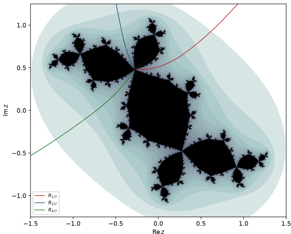
Figura 12.5: I tre raggi esterni di angoli 1/7 , 2/7 , 4/7 — un'orbita periodica di periodo 3 della mappa raddoppiante, 1/7 \mapsto 2/7 \mapsto 4/7 \mapsto 8/7 \equiv 1/7 — sul coniglio di Douady K_c con c = -0,1225611669 + 0,7448617666i . I tre raggi atterrano nello stesso punto \alpha , il punto fisso repulsivo dove si toccano le tre «orecchie». Costruzione dello script fig12_julia.py (Appendice B, 17 settembre 2026): il punto di R_t a potenziale s si ottiene risolvendo con Newton g_c^n(z) = \exp(s 2^n) e^{2\pi i(2^n p \bmod q)/q} , con n scelto in modo che il potenziale d'arrivo sia circa 12 (l'angolo raddoppiato è calcolato con interi esatti, non in virgola mobile). Controlli: i due punti fissi sono z_+ = 1,2763376236 - 0,4797279843i (moltiplicatore di modulo 2,727) e \alpha = z_- = -0,2763376236 + 0,4797279843i (moltiplicatore di modulo 1,10725141 e argomento 0,33317563 giri, cioè circa 1/3 : il numero di rotazione del bulbo, Osservazione 12.8); al potenziale finale 2,9 \times 10^{-14} i tre raggi distano da \alpha rispettivamente 6,43 \times 10^{-3} , 6,41 \times 10^{-3} , 6,44 \times 10^{-3} . La relazione g_c(R_{1/7}) = R_{2/7} del Teorema 12.9 è verificata su 1100 punti con scarto mediano 7,9 \times 10^{-17} e massimo 1,5 \times 10^{-8} . ✓
