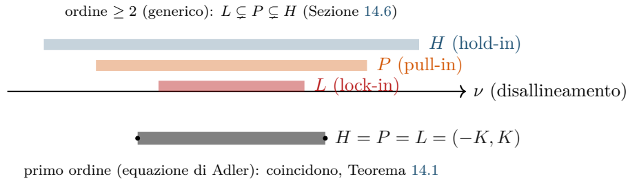
Figura 14.2: Le bande di aggancio come insiemi annidati (Definizione 14.1, Osservazione 14.3): in generale, per un PLL di ordine \geq 2 , L \subsetneq P \subsetneq H (schema qualitativo, non in scala); per il PLL del primo ordine i tre insiemi collassano esattamente sullo stesso intervallo (-K, K) (Teorema 14.1).
