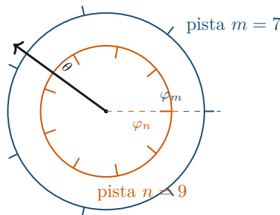
Figura 14.4: Schema (non in scala) di un encoder Vernier/nonio a due piste con m = 7 e n = 9 tacche coprima per giro (l'esempio della Sezione 14.9 e dell'Esempio Svolto 14.3): l'angolo vero \theta genera due letture di fase \varphi_m, \varphi_n (una per pista), la cui combinazione J = (n\varphi_m - m\varphi_n)/2\pi (Costruzione 14.2) determina univocamente \theta entro la tolleranza del Teorema 14.3.
