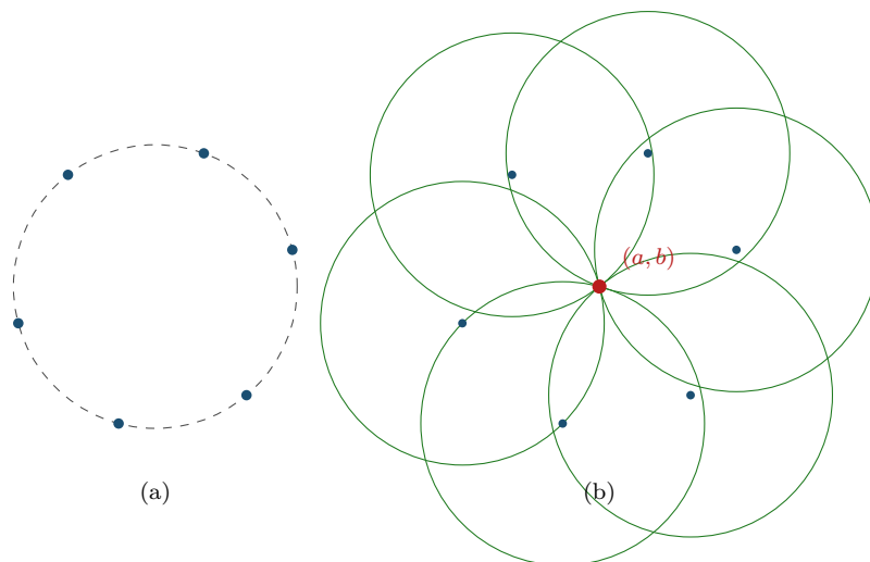
Figura 11.4: La trasformata di Hough per cerchi di raggio noto R . In (a) i punti di bordo rilevati nell'immagine. In (b) lo spazio dei parametri (a, b) : ogni punto (x_i, y_i) dell'immagine è compatibile con tutti i centri che distano R da esso, cioè vota per un intero cerchio di raggio R centrato in (x_i, y_i) . Poiché tutti i punti di bordo appartengono allo stesso cerchio vero, i loro cerchi di voto si intersecano tutti nel centro cercato, che appare come un picco netto dell'accumulatore. Se il raggio non è noto, l'accumulatore diventa tridimensionale (a, b, R) e ogni punto vota su un cono: il costo cresce, ma il principio — trasformare il riconoscimento di forme in una ricerca di massimi — resta lo stesso.
