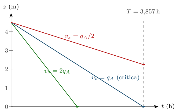
Figura 14.2: Quota verticale z(t) = h - v_s t di tre particelle (Passo 2 della dimostrazione del Teorema 14.1), per l'esempio del testo: la particella critica v_s = q_A tocca il fondo esattamente al tempo di detenzione teorico T (pallino blu su z = 0 ); una particella più veloce lo tocca in anticipo, con margine (pallino verde); una più lenta non ha ancora toccato il fondo quando t = T (pallino rosso, z = 2,25 m).
