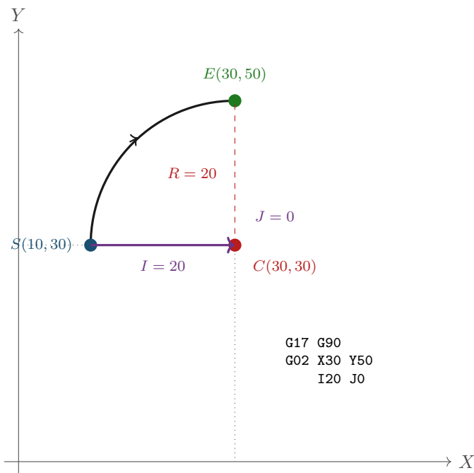
Figura 11.6: L'interpolazione circolare in G-code. Il blocco G02 percorre un arco in senso orario dal punto corrente S al punto E dichiarato con X e Y ; il centro non si dichiara in assoluto ma con gli scostamenti I e J , cioè le componenti del vettore \vec{SC} dal punto iniziale al centro. Qui S = (10, 30) , E = (30, 50) , C = (30, 30) , dunque I = 30 - 10 = 20 e J = 30 - 30 = 0 , e l'arco ha raggio 20. La scelta relativa non è un capriccio: rende il blocco indipendente dall'origine pezzo, sicché lo stesso programma funziona dopo un cambio di zero. Il controllo verifica che S ed E siano equidistanti da C entro una tolleranza, e segnala errore altrimenti.
