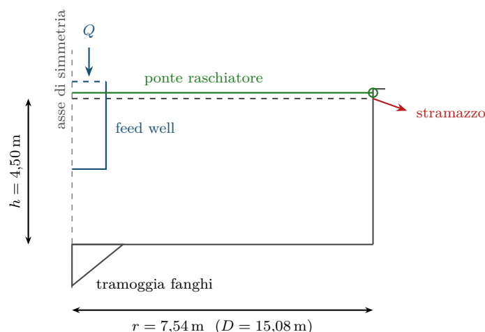
Figura 14.1: Semisezione schematica (non in scala) del chiarificatore dell'Esempio 14.3: alimentazione centrale dal feed well, ponte raschiatore radiale con ruota di sostegno alla periferia, stramazzo perimetrale. La tramoggia dei fanghi al centro non è in scala rispetto al resto della vasca.
