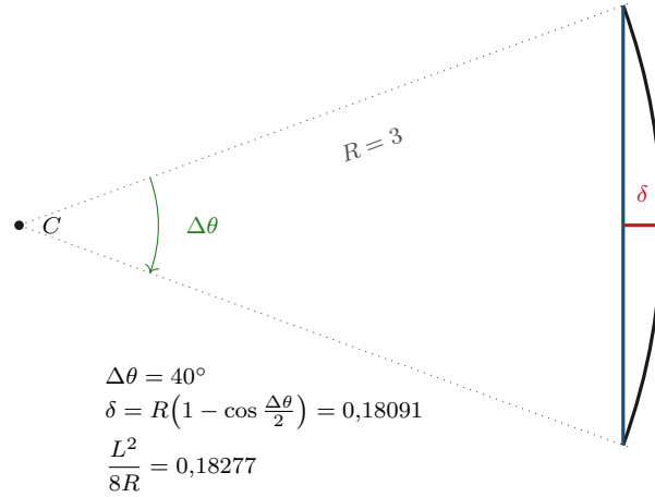
Figura 13.2: L'errore di corda: la ragione per cui un arco eseguito da un controllo numerico non è mai un arco. L'interpolatore approssima l'arco con una spezzata di corde, una per periodo di interpolazione, e la freccia \delta fra corda e arco è l'errore geometrico che ne risulta: \delta = R(1 - \cos \frac{\Delta\theta}{2}) . Nell'esempio ( R = 3 , \Delta\theta = 40^\circ ) si ha \delta = 0,18091 . Sviluppando il coseno in serie si ottiene l'approssimazione di uso pratico \delta \simeq R\Delta\theta^2/8 = L^2/(8R) , con L = R\Delta\theta lunghezza dell'arco percorso in un periodo: qui 0,18277, con uno scarto dell'1%. Poiché L = vT , invertendo si ottiene il vincolo di velocità v \leq \sqrt{8R\delta_{\max}}/T : raddoppiare la velocità quadruplica l'errore di corda.
