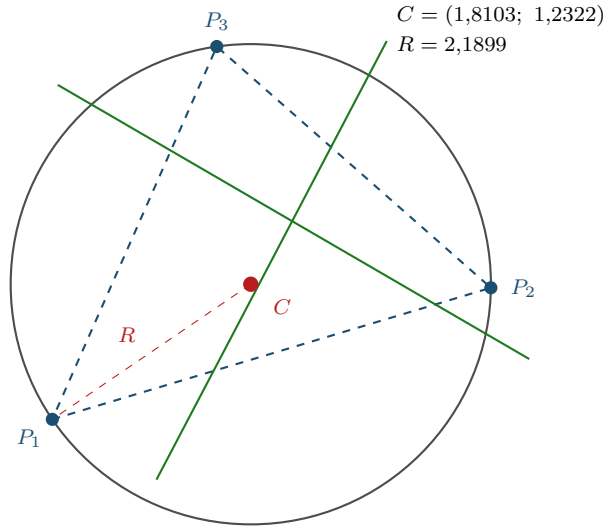
Figura 13.1: Il cerchio per tre punti, primitiva di ogni interpolazione circolare industriale. Il centro è l'intersezione degli assi di due qualunque dei tre segmenti (in verde): imponendo |C - P_1|^2 = |C - P_2|^2 e |C - P_1|^2 = |C - P_3|^2 i termini quadratici si elidono e resta un sistema lineare 2 \times 2 , che ha soluzione unica se e solo se i tre punti non sono allineati. Con P_1 = (0;0) , P_2 = (4;1,2) , P_3 = (1,5;3,4) si ottiene C = (1,8103; 1,2322) e R = 2,1899 . Nello spazio la costruzione è la stessa, eseguita nel piano dei tre punti: si prende il versore normale \mathbf{n} = (P_2 - P_1) \times (P_3 - P_1) normalizzato, si costruisce una base ortonormale del piano e si risolve il problema piano; il condizionamento peggiora quando i punti sono quasi allineati, ed è per questo che i controlli rifiutano gli archi con punti troppo vicini fra loro.
