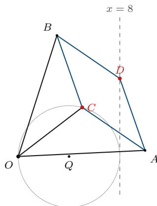
Figura 5.7: L'inversore di Peaucellier-Lipkin con R = 10 , s = 6 , manovella di centro Q = (4, 0) e raggio 4 (grigio), C all'angolo 75^\circ sulla manovella: C \approx (5,035; 3,864) , A \approx (9,989; 0,478) , B \approx (3,047; 9,525) (vertici del rombo ACBD con |OA| = |OB| = 10 , |CA| = |CB| = |DA| = |DB| = 6 , verificato indipendentemente) e D = (8; 6,139) , sempre sulla retta x = 8 come previsto dal Corollario 5.5.
