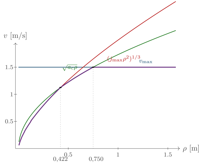
Figura 13.5: La velocità massima ammissibile su un arco, in funzione del raggio di curvatura \rho . Tre vincoli indipendenti agiscono insieme e la velocità effettiva è il loro minimo (in viola). Il vincolo di velocità di targa v_{\max} è costante; quello di accelerazione centripeta dà v \leq \sqrt{a_c \rho} , cioè cresce come \sqrt{\rho} ; quello di strappo ( jerk ), che sul cerchio vale |\dot{a}| = v^3/\rho^2 , dà v \leq (j_{\max} \rho^2)^{1/3} e cresce come \rho^{2/3} . Con v_{\max} = 1,5 m/s, a_c = 3 m/s 2 e j_{\max} = 8 m/s 3 si hanno tre regimi distinti: sotto \rho = 0,422 m comanda lo strappo, fra 0,422 e 0,750 m comanda l'accelerazione centripeta, oltre comanda la velocità di targa. È il motivo per cui su raggi piccoli il robot rallenta drasticamente pur essendo lontano dai suoi limiti di velocità.
