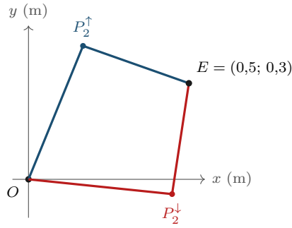
Figura 13.3: Le due soluzioni di cinematica inversa dell'Esempio 13.1 per lo stesso bersaglio E : gomito su (blu, P_2^\uparrow ) e gomito giù (rosso, P_2^\downarrow ), immagini speculari rispetto alla retta OE , come dimostrato nell'Osservazione 13.5.
