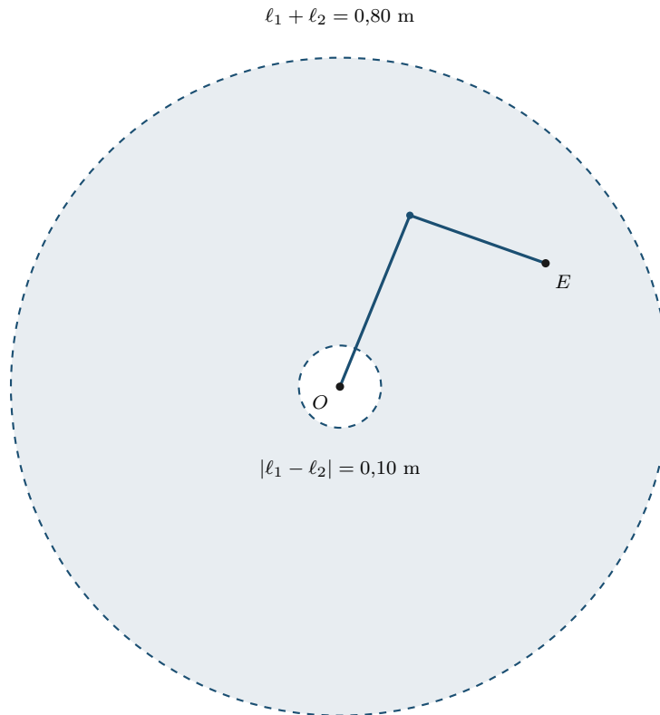
Figura 13.4: Lo spazio di lavoro W dell'Osservazione 13.4: la corona circolare fra |\ell_1 - \ell_2| = 0,10 m e \ell_1 + \ell_2 = 0,80 m. Il braccio in configurazione gomito su raggiunge il bersaglio E dell'Esempio 13.1, ben interno alla corona.
