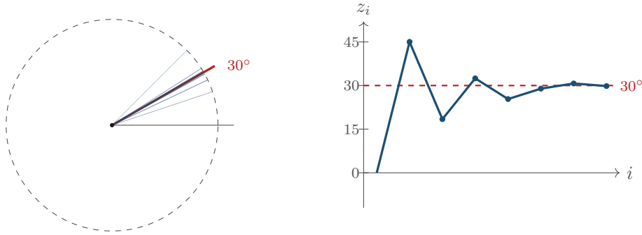
Figura 11.2: CORDIC: la trigonometria per sole addizioni e scorrimenti. L'angolo obiettivo ( 30^\circ ) si raggiunge sommando o sottraendo, in ordine fisso, gli angoli elementari \arctan 2^{-i} : 45^\circ , 26,565^\circ , 14,036^\circ , 7,125^\circ , 3,576^\circ , 1,790^\circ , 0,895^\circ . A sinistra le successive direzioni del vettore, a destra la successione z_i degli angoli accumulati, che converge a 30^\circ oscillando attorno al valore. La scelta del segno è l'unica decisione: ogni rotazione elementare si realizza con x' = x \mp y 2^{-i} , y' = y \pm x 2^{-i} , cioè con due scorrimenti e due addizioni, e il fattore di scala accumulato è una costante nota. Dopo n passi l'errore è al più \arctan 2^{-n} : si guadagna circa un bit per iterazione.
