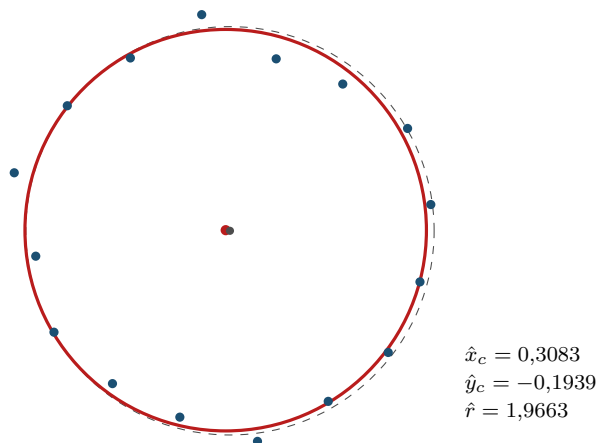
Figura 11.3: Stima di un cerchio da punti rumorosi con il metodo di Kåsa. I sedici punti blu sono stati generati sul cerchio grigio (centro (0,35; -0,20) , raggio 2) perturbando il raggio con rumore gaussiano di deviazione standard 0,10. Il metodo minimizza \sum_i (x_i^2 + y_i^2 + Dx_i + Ey_i + F)^2 , che è lineare nelle incognite D, E, F e si risolve con un sistema 3 \times 3 ; da esse (x_c, y_c) = (-D/2, -E/2) e r = \sqrt{D^2/4 + E^2/4 - F} . Il cerchio rosso è la stima ottenuta. Il pregio è di non richiedere iterazioni; il difetto è che la quantità minimizzata non è la distanza geometrica ma la potenza del punto, sicché la stima è distorta quando i punti coprono solo un arco breve.
