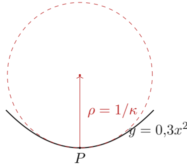
Figura 1.2: Il cerchio osculatore in P = (0,0) alla parabola y = 0,3x^2 . Qui x' = 1 , y' = 0,6x , x'' = 0 , y'' = 0,6 , dunque \kappa(0) = 0,6 e \rho = 1/0,6 = 1,6\bar{6} .
