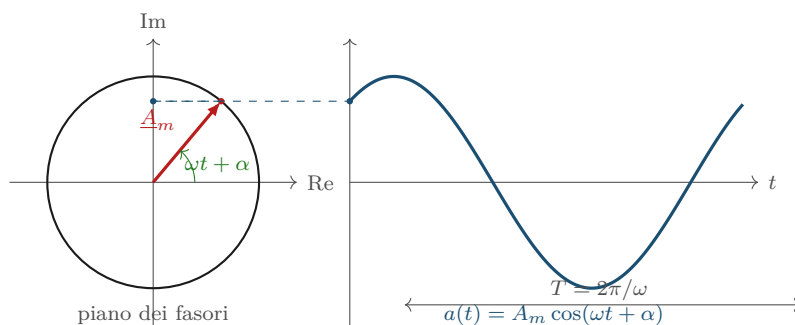
Figura 5.1: Il fasore e la sua ombra. A sinistra il punto \underline{A}_m e^{i\omega t} che percorre il cerchio di raggio A_m con velocità angolare \omega ; a destra la sinusoide generata dalla sua proiezione, letta in funzione del tempo. Le due figure sono lo stesso oggetto: il cerchio ne è la fotografia istantanea, la sinusoide la registrazione (Teorema 5.1).
