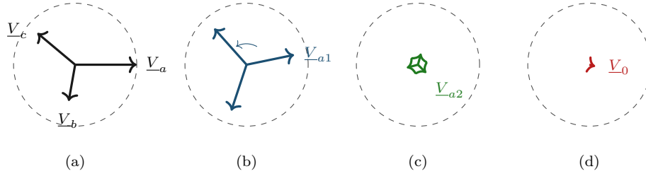
Figura 5.7: La scomposizione di Fortescue di una terna squilibrata. In (a) la terna assegnata \underline{V}_a = 1\angle 0^\circ , \underline{V}_b = 0,6\angle -100^\circ , \underline{V}_c = 0,8\angle 140^\circ . In (b), (c), (d) le tre terne componenti: la sequenza diretta ( 0,788\angle 11,7^\circ , che ruota nel verso a-b-c ), la sequenza inversa ( 0,189\angle -45^\circ , che ruota nel verso opposto) e la sequenza omopolare ( 0,098\angle -15,2^\circ , tre fasori identici). Le formule \underline{V}_{0,1,2} = \frac{1}{3}(\underline{V}_a + a^k \underline{V}_b + a^{2k} \underline{V}_c) sono esattamente la trasformata discreta di Fourier a tre punti, e la ricostruzione \underline{V}_a = \underline{V}_0 + \underline{V}_1 + \underline{V}_2 ne è l'antitrasformata.
