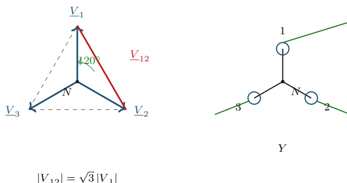
Figura 5.6: Il sistema trifase simmetrico. A sinistra la terna di tensioni stellate, tre fasori di uguale modulo sfasati di 120^\circ : la loro somma è nulla, perché 1 + a + a^2 = 0 con a = e^{j2\pi/3} . È la stessa identità che dice che le radici cubiche dell'unità hanno somma zero, e da essa discende che nel sistema equilibrato il conduttore di neutro non porta corrente. La tensione concatenata \underline{V}_{12} = \underline{V}_1 - \underline{V}_2 è il lato del triangolo inscritto: ha modulo \sqrt{3} volte quello di fase e anticipa di 30^\circ , donde la coppia 230/400 V della rete europea, con 400 \simeq 230\sqrt{3} . A destra la corrispondente connessione a stella.
