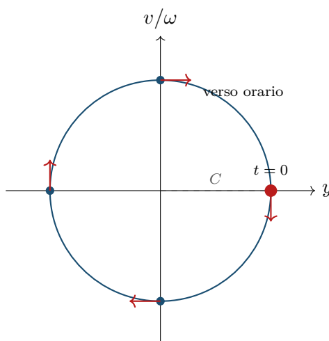
Figura 9.1: Ritratto di fase dell'oscillatore armonico (Teorema 9.4): il punto (y(t), v(t)/\omega) percorre in verso orario, a velocità angolare \omega costante, la circonferenza di raggio C . Le quattro frecce rosse indicano la direzione del moto nei quattro punti cardinali della traiettoria, coerenti con \dot{y}(0) > 0 \Rightarrow discesa da (C, 0) verso il quarto quadrante, come nella dimostrazione.
