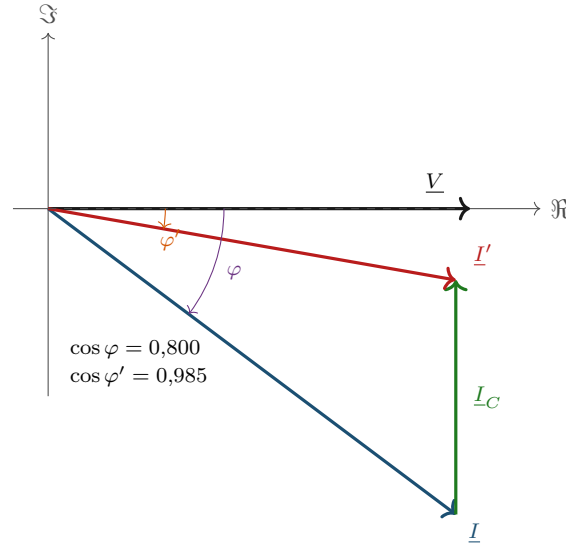
Figura 5.3: Il rifasamento visto sul diagramma dei fasori. Il carico induttivo assorbe la corrente \underline{I} in ritardo di \varphi = 36,87^\circ sulla tensione \underline{V} ( \cos \varphi = 0,8 ). Il condensatore in parallelo assorbe una corrente \underline{I}_C puramente immaginaria e in anticipo di 90^\circ , che si somma verticalmente e accorcia la componente reattiva senza toccare quella attiva: la corrente di linea diventa \underline{I}' , di modulo minore e sfasata di soli \varphi' = 9,94^\circ ( \cos \varphi' = 0,985 ). La potenza attiva è rimasta la stessa ( P = \Re \underline{V} \underline{I}^* non cambia), ma la linea trasporta il 19% di corrente in meno e le perdite per effetto Joule, che vanno come I^2 , calano del 34%.
