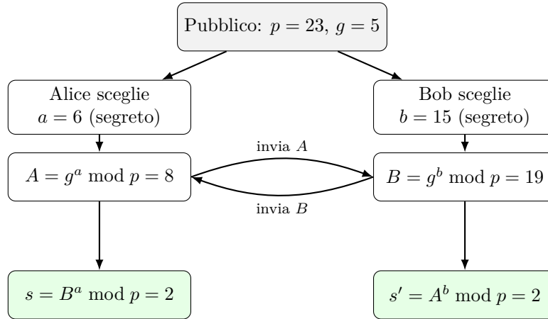
Figura 12.2: Il protocollo di scambio di chiavi di Diffie–Hellman, con i valori dell’Esempio 12.1 ( p = 23 , g = 5 ): Alice e Bob calcolano indipendentemente lo stesso segreto s = s' = 2 (Teorema 12.1), pur scambiandosi solo A, B in chiaro.
