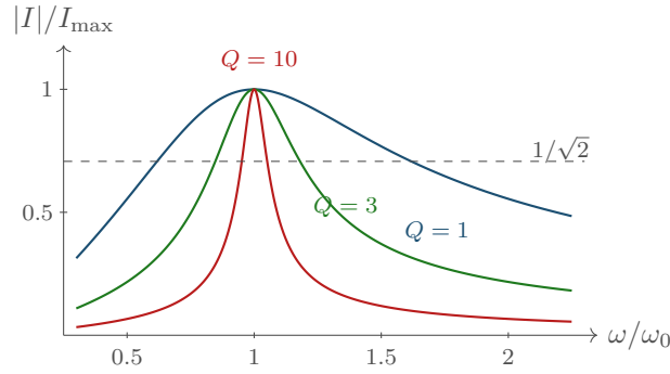
Figura 5.4: Le curve di risonanza di un circuito RLC serie, per tre valori del fattore di merito Q = \omega_0 L/R . In forma normalizzata |I|/I_{\max} = 1/\sqrt{1 + Q^2(x - 1/x)^2} con x = \omega/\omega_0 : tutte le curve valgono 1 in x = 1 , dove la reattanza si annulla e il circuito è puramente resistivo. La banda passante a -3 dB, cioè l'intervallo in cui |I|/I_{\max} \geq 1/\sqrt{2} , ha ampiezza \Delta\omega = \omega_0/Q : il fattore di merito è esattamente il rapporto fra frequenza di risonanza e larghezza di banda. Si noti l'asimmetria delle curve rispetto a x = 1 : la scala naturale del fenomeno è logaritmica, e la curva è simmetrica in \ln x .
