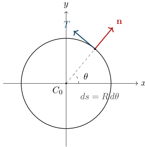
Figura 2.1: Gli elementi differenziali sulla circonferenza percorsa in senso antiorario: il versore tangente T , il versore normale esterno \mathbf{n} (che coincide con il versore radiale) e l'elemento di lunghezza ds = R d\theta .
