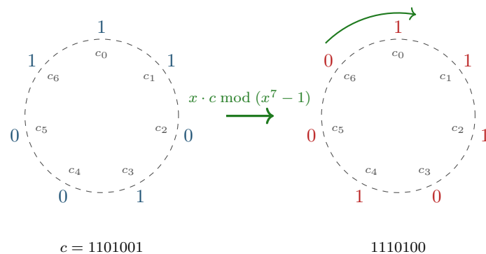
Figura 7.5: Perché i codici ciclici si chiamano così. Disponendo i sette bit di una parola di codice sui vertici di un 7-gono, lo scorrimento ciclico di una posizione è semplicemente una rotazione della figura. Algebricamente, identificando la parola c_0 c_1 \dots c_6 con il polinomio c(x) = c_0 + c_1 x + \dots + c_6 x^6 dell'anello \mathbb{F}_2[x]/(x^7 - 1) , lo scorrimento è la moltiplicazione per x : il gruppo delle rotazioni del cerchio discreto agisce sul codice. Un codice ciclico è per definizione un sottospazio chiuso rispetto a questa azione, e si dimostra che tale sottospazio è sempre l'ideale generato da un divisore g(x) di x^n - 1 : il polinomio generatore.
