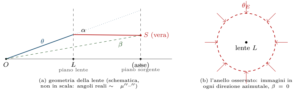
Figura 11.2: Geometria della lente gravitazionale (Teorema 11.3) e anello di Einstein nel caso allineato (Teorema 11.4). Pannello (a): schema qualitativo con angoli fortemente ingranditi per chiarezza grafica (non in scala). Pannello (b): vista frontale dall'osservatore nel caso \beta = 0 , con immagini che arrivano da ogni direzione azimutale a distanza angolare \theta_E dalla lente, formando il cerchio completo del Teorema 11.4.
