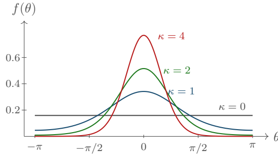
Figura 6.3: La densità di von Mises f(\theta) = e^{\kappa \cos(\theta-\mu)} / (2\pi I_0(\kappa)) con \mu = 0 , per \kappa = 0, 1, 2, 4 . Per \kappa = 0 si riduce alla densità uniforme 1/(2\pi) ; al crescere di \kappa si concentra attorno alla direzione media \mu . La costante di normalizzazione è la funzione di Bessel modificata I_0(\kappa) = \frac{1}{2\pi} \int_0^{2\pi} e^{\kappa \cos t} dt ( I_0(1) = 1,2661 , I_0(2) = 2,2796 , I_0(4) = 11,3019 ): è il caso p = 0 della famiglia I_p , i cui valori sono esattamente i coefficienti di Fourier di e^{\kappa \cos t} . Per \kappa grande la von Mises approssima una gaussiana di varianza 1/\kappa .
