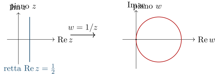
Figura 3.2: La retta \operatorname{Re} z = \frac{1}{2} (che non passa per l'origine) è mandata dall'inversione w = 1/z nel cerchio di centro 1 e raggio 1, che passa per l'origine: è la regola A = 0 \Rightarrow C' = A = 0 del Passo 3, letta al contrario.
