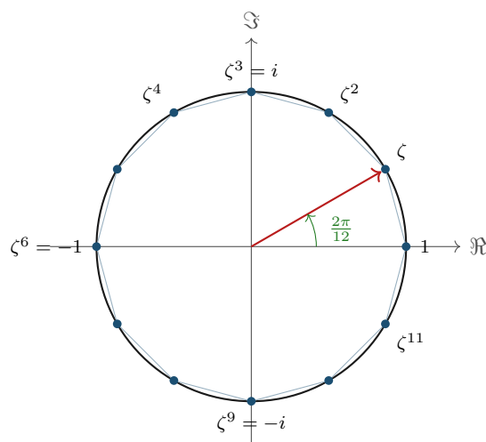
Figura 7.1: Le dodici radici dodicesime dell'unità, cioè le soluzioni di z^{12} = 1 : sono i vertici del poligono regolare di 12 lati inscritto nel cerchio unitario, di coordinate \zeta^k = e^{2\pi i k/12} . Rispetto alla moltiplicazione formano un gruppo ciclico \mu_{12} generato da \zeta = e^{2\pi i/12} , e l'isomorfismo k \mapsto \zeta^k identifica \mathbb{Z}/12\mathbb{Z} con \mu_{12} : sommare esponenti modulo 12 e moltiplicare radici sono la stessa operazione. Dividere il cerchio in parti uguali e fare aritmetica modulare sono dunque due descrizioni dello stesso oggetto.
