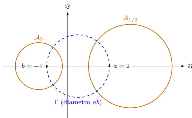
Figura 8.1: Due cerchi di Apollonio del fascio non secante di punti limite a = 2, b = -1 (arancio, \mathcal{A}_3 e \mathcal{A}_{1/2} , dall'Esercizio N1) e un cerchio \Gamma del fascio secante ortogonale per a, b (blu tratteggiato, di diametro ab ): la relazione |c_1 - c_2|^2 = r_1^2 + r_2^2 verificata nell'Esercizio N2 illustra il Teorema 8.3.
