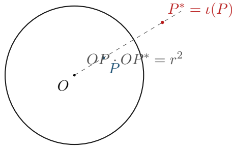
Figura 3.1: Inversione rispetto a C(O, r) : P e P^* giacciono sulla stessa semiretta uscente da O , con OP \cdot OP^* = r^2 ; i punti della circonferenza restano fissi (Proposizione 3.1).
