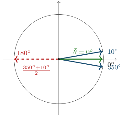
Figura 6.1: Perché sul cerchio la media aritmetica non funziona. Due direzioni misurate a 350^\circ e 10^\circ sono vicinissime fra loro (distanza 20^\circ ), ma la loro media aritmetica (350 + 10)/2 = 180^\circ cade dalla parte opposta del cerchio. La media circolare risolve il problema trattando le osservazioni come vettori unitari e mediando i vettori: la somma (\cos 350^\circ + \cos 10^\circ, \sin 350^\circ + \sin 10^\circ) = (1,970, 0) punta esattamente a \bar{\theta} = 0^\circ , che è la risposta giusta.
