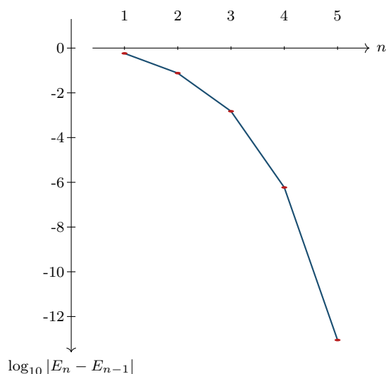
Figura 10.2: Convergenza quadratica dell'iterazione di Newton per l'equazione di Keplero (Esempio 10.3, M = 1 , e = 0,5 ): errore |E_n - E_{n-1}| in scala semi-logaritmica ( \log_{10} in ordinata). La concavità marcata verso il basso, invece di un allineamento su una retta (che indicherebbe convergenza solo lineare), è la firma grafica del raddoppio delle cifre esatte a ogni passo previsto dal Corollario 10.1: valori di \log_{10} |E_n - E_{n-1}| pari a -0,24 , -1,12 , -2,82 , -6,23 , -13,05 per n = 1, \dots, 5 , calcolati da vol2_cap10_keplero.py .
