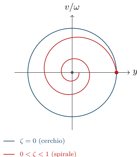
Figura 9.2: Confronto qualitativo dei ritratti di fase: il cerchio blu è la traiettoria non smorzata di raggio costante ( \zeta = 0 , Teorema 9.4); la spirale rossa r(\theta) = e^{-0,15\theta} illustra il caso sottosmorzato ( 0 < \zeta < 1 , Osservazione 9.4), che collassa verso l'origine pur partendo dallo stesso punto (1, 0) : il decadimento è generato dalla stessa famiglia di spirali logaritmiche del Capitolo 1, qui non richiesta per il calcolo (formula esplicita), ma solo a scopo illustrativo del comportamento qualitativo descritto nell'osservazione citata.
