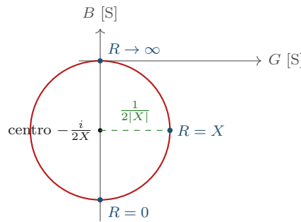
Figura 5.5: Il diagramma circolare. Al variare della sola resistenza R , con reattanza X > 0 fissata, l'ammettenza percorre la semicirconferenza destra di centro -i/(2X) e raggio 1/(2|X|) (Teorema 5.17). Il punto di massima conduttanza, e dunque di massima potenza attiva a tensione fissata, si ha per R = X .
