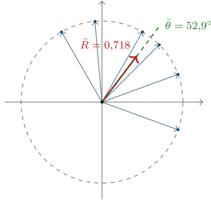
Figura 6.2: La risultante di sei direzioni. Ogni osservazione \theta_j diventa il versore (\cos \theta_j, \sin \theta_j) ; la loro media vettoriale ha modulo \bar{R} e argomento \bar{\theta} . Qui \bar{R} = 0,718 : il valore sta fra 0 (direzioni perfettamente sparse, risultante nulla) e 1 (direzioni tutte coincidenti). La lunghezza \bar{R} misura dunque la concentrazione, e la varianza circolare si definisce come V = 1 - \bar{R} . Si noti che \bar{R} è esattamente il modulo del primo momento trigonometrico, cioè del primo coefficiente di Fourier empirico.
