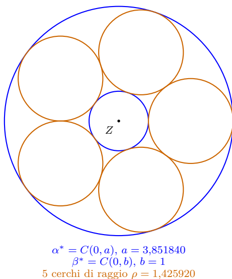
Figura 8.2: La catena di Steiner a chiusura esatta dell'Esempio 8.3 nel caso concentrico: cinque cerchi congruenti (arancio), ciascuno tangente internamente ad \alpha^* , esternamente a \beta^* e ai due vicini (Porisma di Steiner, Volume I, Capitolo 5). Applicando l'inversa dell'inversione di riduzione (Osservazione 8.4) questa figura torna alla catena per la coppia originaria \alpha, \beta , non concentrica.
