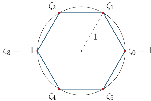
Figura 3.3: Le radici seste dell'unità: vertici di un esagono regolare inscritto in \mathbb{T} , con un vertice in 1. Il lato misura 2\sin(\pi/6) = 1 , uguale al raggio — la proprietà caratteristica dell'esagono regolare già osservata nel Volume I.
