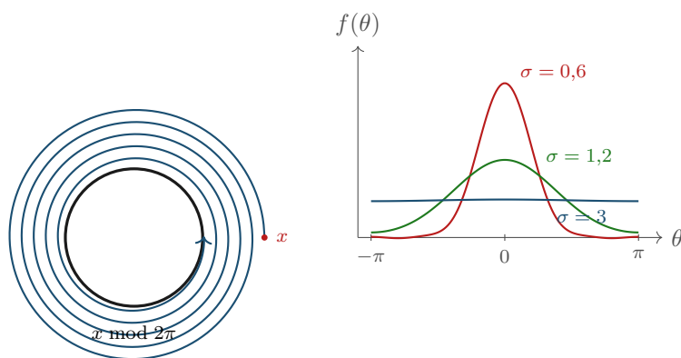
Figura 6.4: L'avvolgimento è un aliasing. A sinistra: la retta reale si avvolge sul cerchio tramite x \mapsto x \bmod 2\pi ; tutti i punti x + 2\pi k finiscono nello stesso posto. A destra: la densità normale avvolta, cioè l'immagine di una N(0, \sigma^2) tramite quella mappa. I suoi coefficienti di Fourier sono \rho_k = e^{-k^2 \sigma^2 / 2} : l'avvolgimento somma le repliche traslate di 2\pi esattamente come il campionamento somma le repliche spettrali. Al crescere di \sigma i coefficienti con k \geq 1 si spengono e la densità tende all'uniforme: quando la deviazione supera l'ampiezza del cerchio, l'informazione sulla direzione si perde del tutto.
