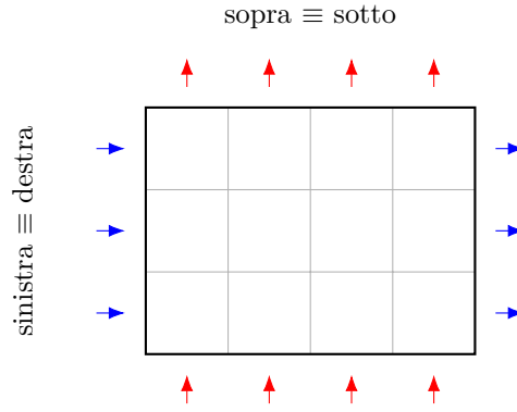
Figura 13.1: Il toro discreto \mathbb{Z}/4\mathbb{Z} \times \mathbb{Z}/3\mathbb{Z} (esempio con n = 4, m = 3 ): la griglia n \times m con i lati opposti identificati nello stesso verso (freccie blu: colonna n - 1 e colonna 0 sono adiacenti; frecce rosse: riga m - 1 e riga 0 sono adiacenti) — esattamente come il cerchio \mathbb{Z}/n\mathbb{Z} è un segmento con i due estremi identificati.
