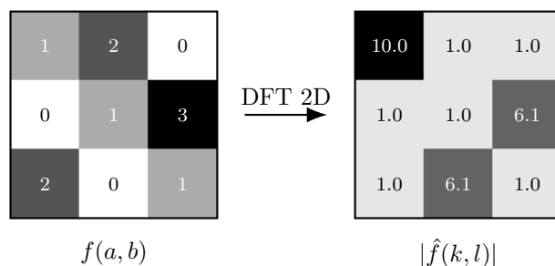
Figura 13.2: L'esempio 3 \times 3 dell'Esempio 13.1, come griglia: a sinistra il dominio spaziale f(a,b) (ombreggiatura proporzionale al valore, 0–3), a destra il modulo della DFT |\hat{f}(k,l)| (ombreggiatura proporzionale al valore, 0–10; celle calcolate con vol2_cap12_dft2d.py ). Il valore \hat{f}(0,0) = 10 (in alto a sinistra nella griglia di frequenza) è sempre la somma di tutti i valori spaziali: 1+2+0+0+1+3+2+0+1 = 10 .
