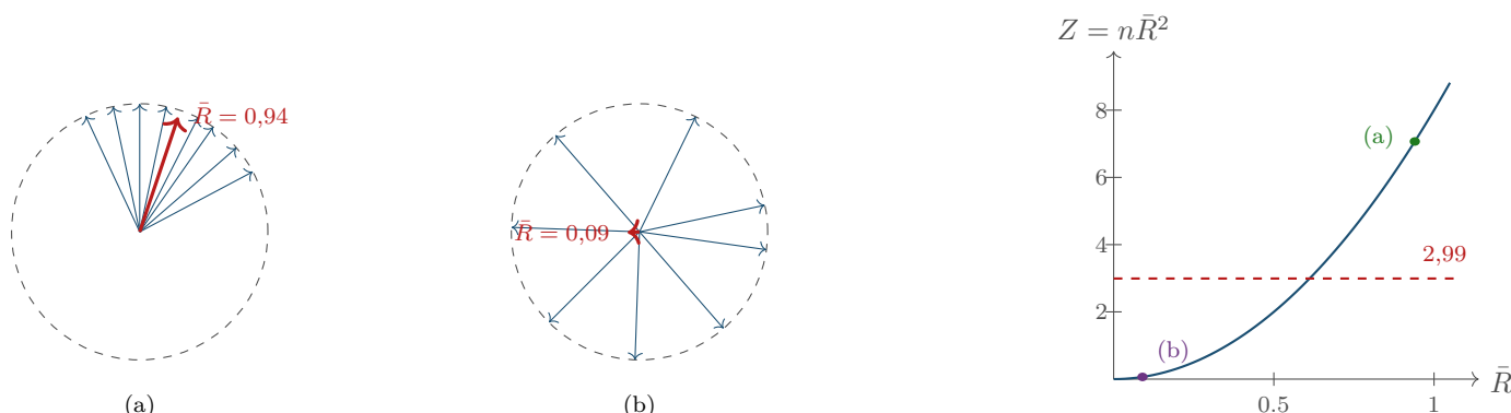
Figura 6.5: Il test di Rayleigh in una figura. A sinistra un campione di n = 8 direzioni fortemente concentrato: la risultante è lunga, \bar{R} = 0,94 . Al centro un campione quasi uniforme: le direzioni si elidono e \bar{R} = 0,09 . A destra la statistica di Rayleigh Z = n\bar{R}^2 in funzione di \bar{R} : sotto l'ipotesi nulla di uniformità Z tende in distribuzione a una esponenziale di media 1, dunque si rifiuta l'uniformità quando Z > -\ln \alpha , cioè Z > 2,99 al livello \alpha = 0,05 . Il campione concentrato dà Z = 8 \cdot 0,94^2 = 7,07 (si rifiuta), quello sparso Z = 8 \cdot 0,09^2 = 0,065 (non si rifiuta).
