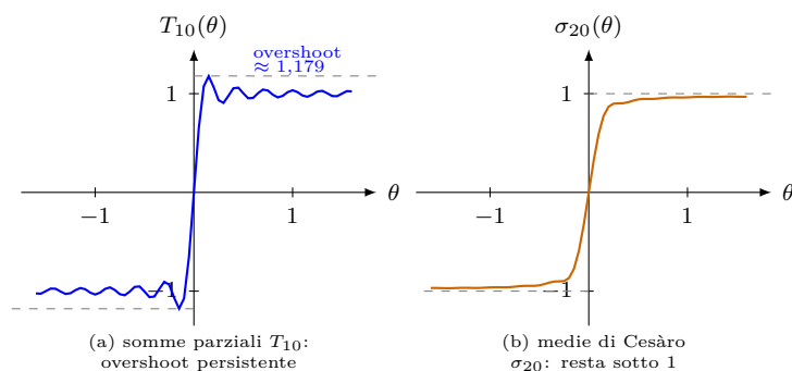
Figura 4.1: Confronto fra le somme parziali T_{10} (a), che superano stabilmente l'ampiezza 1 della funzione vicino al salto (Teorema 4.17), e le medie di Cesàro \sigma_{20} (b), che non la superano mai (Proposizione 4.1) — stessi dati dello script vol2_cap04_gibbs.py .
