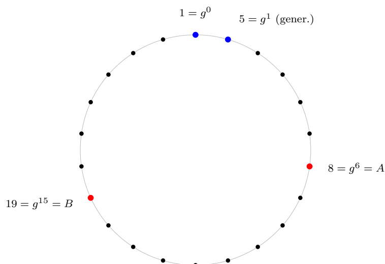
Figura 12.1: Gli elementi di (\mathbb{Z}/23\mathbb{Z})^\times disposti secondo l'esponente k nel generatore g = 5 : la stessa struttura ciclica — lo stesso “cerchio discreto” — del Capitolo 7. Evidenziati A, B dell'Esempio 12.1, alle posizioni k = 6, 15 verificate con lo script vol2_cap11_figure_gruppo.py .
