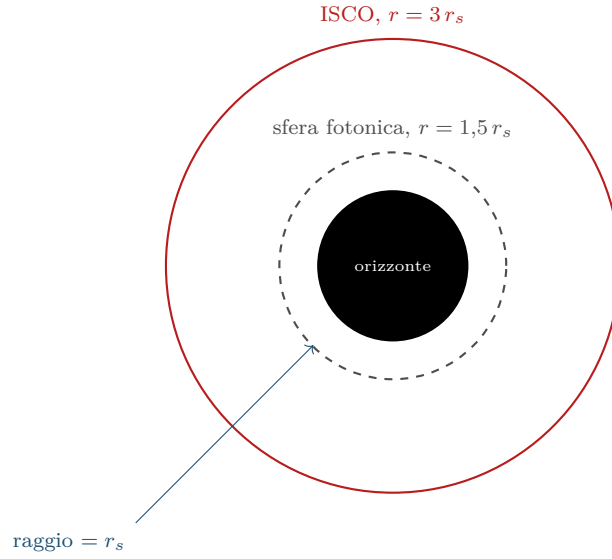
Figura 11.1: Le tre scale caratteristiche del buco nero di Schwarzschild, in scala reale fra loro (raggi in unità di r_s ): l'orizzonte a r = r_s (disco nero, Definizione importata), la sfera fotonica a r = 1,5 r_s (Teorema 11.1, cerchio grigio tratteggiato) e l'ISCO a r = 3 r_s (Teorema 11.2, cerchio rosso).
