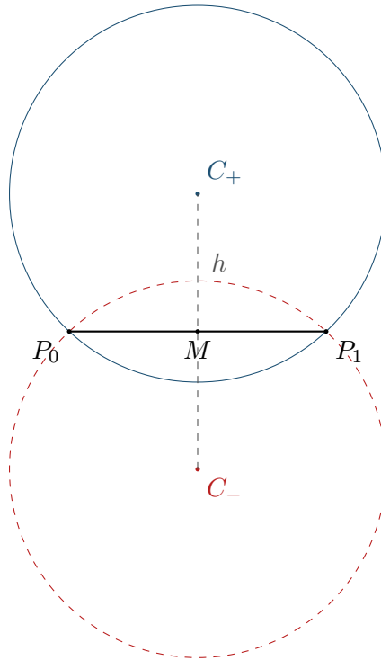
Figura 1.4: Metodo R: i due centri ammissibili giacciono sull'asse di P_0P_1 , simmetrici rispetto al punto medio M , a distanza h = \sqrt{R^2 - (d/2)^2} da esso.
