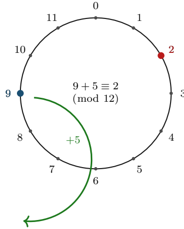
Figura 7.2: L'aritmetica modulare è aritmetica sul cerchio. Il quadrante di un orologio a 12 ore è una realizzazione concreta di \mathbb{Z}/12\mathbb{Z} : sommare 5 a partire da 9 significa percorrere cinque passi in avanti lungo il cerchio, e si arriva a 2, non a 14. Il riporto che si perde è esattamente un giro completo, cioè il modulo. Formalmente la mappa \mathbb{Z} \rightarrow \mathbb{Z}/12\mathbb{Z} è l'avvolgimento della retta degli interi sul cerchio di dodici posizioni, ed è un omomorfismo di gruppi: il nucleo è 12\mathbb{Z} .
