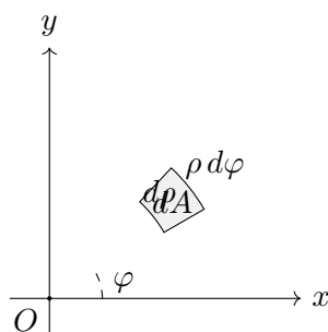
Figura 2.2: L'elemento d'area in coordinate polari: un rettangolo curvilineo di lati d\rho e \rho d\varphi , da cui dA = \rho d\rho d\varphi .
