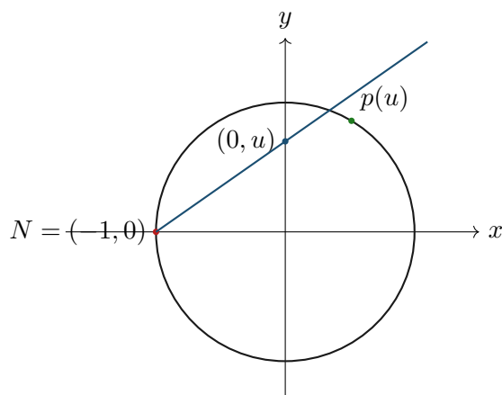
Figura 1.1: La proiezione stereografica dal polo N = (-1, 0) : al parametro u corrisponde il secondo punto d'intersezione della retta N(0, u) con la circonferenza. Al variare di u su tutto \mathbb{R} si ottengono tutti i punti di S^1 tranne N , che corrisponde intuitivamente a u \rightarrow \pm\infty .
