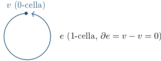
Figura 1.2: Struttura CW minimale di S^1 : una 0-cella v e una 1-cella e i cui due estremi coincidono in v , usata nell'Osservazione 1.5.
