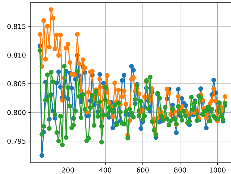
Dimension d=10
