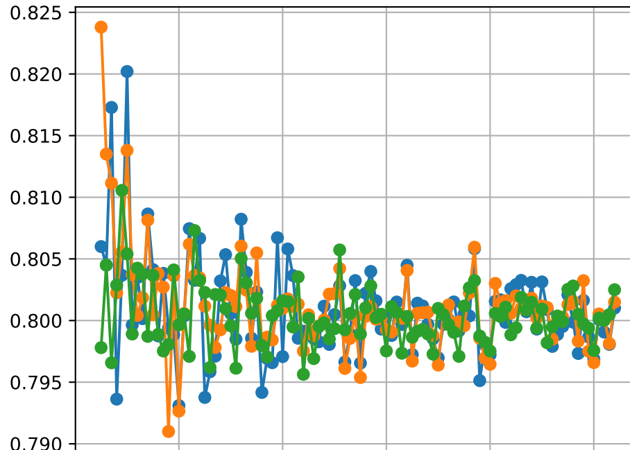
Dimension d=6
