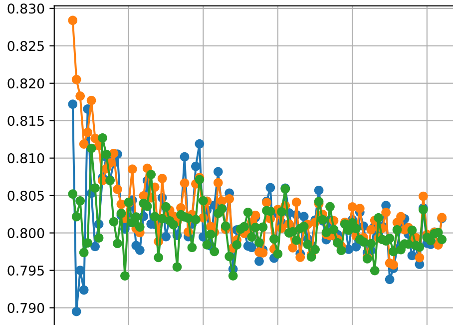
Dimension d=9
