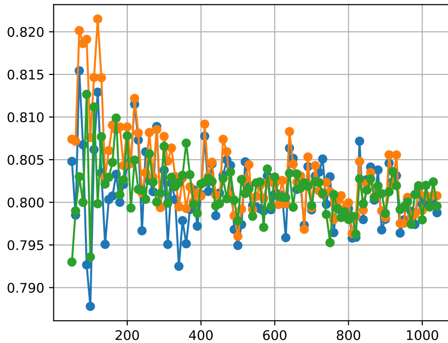
Dimension d=9
