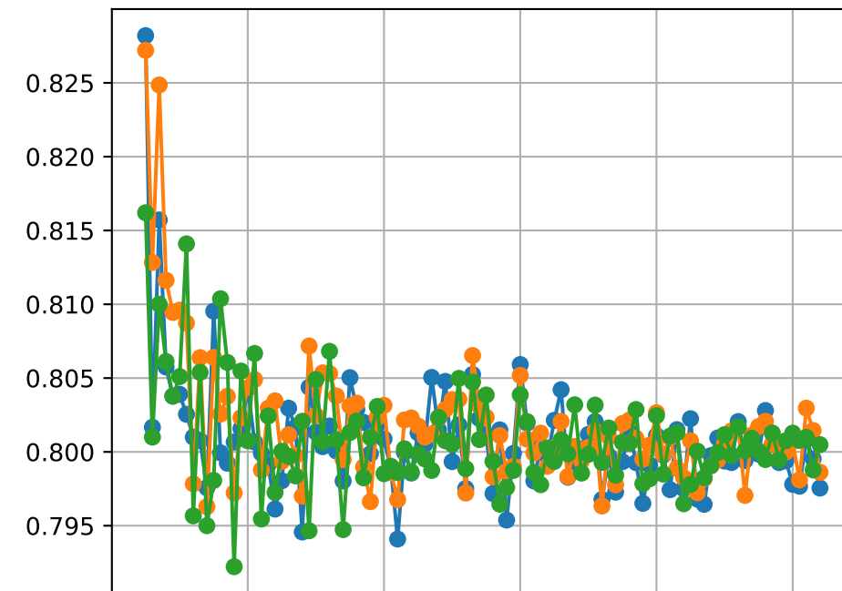
Dimension d=7
