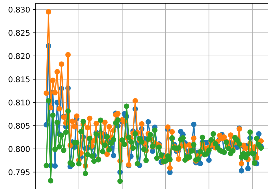
Dimension d=10
