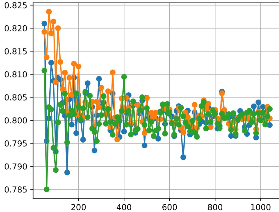
Dimension d=8
