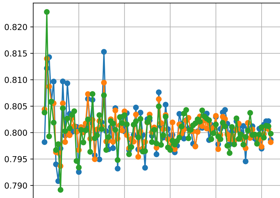
Dimension d=5
