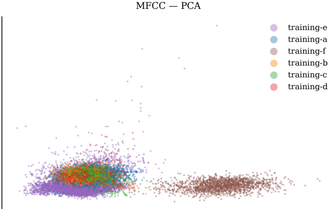
MFCC — PCA
