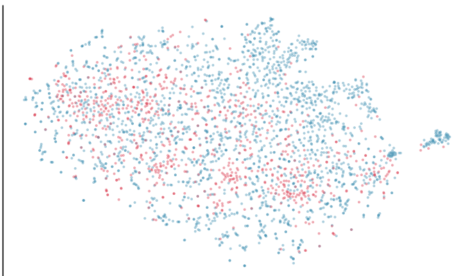
PWP — t-SNE
