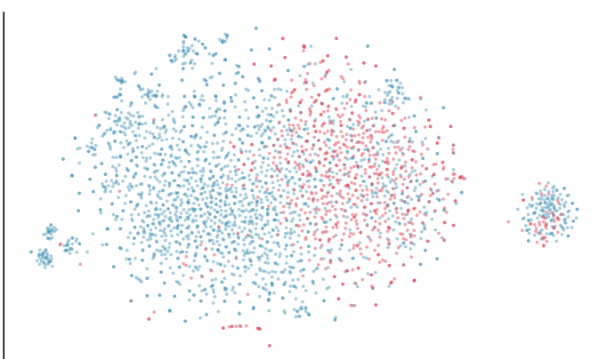
MFCC — t-SNE
