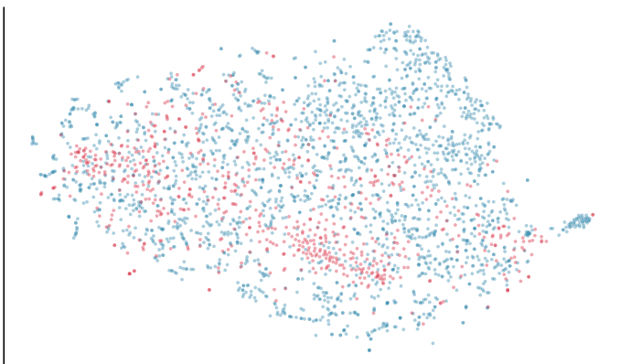
LOGMEL — t-SNE
