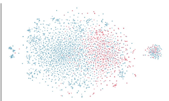
MFCC — t-SNE
