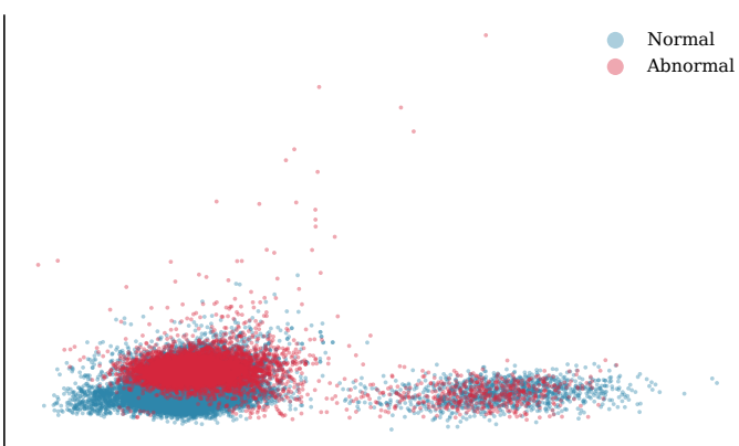
MFCC — PCA
