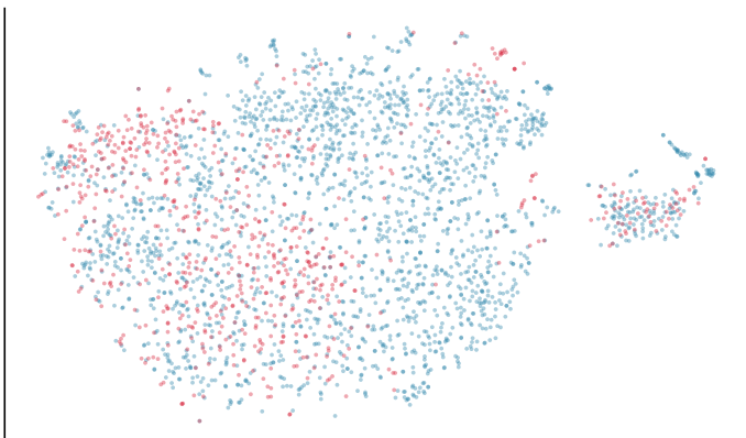
PWP — t-SNE
