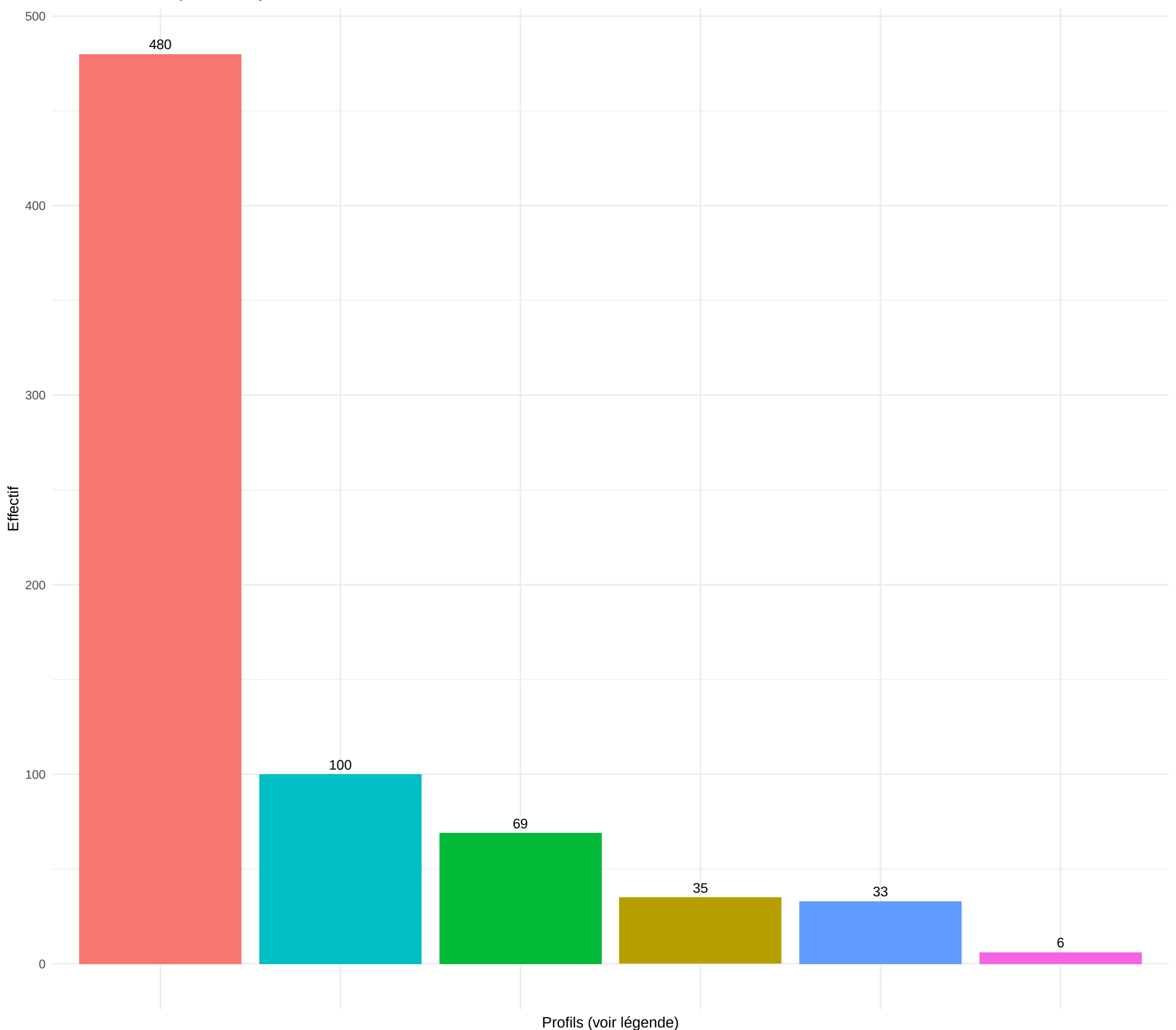
Distribution des profils subjectifs
