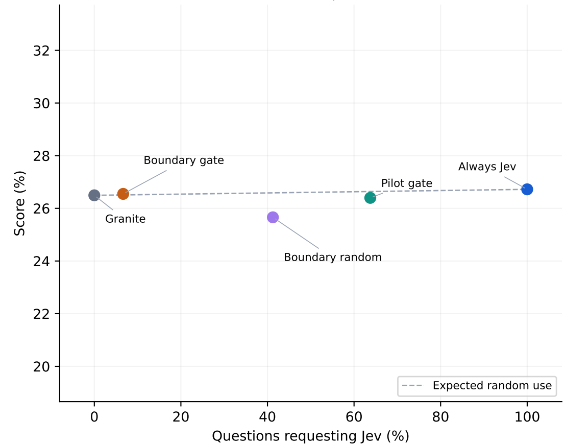
SQuAD2 adapted F1
