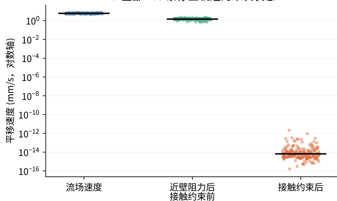
C 全部 185 条停止轨迹的末次状态
