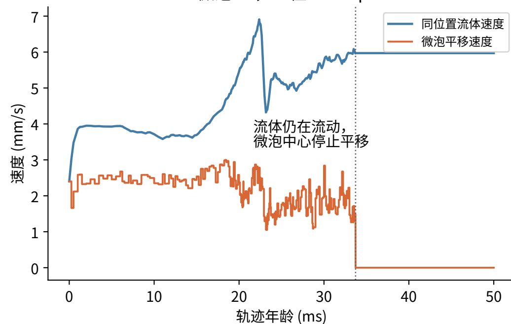
B 微泡 #2, 直径 2.110 \mu\text{m}
