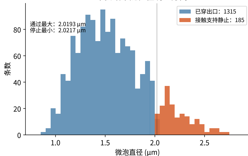
A 本批结果随粒径明显分离
