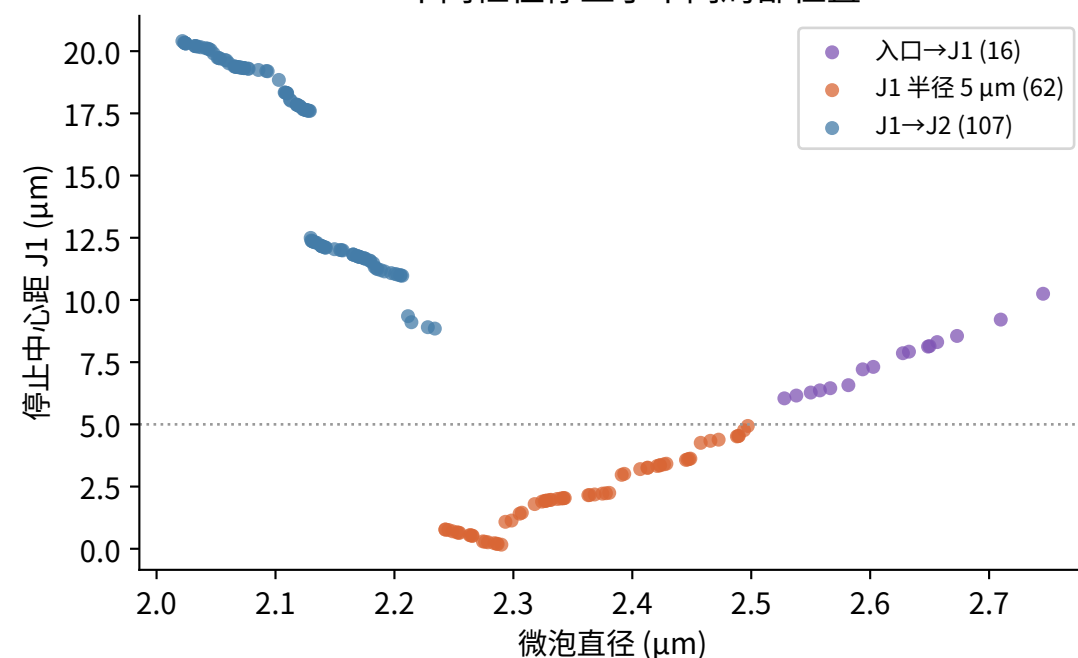
D 不同粒径停止于不同局部位置
