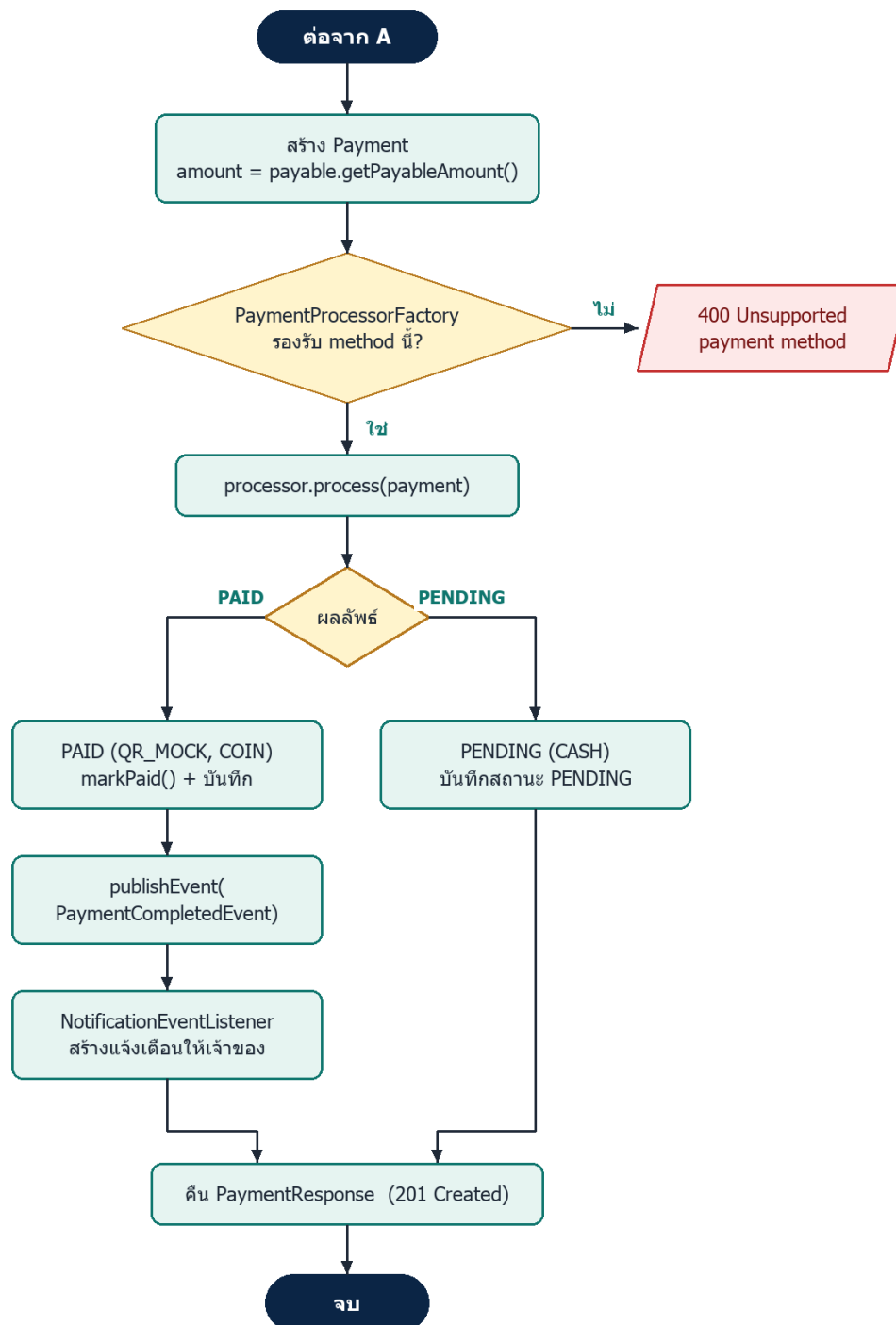
ภาพที่ 11 Activity Diagram ของ checkout ส่วนที่ 2: สร้าง Payment เลือก processor และยิง event พนักงานยืนยันรับเงินสดมีขั้นตอนสั้นกว่า โดยตรวจสอบสถานะปัจจุบันก่อน (จ่ายแล้วได้ 409, ล้มเหลวได้ 400, รอยืนยันจึงดำเนินการต่อ)
