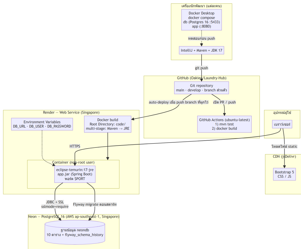
ภาพที่ 4 แผนภาพ Deployment ของระบบ
