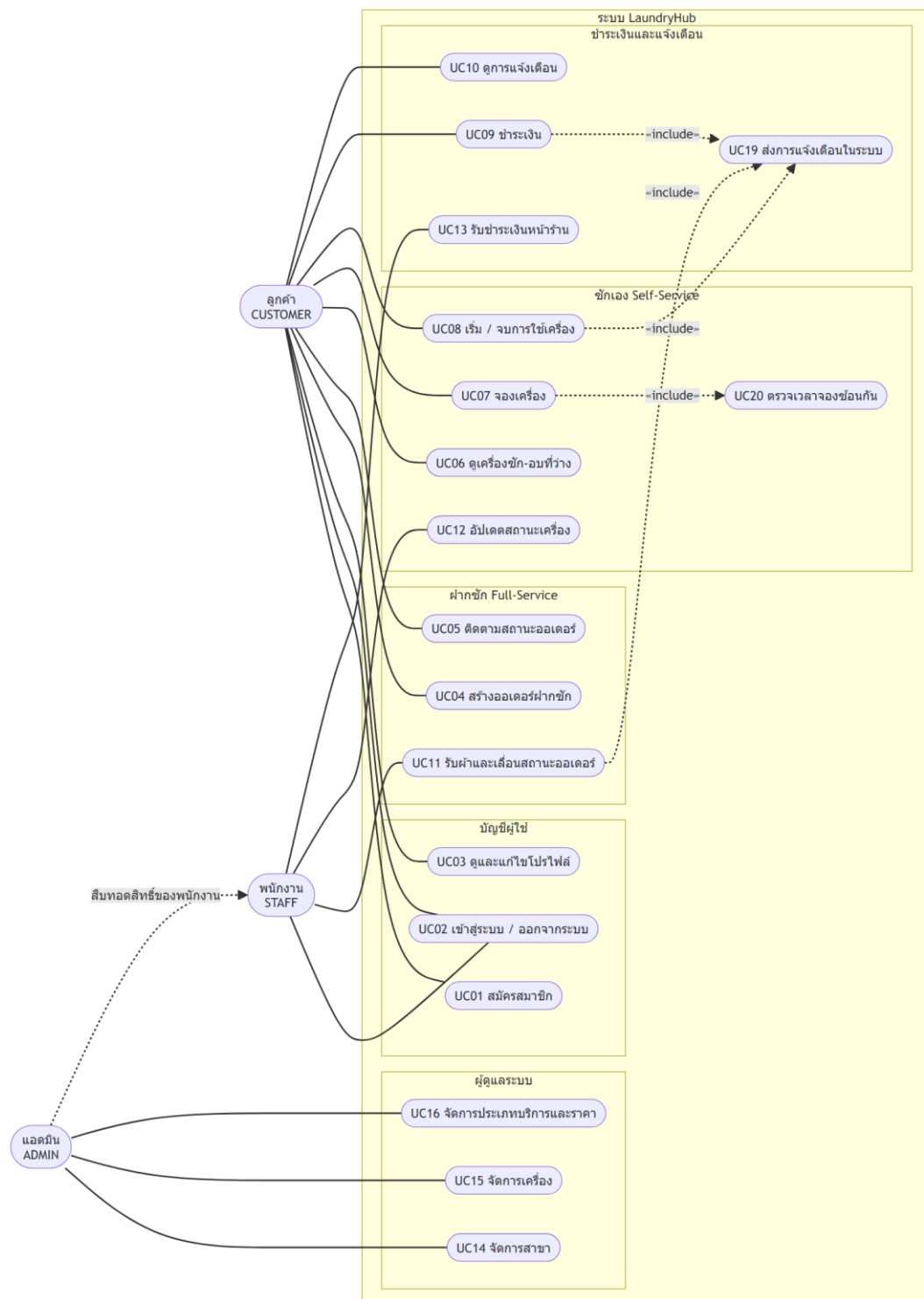
ภาพที่ 2 แผนภาพ Use Case ของระบบ LaundryHub
