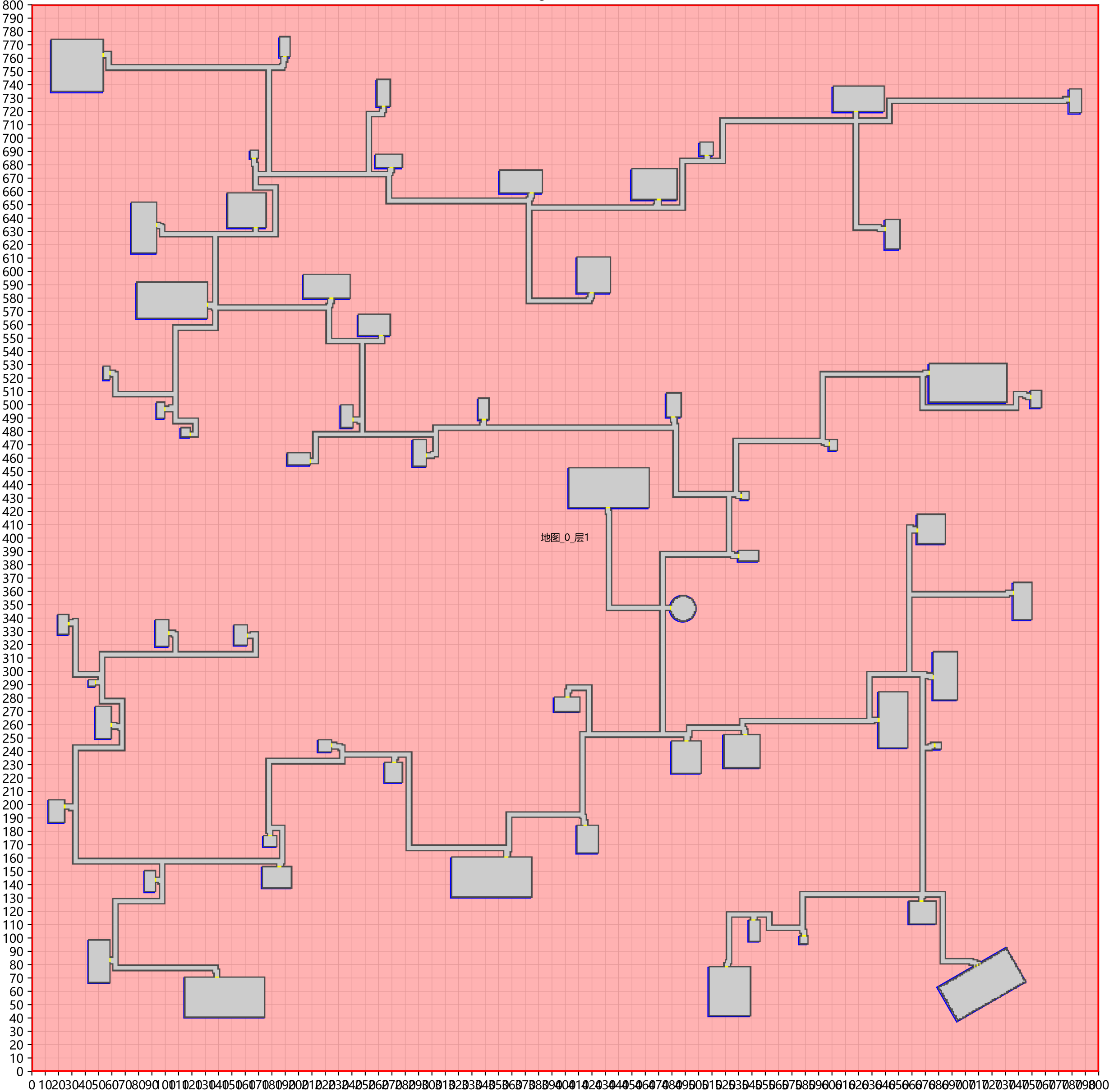
800x800-真菌优化-shrinkage=1-固定60建筑 - 层1 - 像素展示层
