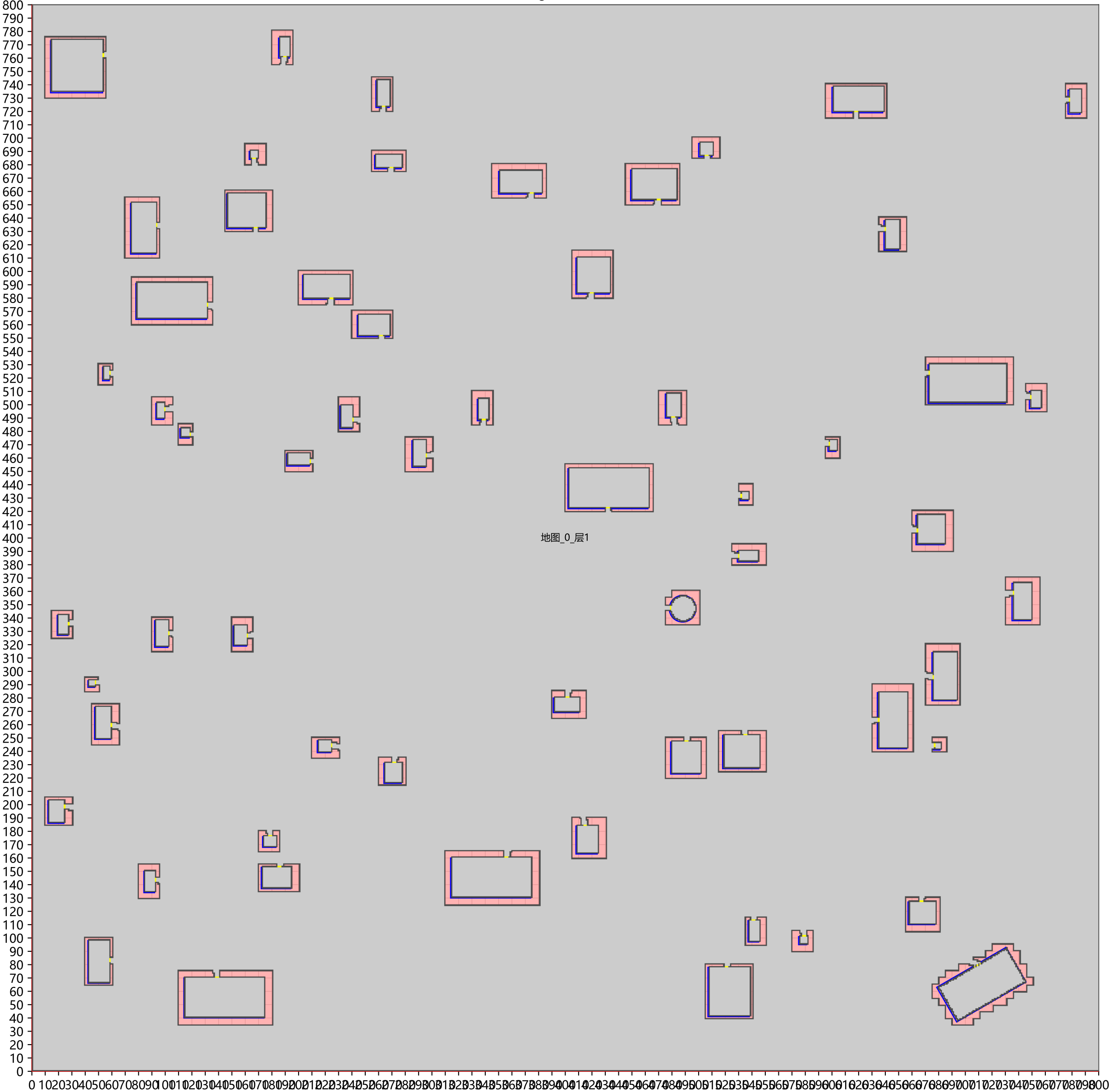
800x800-真菌优化-shrinkage=2-固定60建筑 - 层1 - 像素展示层
