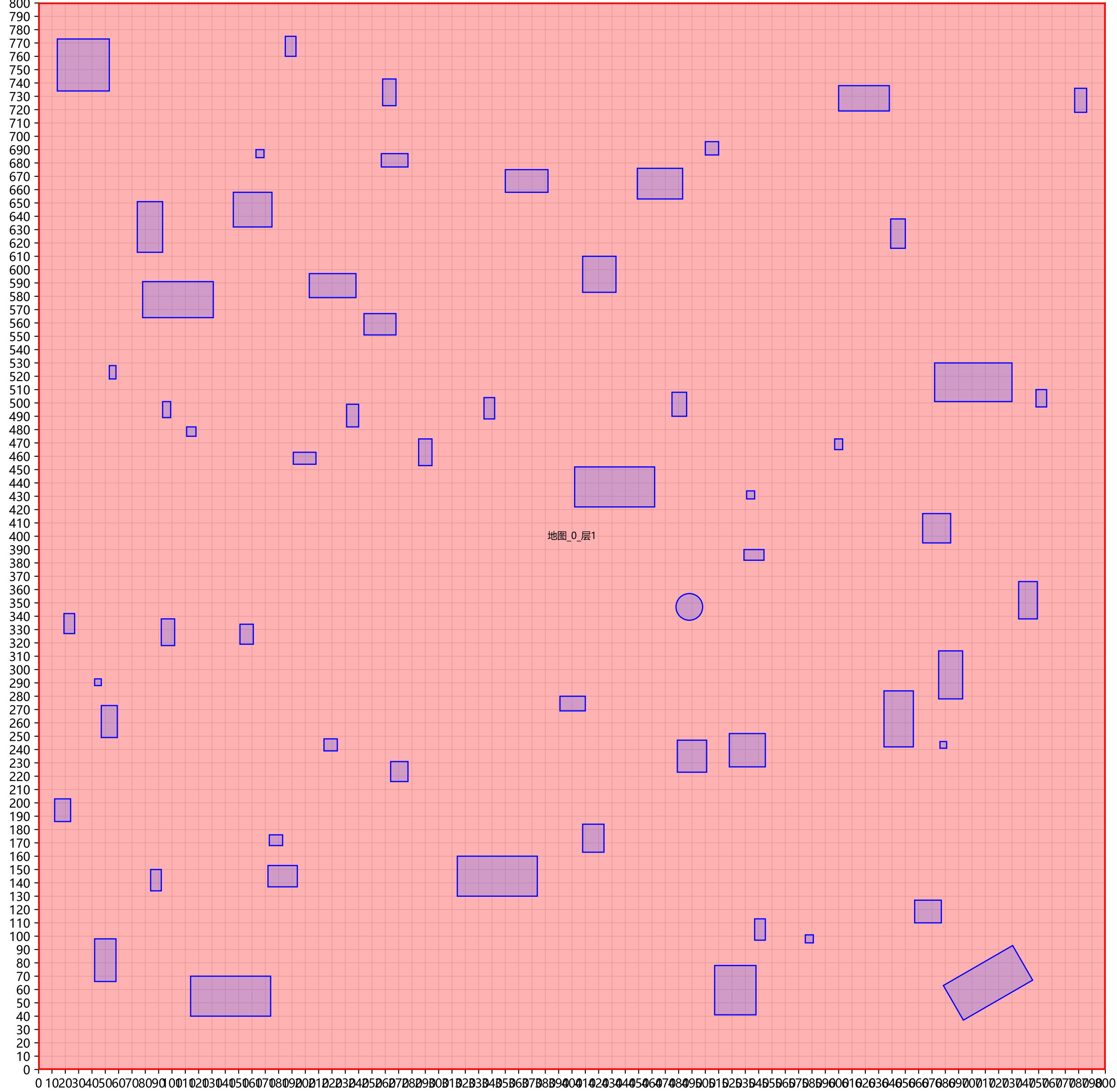
800x800真菌优化-Pareto收缩0.1-固定60建筑 - 层1 - 矢量展示层
