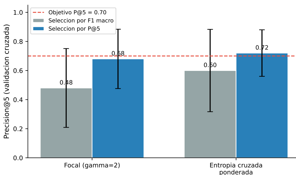
Figura 6. Precisión@5 de la ablación de pérdida y selección
