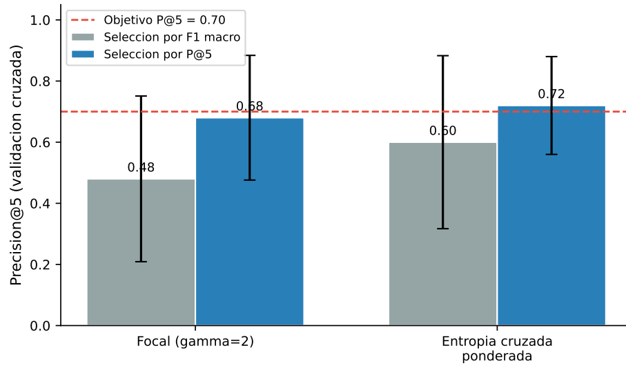
Figura 5.4: Ablación 2×2 de función de pérdida × criterio de selección de checkpoints (Precisión@5 de validación cruzada, \pm\sigma ). Solo la configuración desplegada —entropía cruzada ponderada con selección por Precisión@5— supera el objetivo de diseño.
