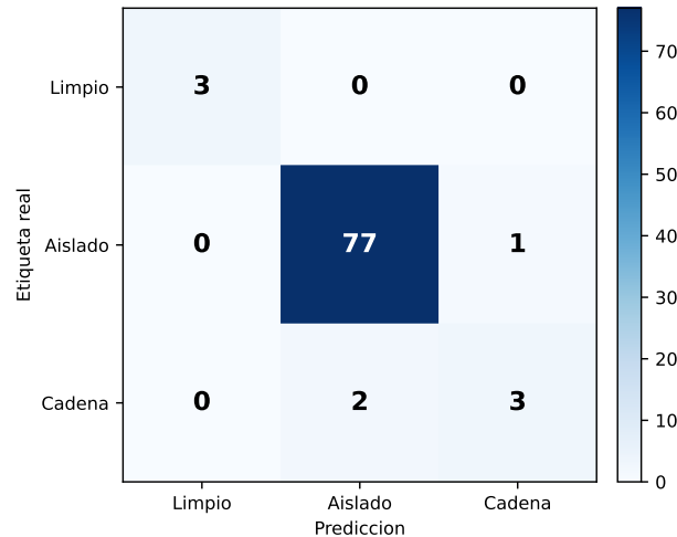
Figura 5.8: Matriz de confusión del ensemble de pliegues sobre el conjunto de test (clasificación argmax ). Los errores caen en la frontera cadena/aislado; ningún manifiesto crítico se degrada a limpio.
