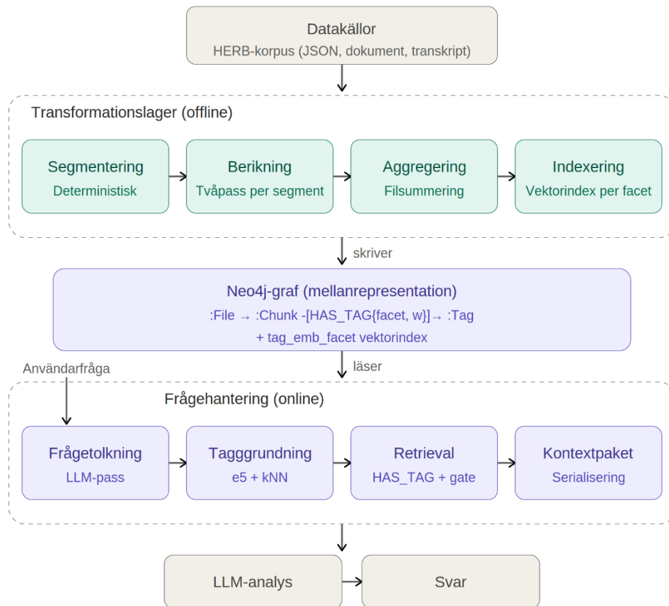
Figur 1. Systemöversikt över den grafbaserade RAG-artefakten.
