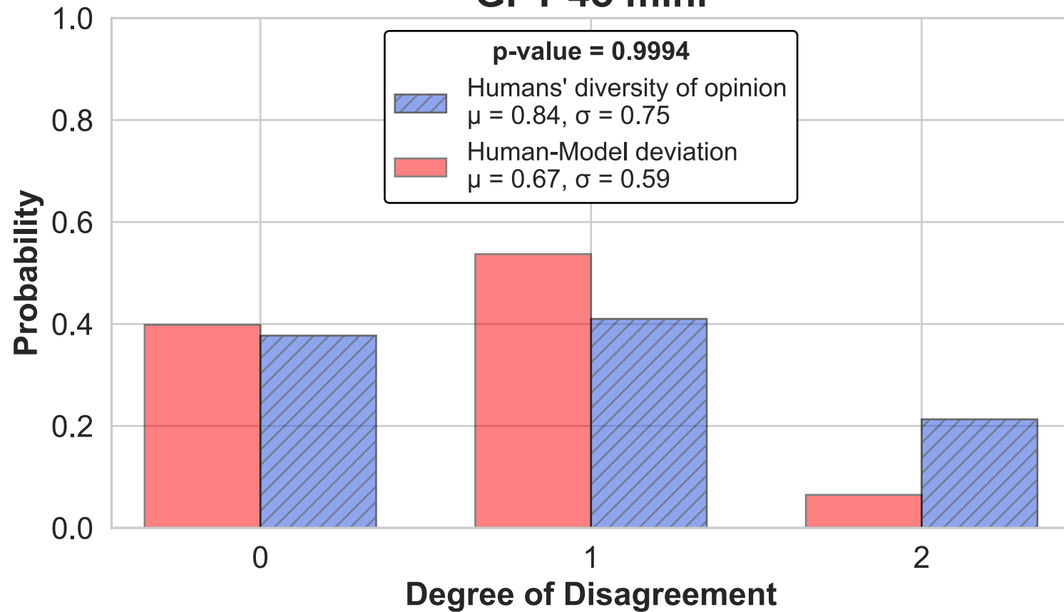
GPT-4o mini
