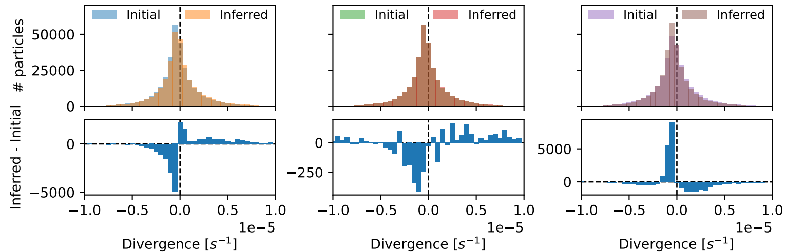
b) RK4 (FB)
