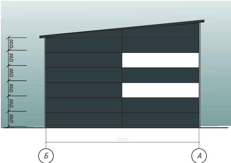
Фасад в осях Б-А
