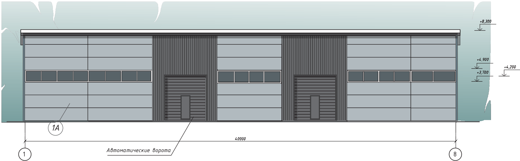
Фасад в осях 1-8 (вариант 2 )
