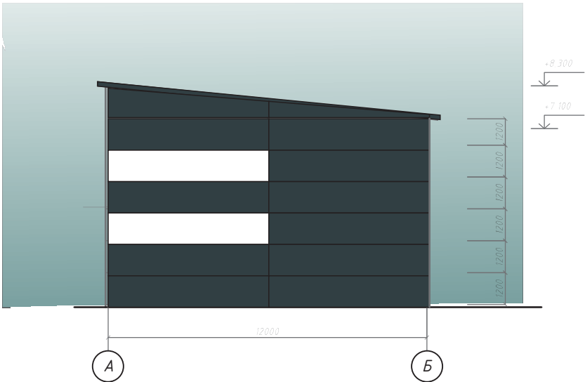
Фасад в осях А-Б
