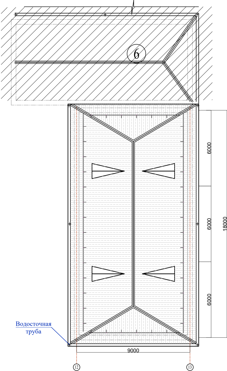
План кровля после реконструкция.
