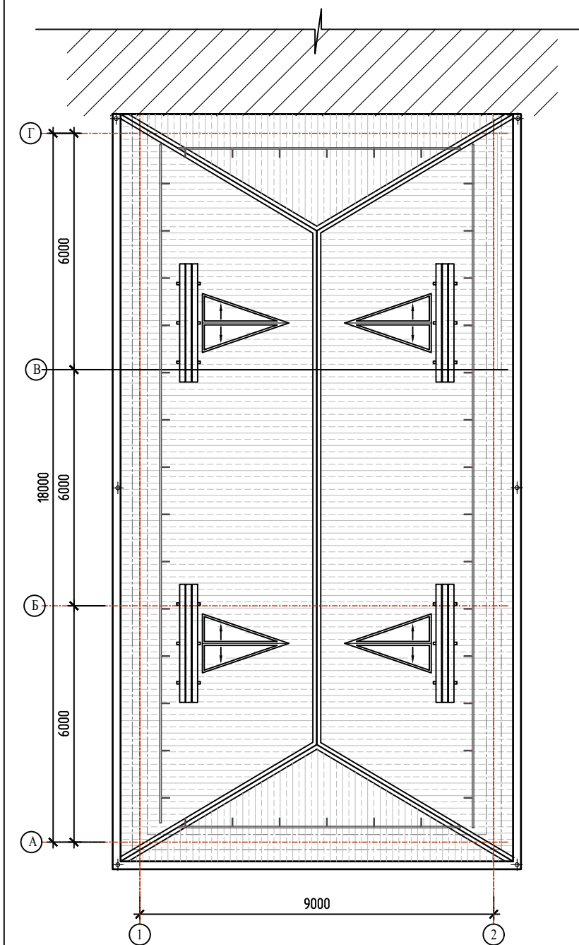
План кровля после реконструкция .
