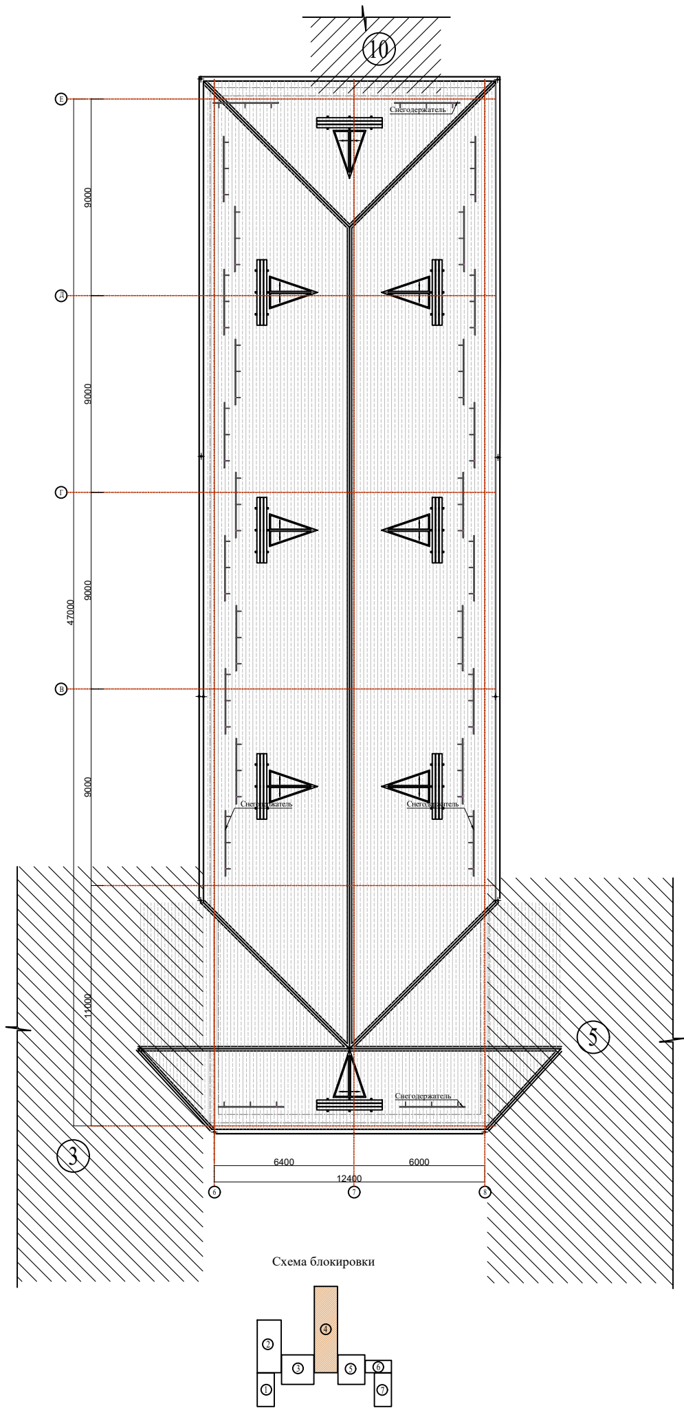
План кровля после реконструкция.
