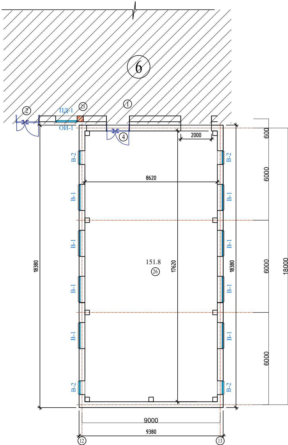
План стен 1-го этажа после реконструкция.
