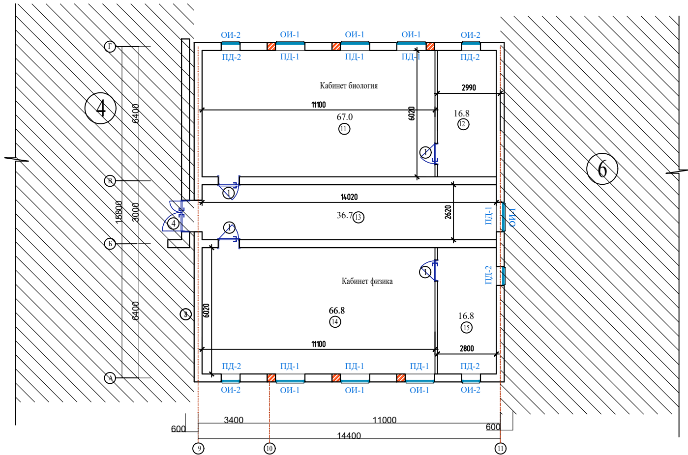
План стен 2-го этажа после реконструкция.
