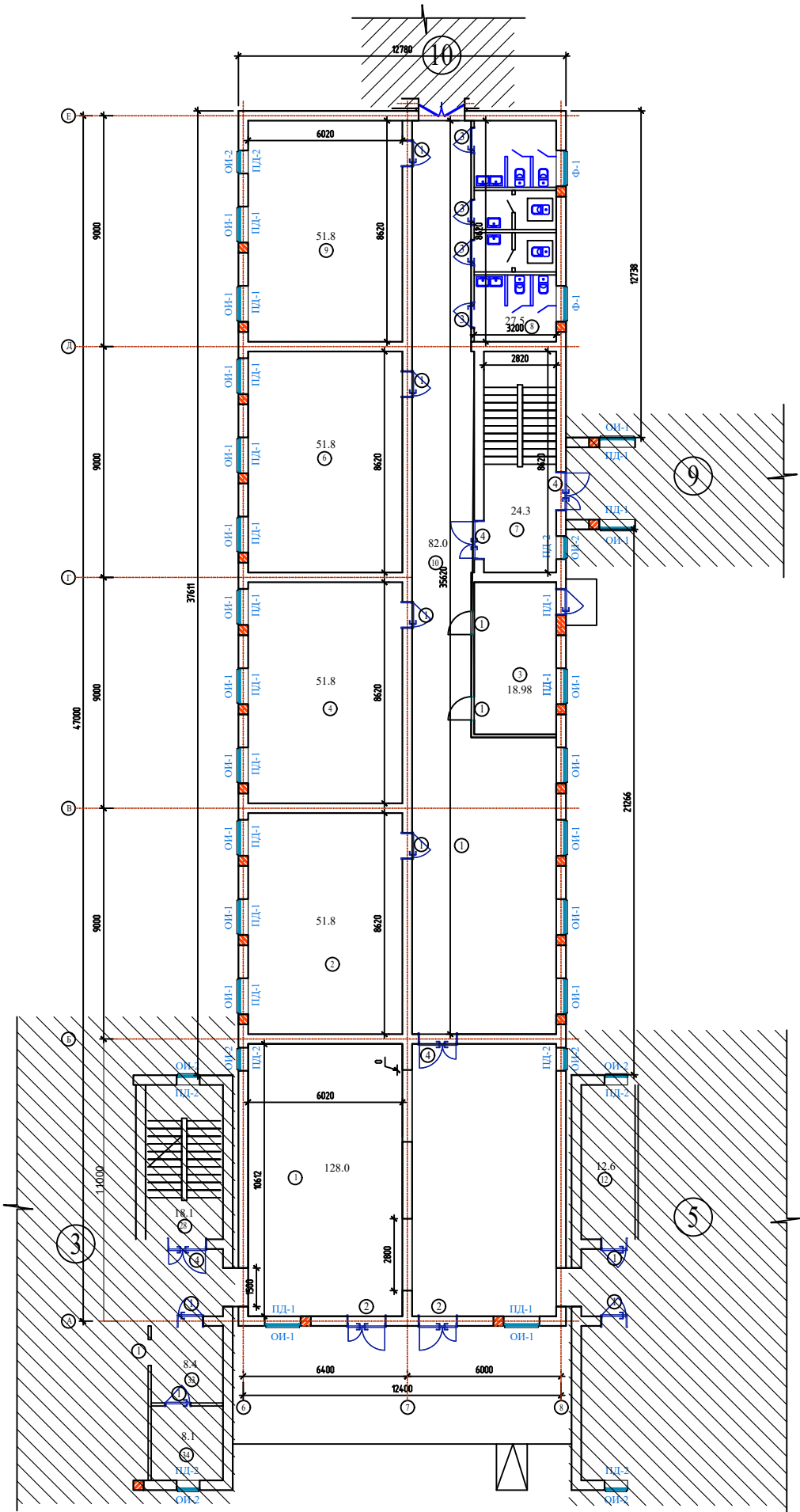
План стен 1-го этажа после реконструкция.
