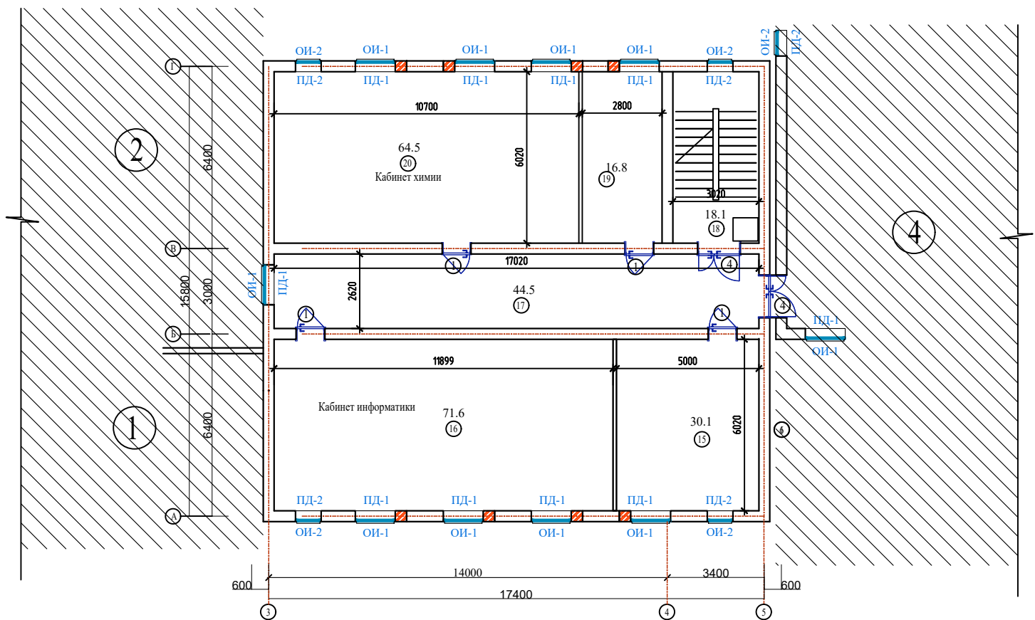
План стен 2-го этажа после реконструкция.
