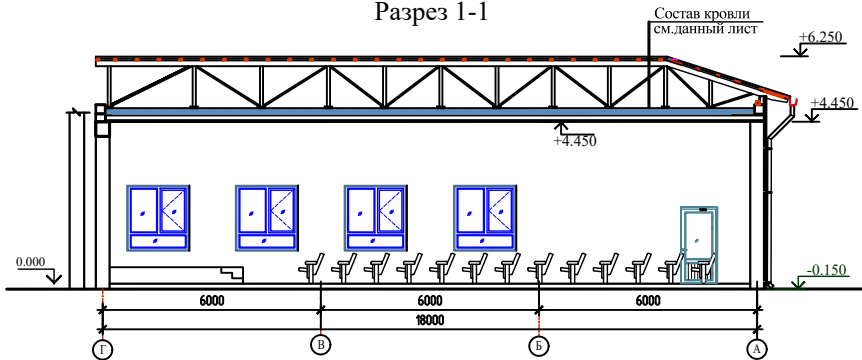
Разрез 1-1
