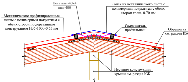
Узел-1
