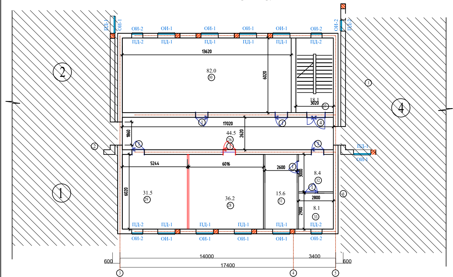
План стен 1-го этажа после реконструкция.
