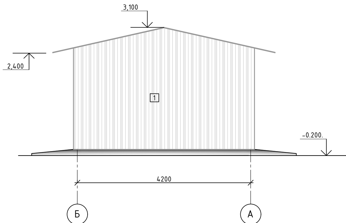
Фасад в осях Б-А М 1:50
