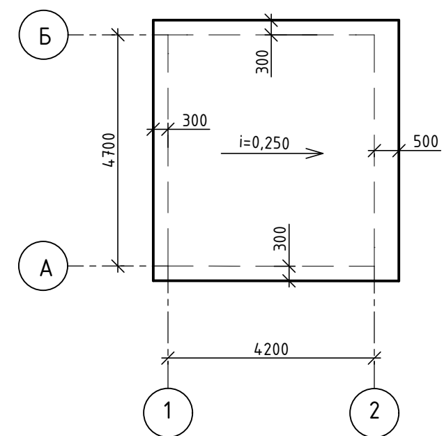
План кровли М 1:100
