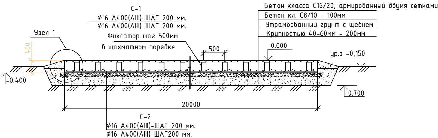
РАЗРЕЗ 1-1 М 1:50
