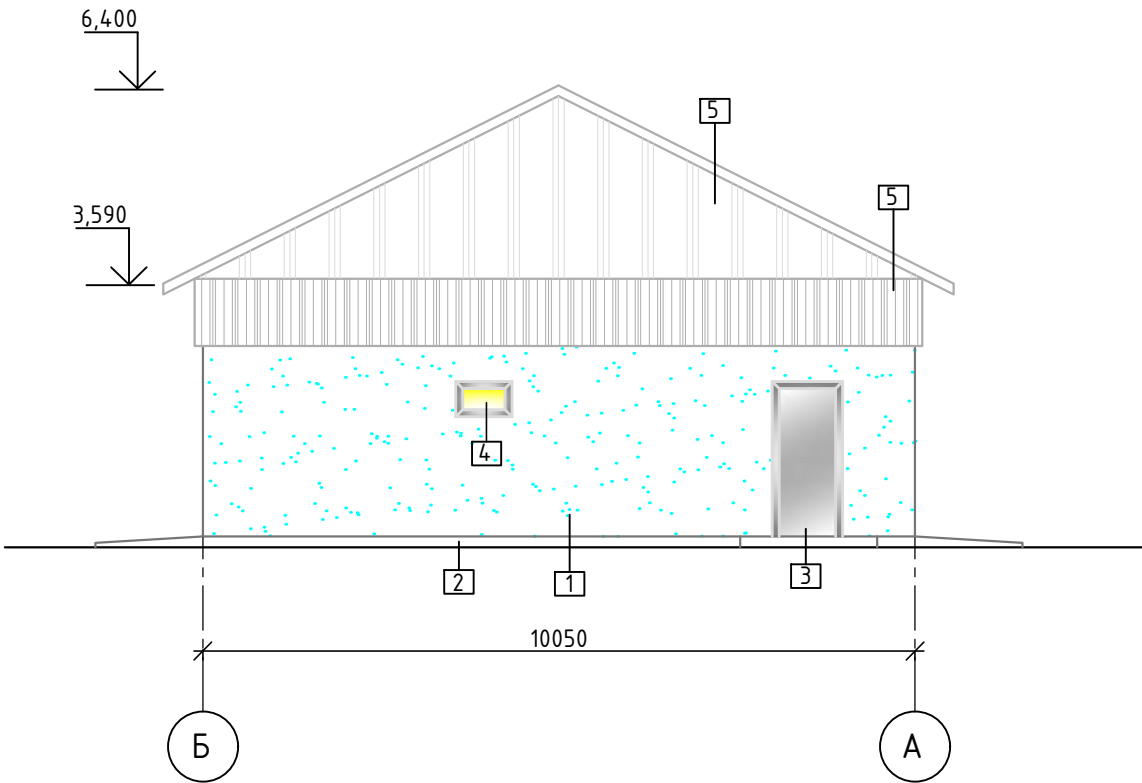
Фасад в осях Б-А М 1:100
