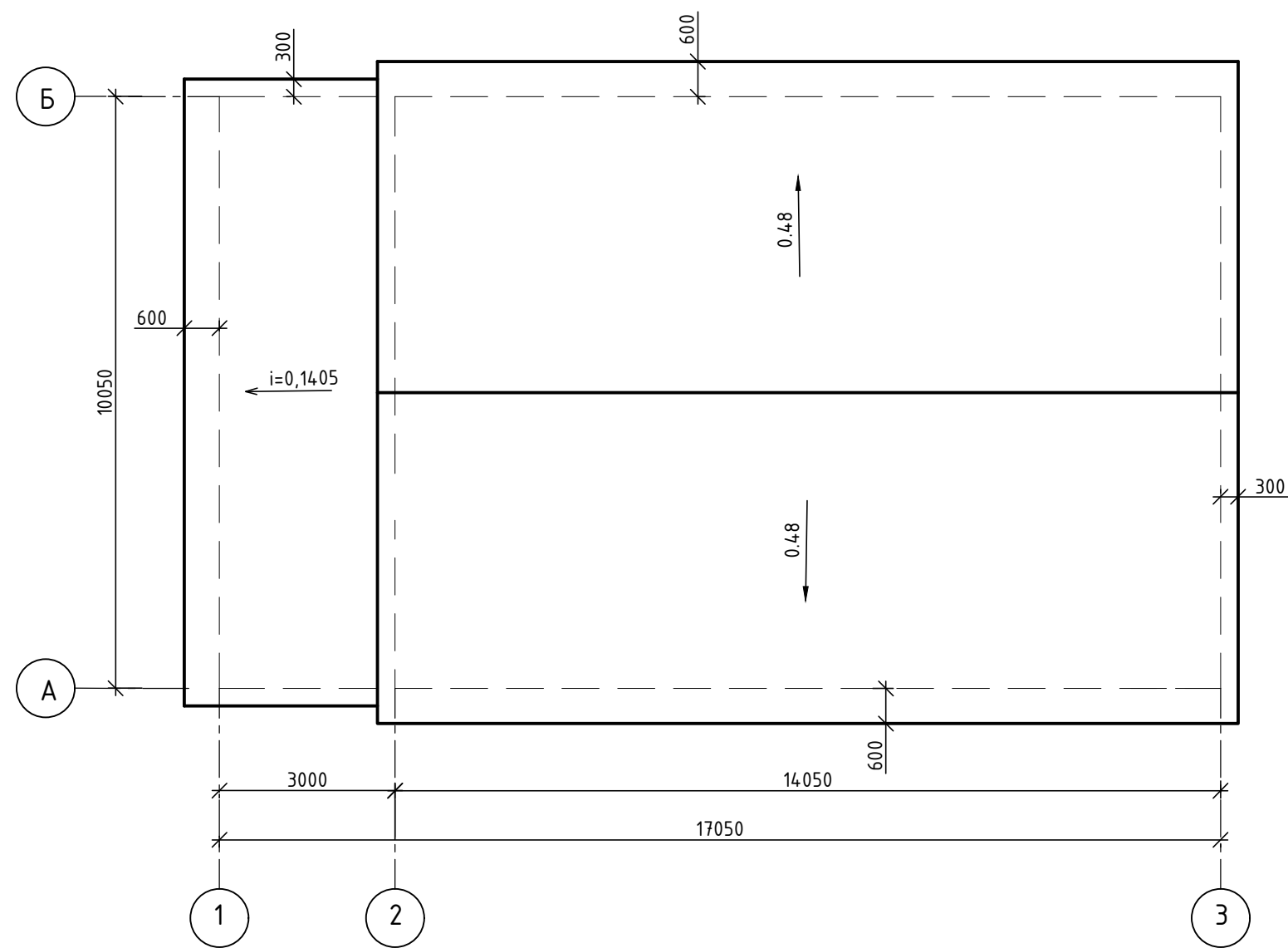
План кровли М 1:100
