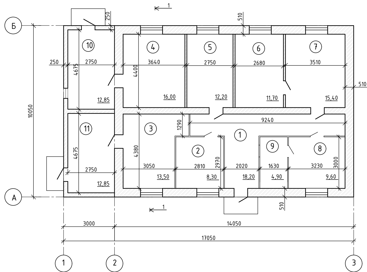
План на отм. 0.000 М 1:100
