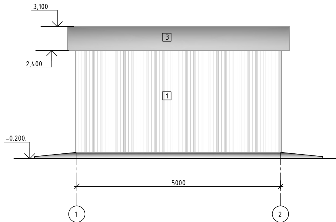
Фасад в осях 1-2, 2-1 М 1:50
