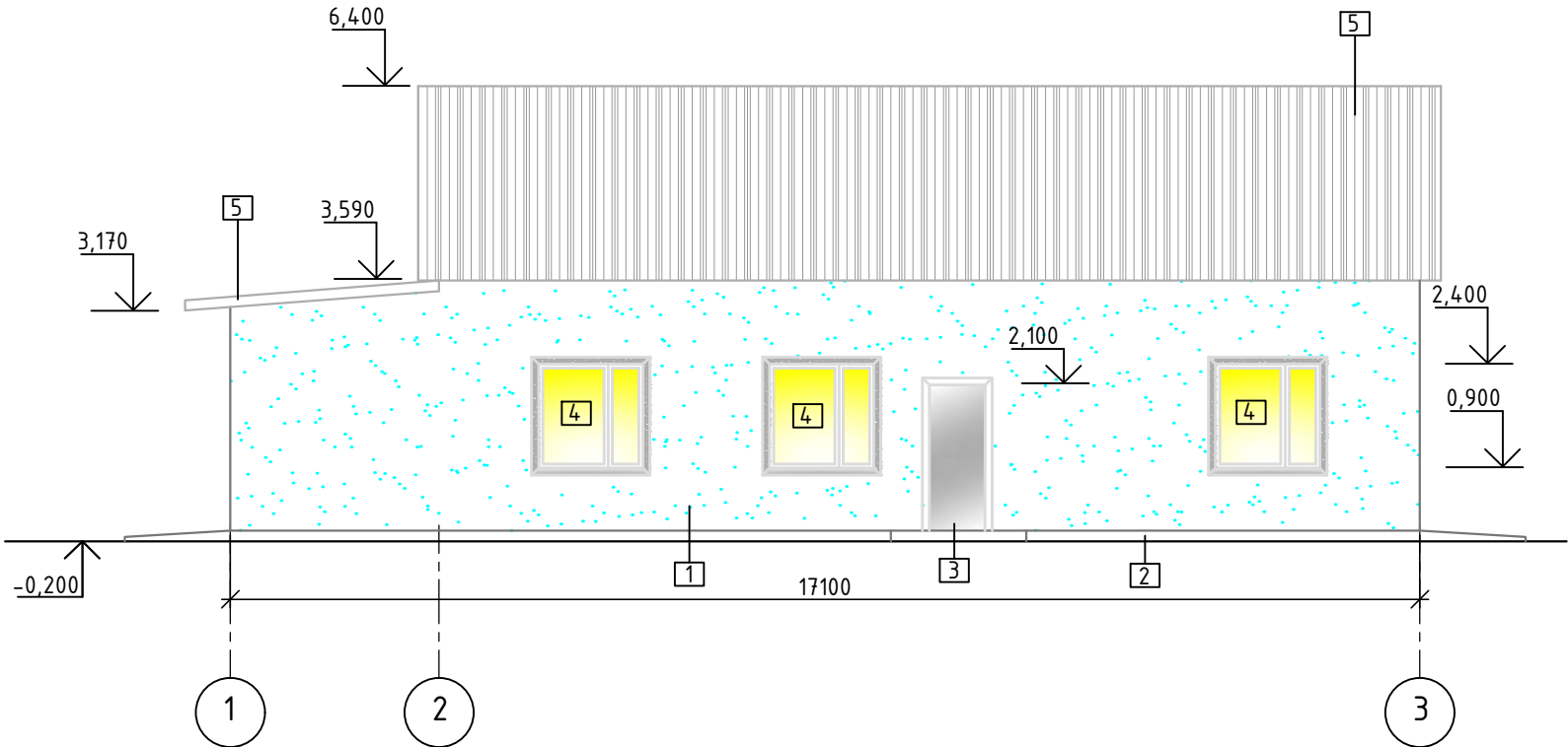
Фасад в осях 1-3 М 1:100
