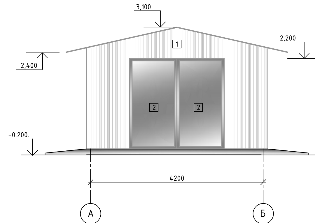
Фасад в осях А-Б М 1:50
