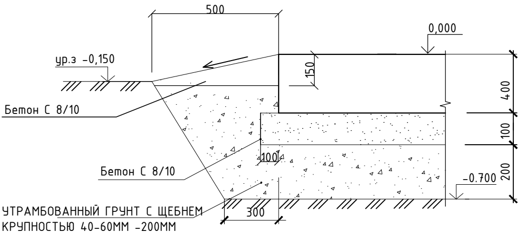
УЗЕЛ 1
