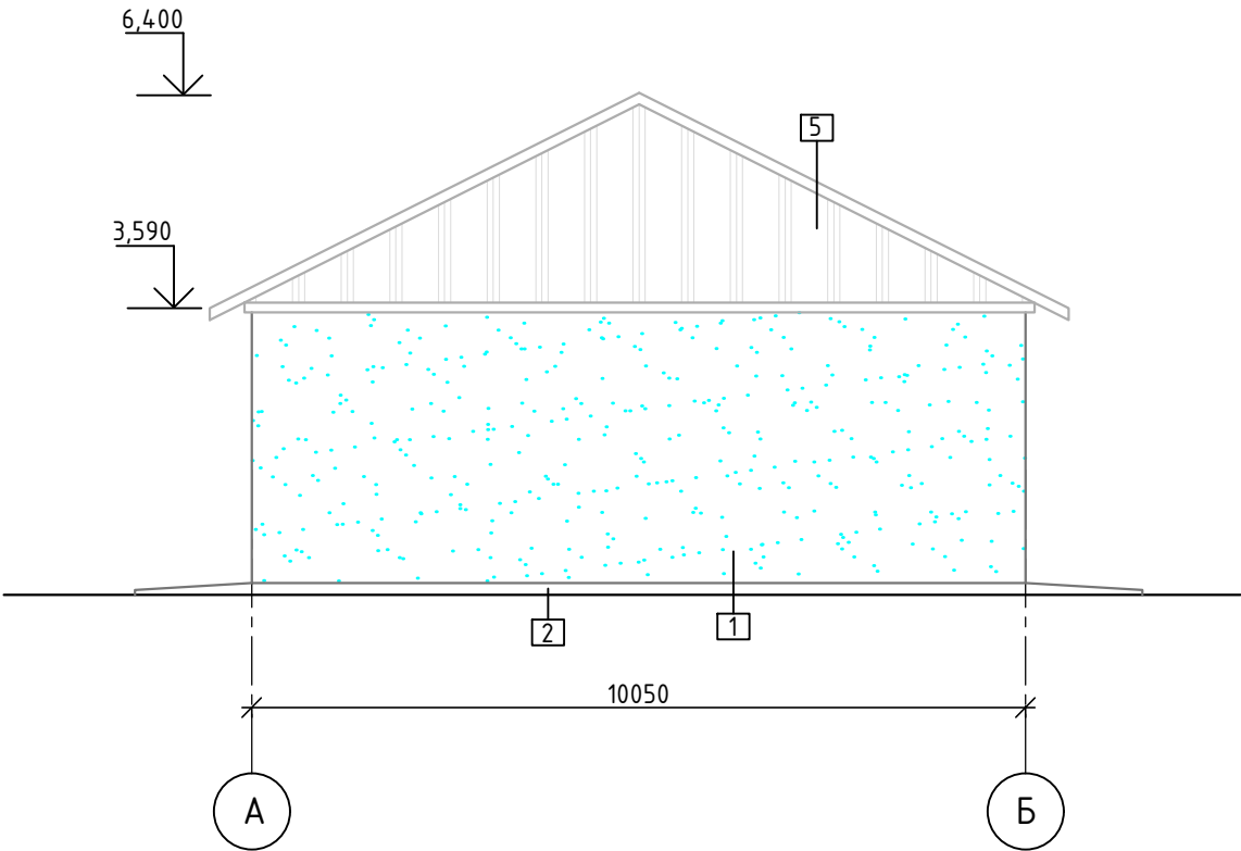
Фасад в осях А-Б М 1:100
