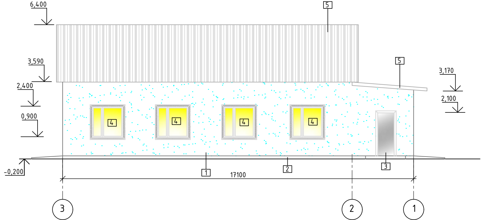
Фасад в осях 3-1 М 1:100
