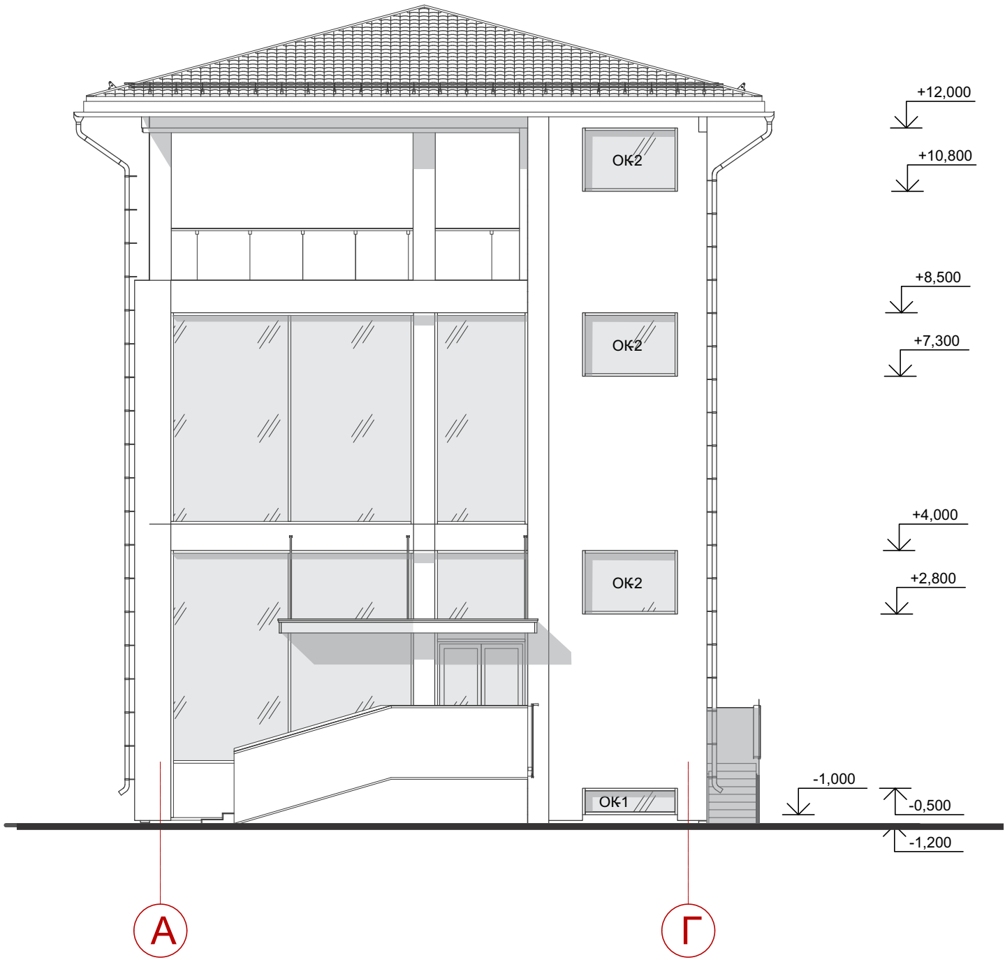
Фасад А-Г
