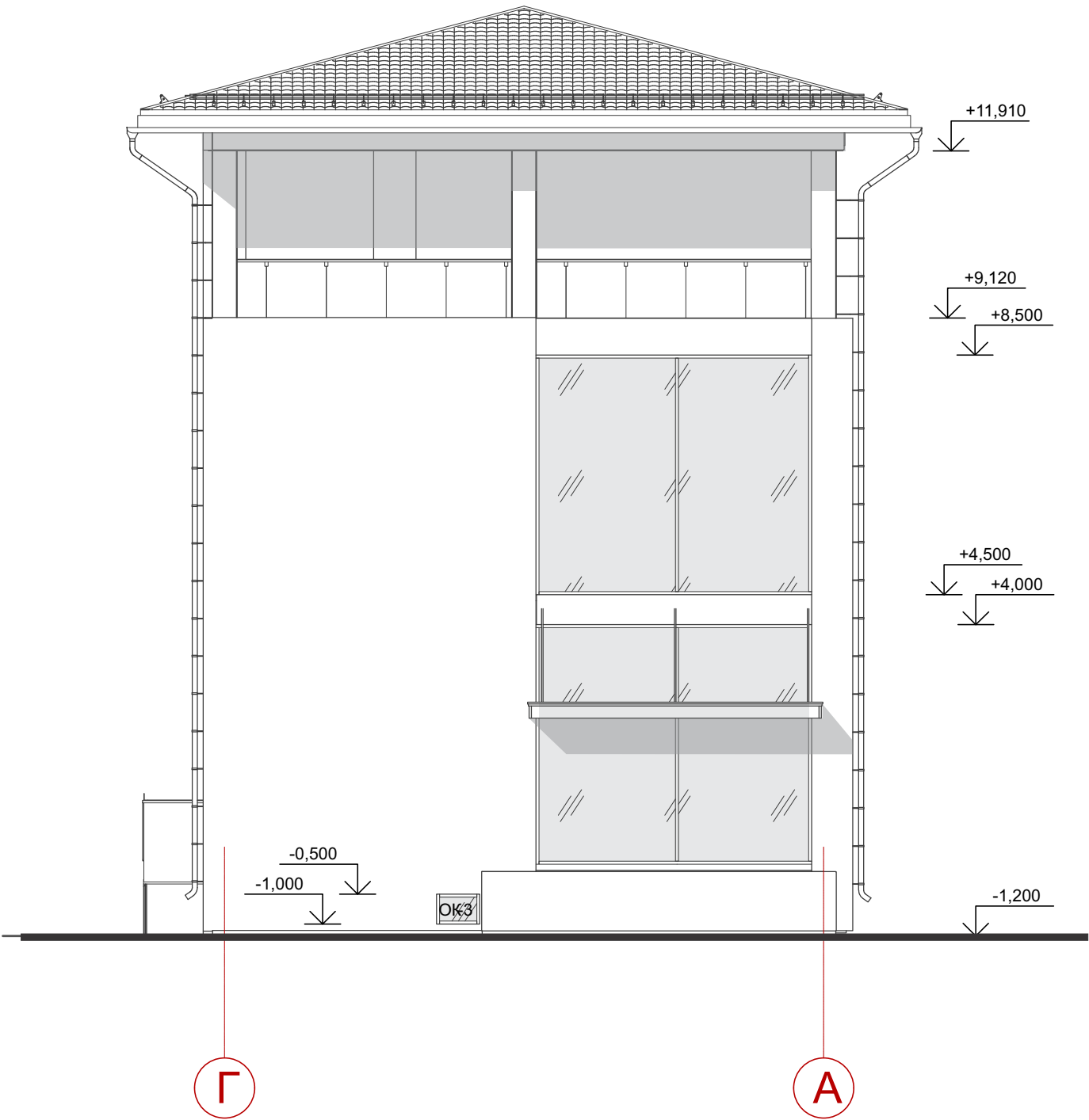
Фасад Г-А
